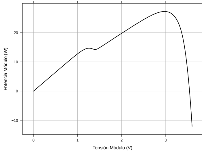
FIGURA 5.8: Curva potencia-tensión de la agrupación serie de la figura 5.4 cuando la célula C_4 presenta problemas de funcionamiento.
