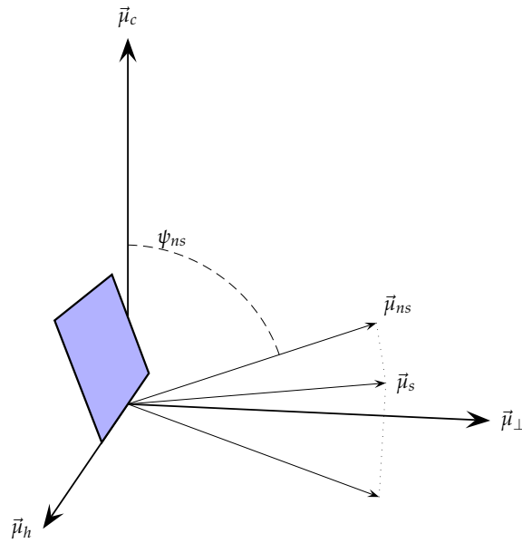
FIGURA 2.14: Vectores y ángulos en un SFCR de eje horizontal Norte-Sur.
