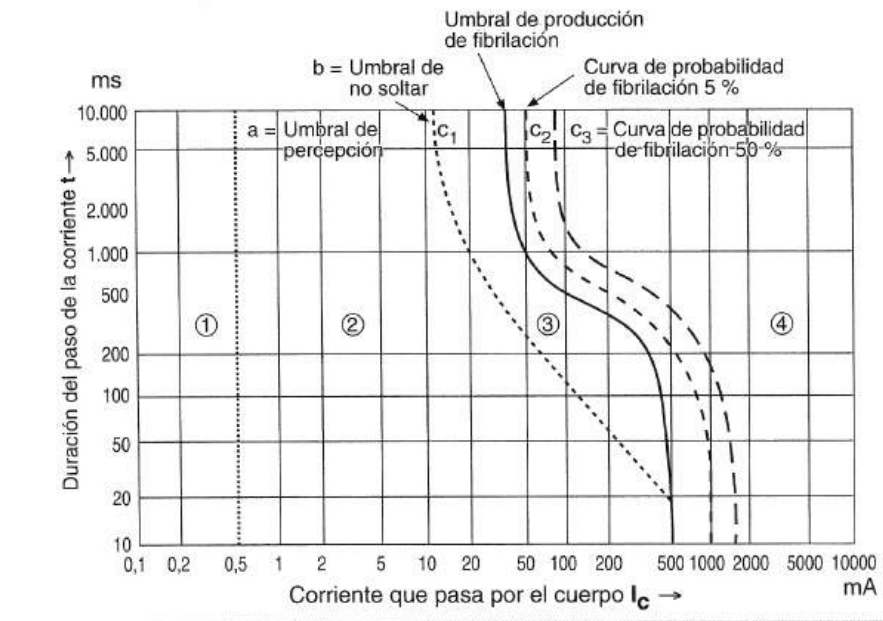
FIGURA 9.1: Efecto de la corriente que circula por el cuerpo humano según su intensidad y tiempo de duración [PG00b; PG00a].
