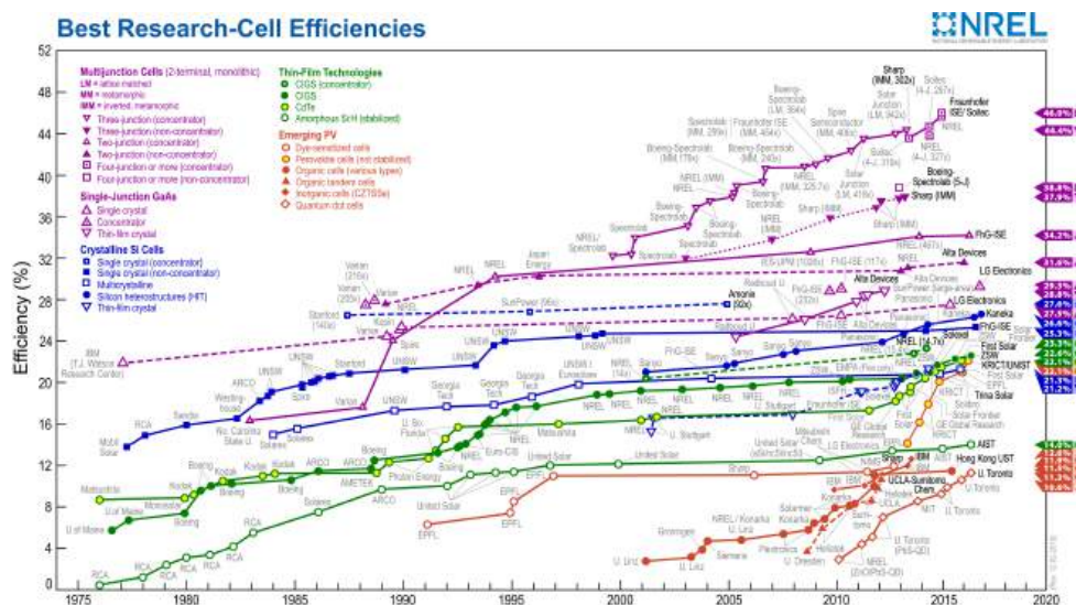
FIGURA 4.7: Evolución de la eficiencia de células según la tecnología (según el National Renewable Energy Laboratory (EEUU)).
