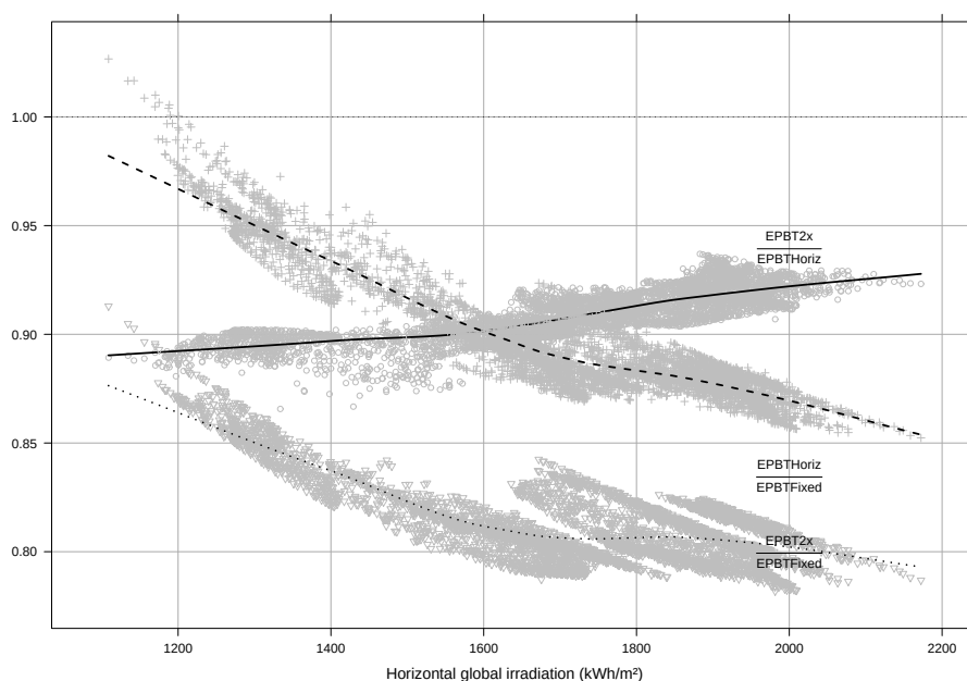
FIGURA 10.5: Comparación entre los EPBT de los diferentes sistemas frente a la radiación global en el plano horizontal en la región geográfica comprendida entre -10^\circ y 10^\circ de longitud, y 30^\circ a 45^\circ de latitud.
