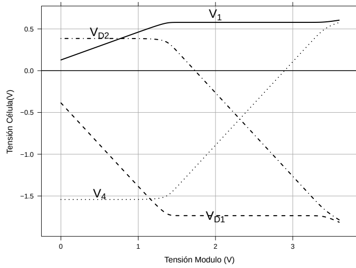
FIGURA 5.6: Tensiones en los elementos de la figura 5.4 para diferentes tensiones de la agrupación serie.
