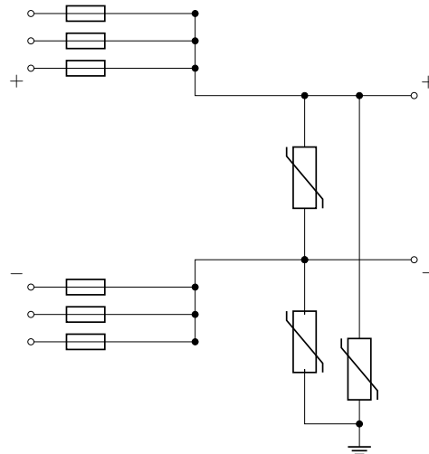
(B) Esquema eléctrico
