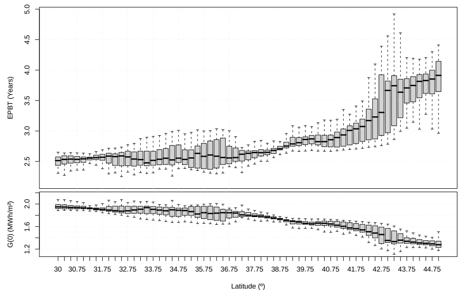
FIGURA 10.2: EPBT de un SFCR con seguimiento horizontal N-S para la región geográfica comprendida entre -10^{\circ} y 10^{\circ} de longitud, y 30^{\circ} a 45^{\circ} de latitud. La figura inferior muestra los valores anuales de radiación global en el plano horizontal como referencia.
