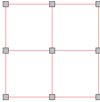
FIGURA 9.8: Esquema de un sistema de puesta a tierra compuesto por un conductor enterrado horizontalmente que interconecta picas verticales.
