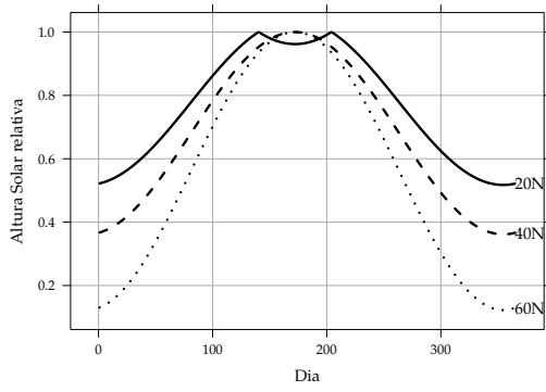
(A) Altura mediodía hemisferio Norte.
