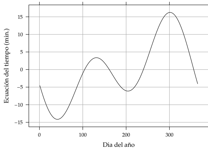
FIGURA 2.11: Ecuación del tiempo (minutos)
