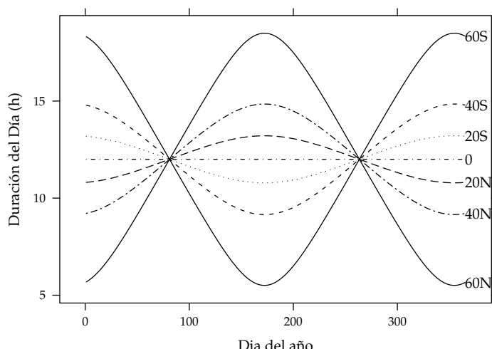
FIGURA 2.10: Duración del día en diferentes latitudes.
