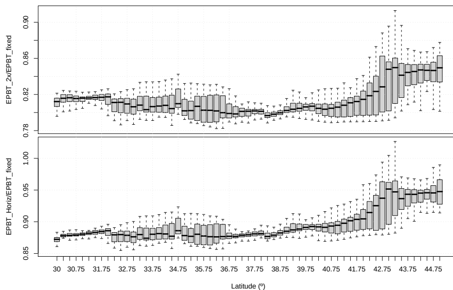
FIGURA 10.4: Comparación entre los valores de EPBT de un sistema a doble eje y un estático (figura superior), y un sistema de seguimiento de eje horizontal N-S con un estático (figura inferior) para la región geográfica comprendida entre -10^\circ y 10^\circ de longitud, y 30^\circ a 45^\circ de latitud.
