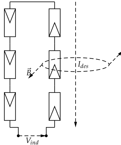
FIGURA 9.10: Inducción sobre un generador.
