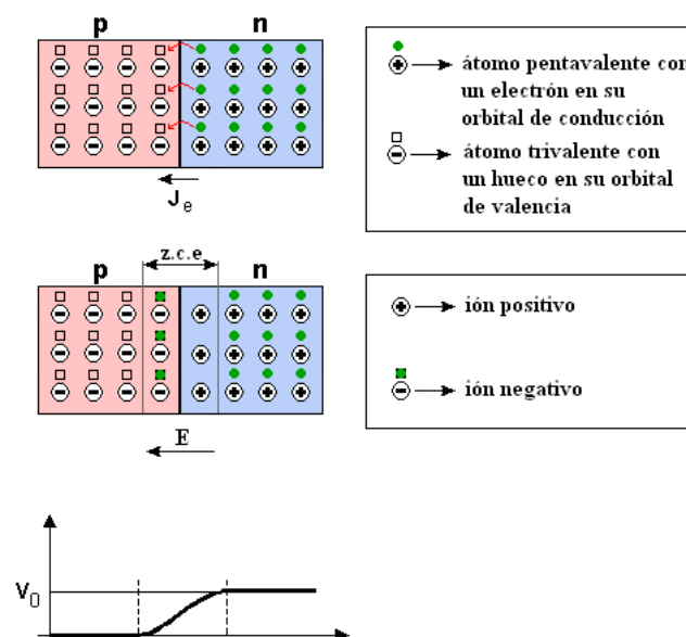
FIGURA 4.2: Unión p-n..
