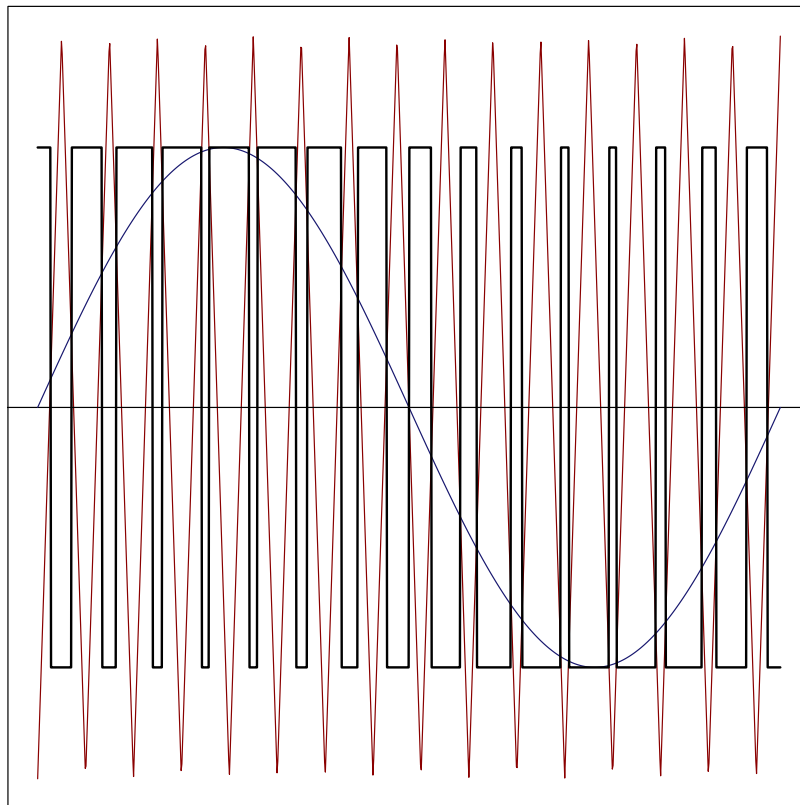
FIGURA 6.4: Onda SPWM monofásica bipolar.
