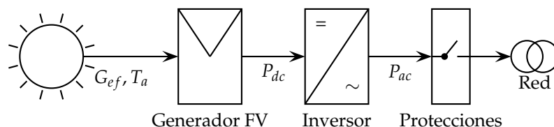
FIGURA 6.1: Esquema de un SFCR.
