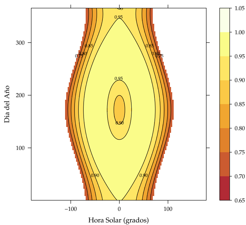
FIGURA 2.18: Coseno del ángulo de incidencia de un seguidor acimutal a lo largo del día y año para un sitio con latitud 40^\circ\text{N} .
