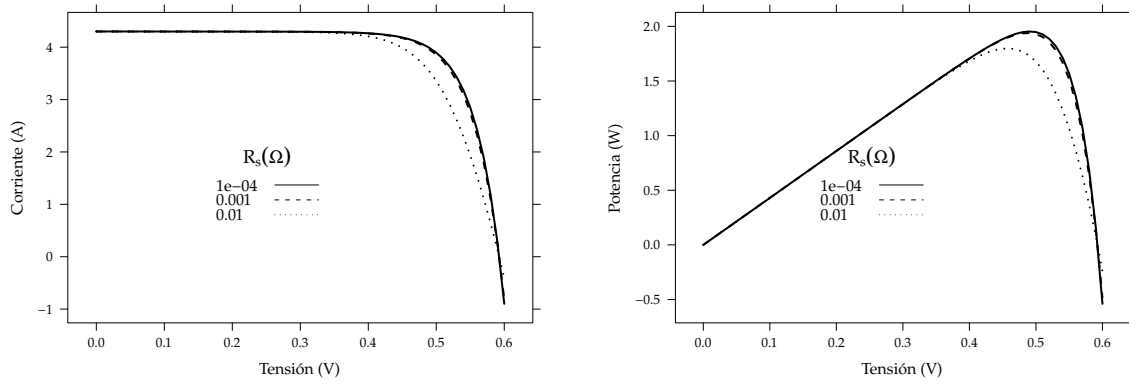
(A) Curva I-V.
