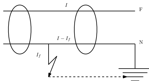
FIGURA 9.14: Funcionamiento de un interruptor diferencial.
