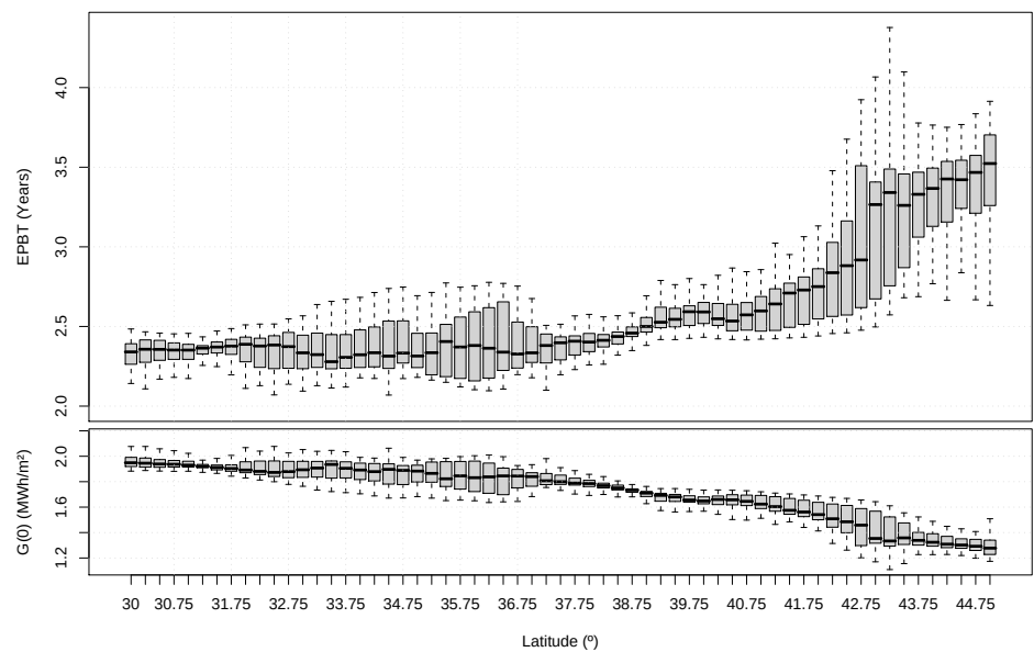
FIGURA 10.1: EPBT de un SFCR con seguimiento a doble eje para la región geográfica comprendida entre -10^{\circ} y 10^{\circ} de longitud, y 30^{\circ} a 45^{\circ} de latitud. La figura inferior muestra los valores anuales de radiación global en el plano horizontal como referencia.
