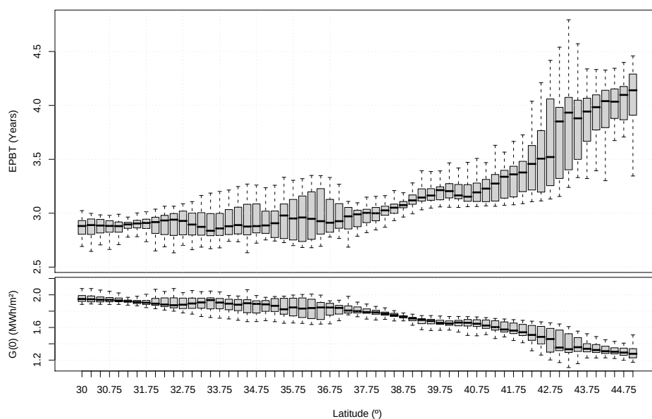
FIGURA 10.3: EPBT de un SFCR estático para la región geográfica comprendida entre -10^\circ y 10^\circ de longitud, y 30^\circ a 45^\circ de latitud. La figura inferior muestra los valores anuales de radiación global en el plano horizontal como referencia.
