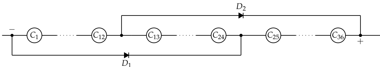
FIGURA 5.9: Configuración típica de conexión de diodos de paso en una serie de 36 células.
