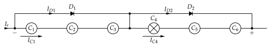
FIGURA 5.4: Colocación de diodo de paso para evitar el fenómeno de punto caliente.
