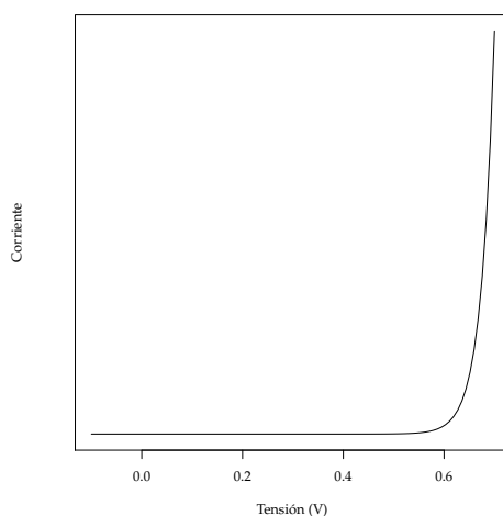
(A) Característica corriente-tensión de un diodo según la ecuación 4.1.
