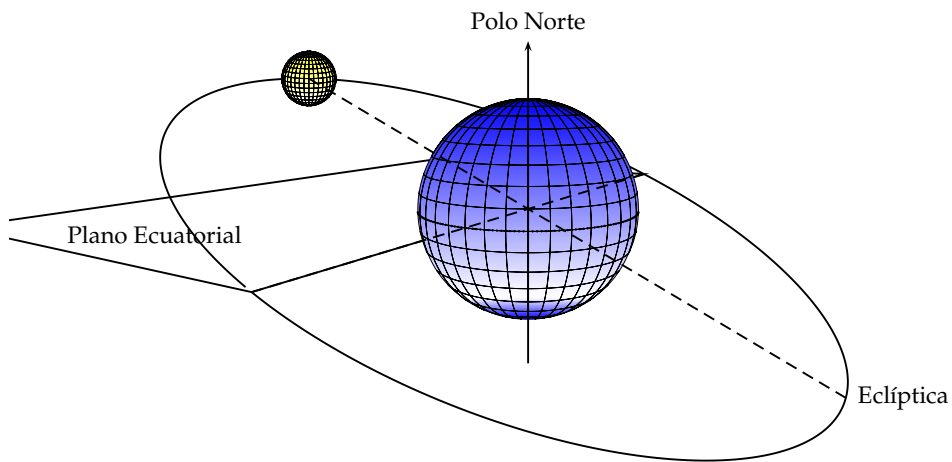
FIGURA 2.3: Sistema geocéntrico según el cual el Sol parece girar alrededor de la Tierra.
