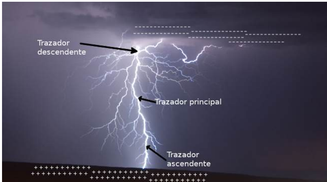
FIGURA 9.9: Formación de un rayo eléctrico (imagen elaborada a partir de la fotografía disponible en http://commons.wikimedia.org/wiki/File:DC16_Lightning.jpg ).
