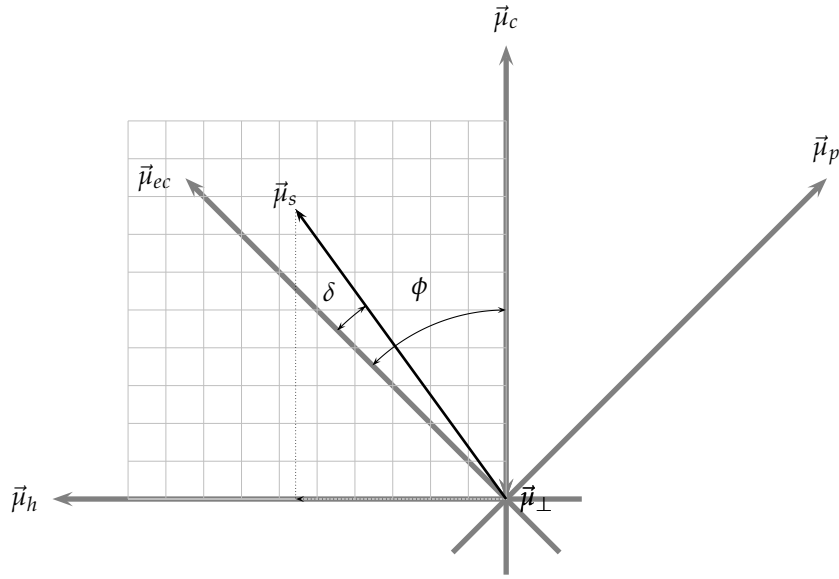
FIGURA 2.7: Relación entre los sistemas de coordenadas terrestre y local (particularizado para el hemisferio Norte).
