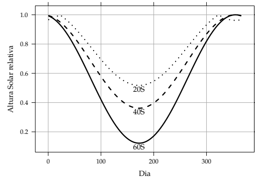
(B) Altura mediodía hemisferio Sur.
