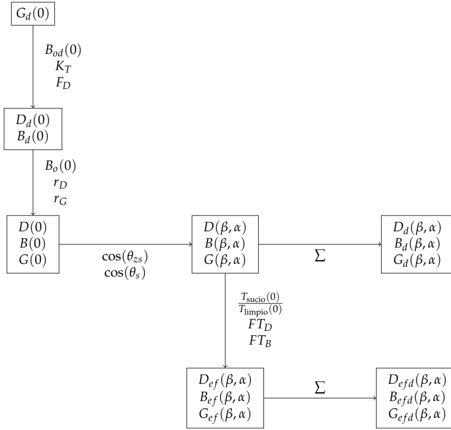
FIGURA 3.3: Procedimiento de cálculo.
