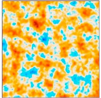
Planck
