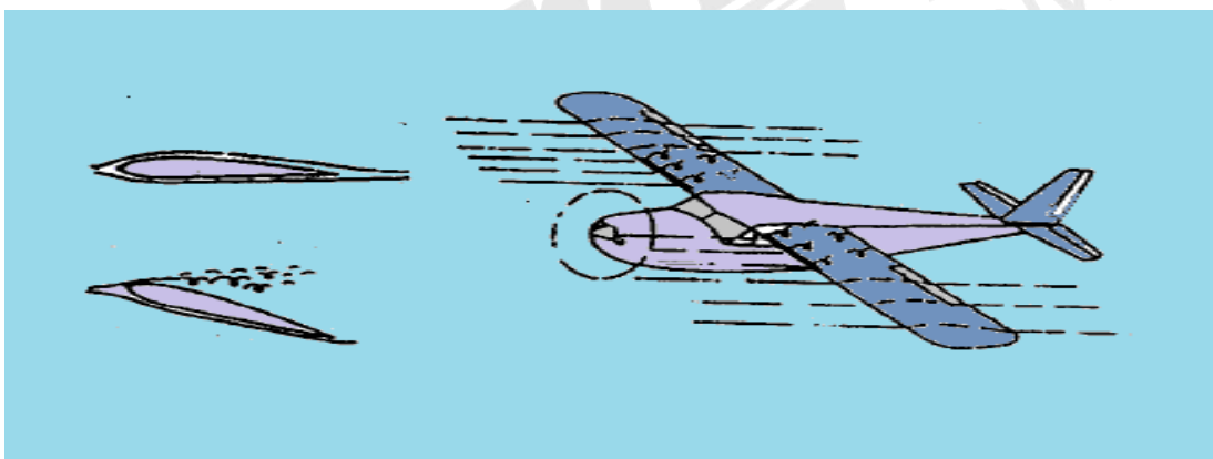
Figura 13-21 Spoileres fixos.
