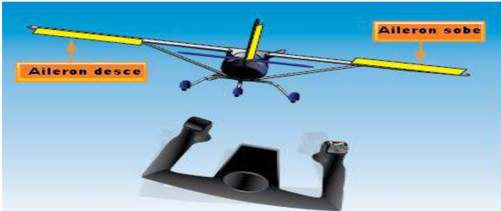
Figura 13-19 Sistema de controle do aileron.
