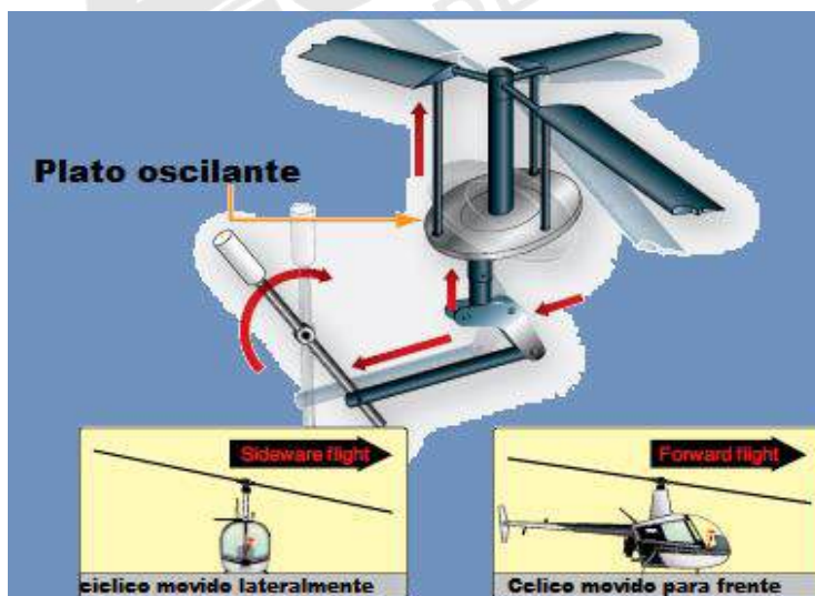
Figura 13-44 Mecanismo de controle do passo cíclico.
