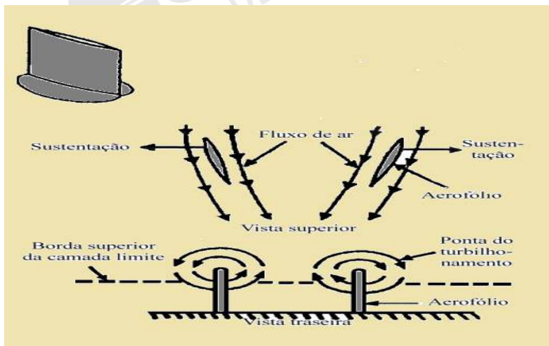
Figura 13-56 Gerador de turbilhonamento na asa.
