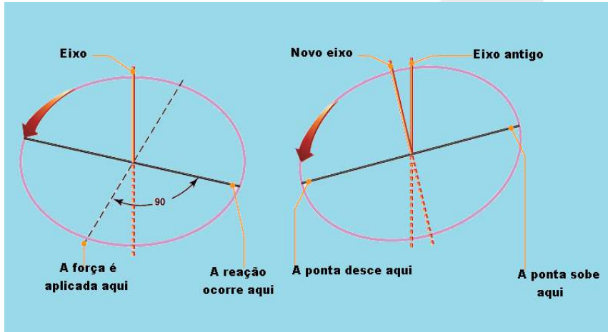
Fonte: FAA - Mechanic Training Handbook-Airframe Figura 13-34 Princípio da precessão giroscópica.
