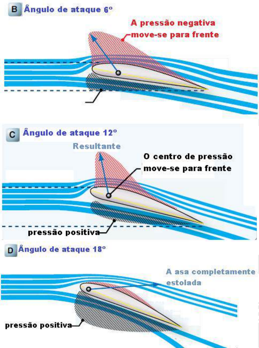
Figura 13-5 Efeito do aumento do ângulo de ataque.
