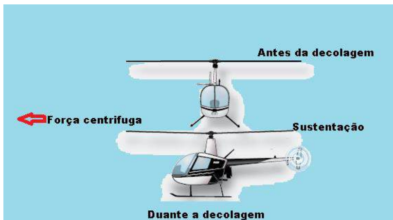
Fonte: FAA - Mechanic Training Handbook-Airframe Figura 13-41 Cone nas pás.
