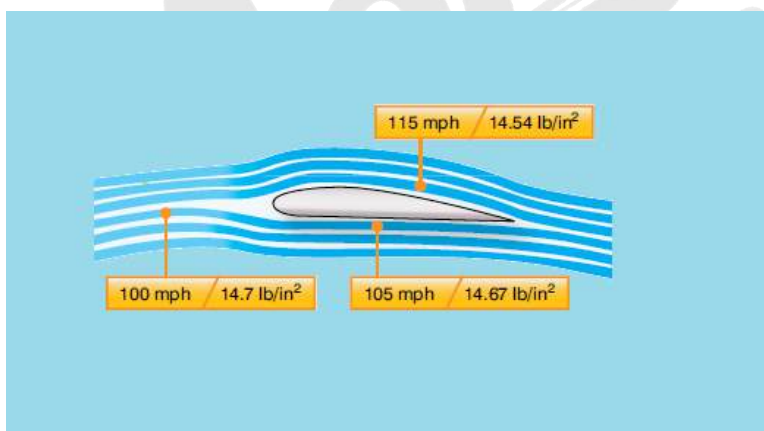
Figura 13-3 Fluxo de ar sobre a seção de uma asa.
