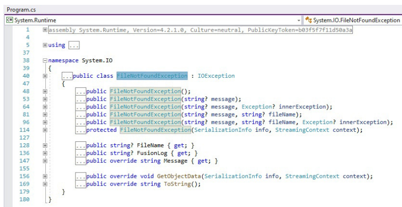
Figura 8.2: Inspeccionando os membros da classe FileNotFoundException
