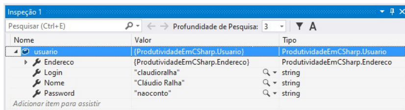
Figura 13.5: Inspecionando as propriedades do objeto usuario
