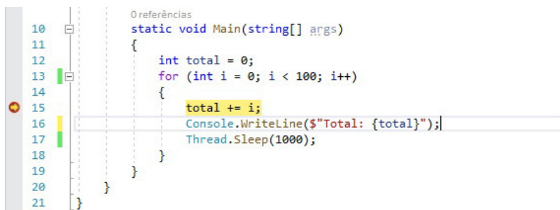
Figura 12.21: Empregando o recurso Editar e Continuar
