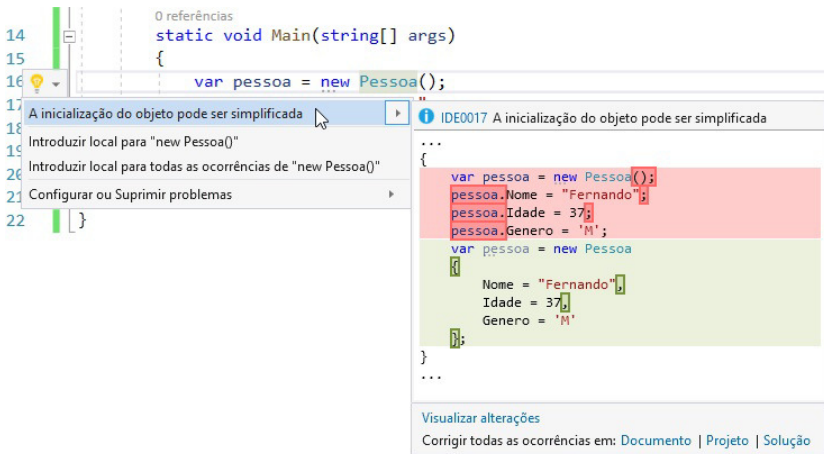
Figura 11.28: Simplificando a inicialização de um objeto
