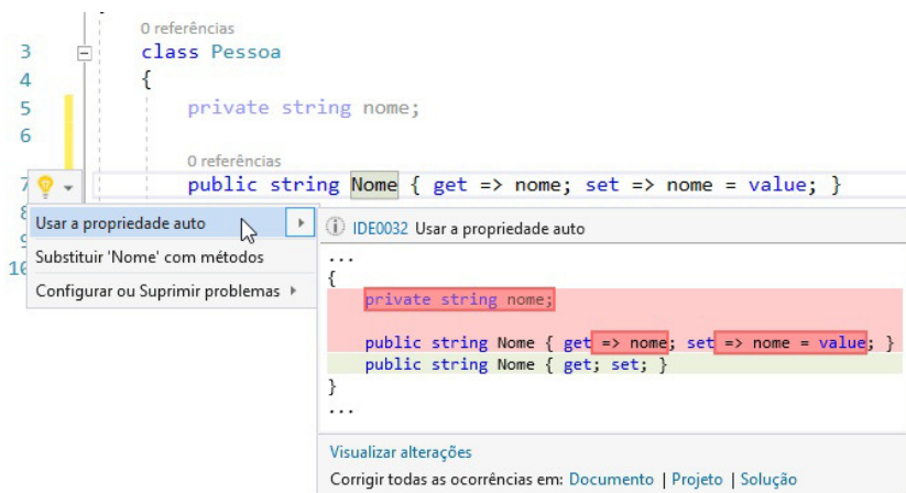
Figura 11.13: Convertendo uma propriedade em uma propriedade autoimplementada
