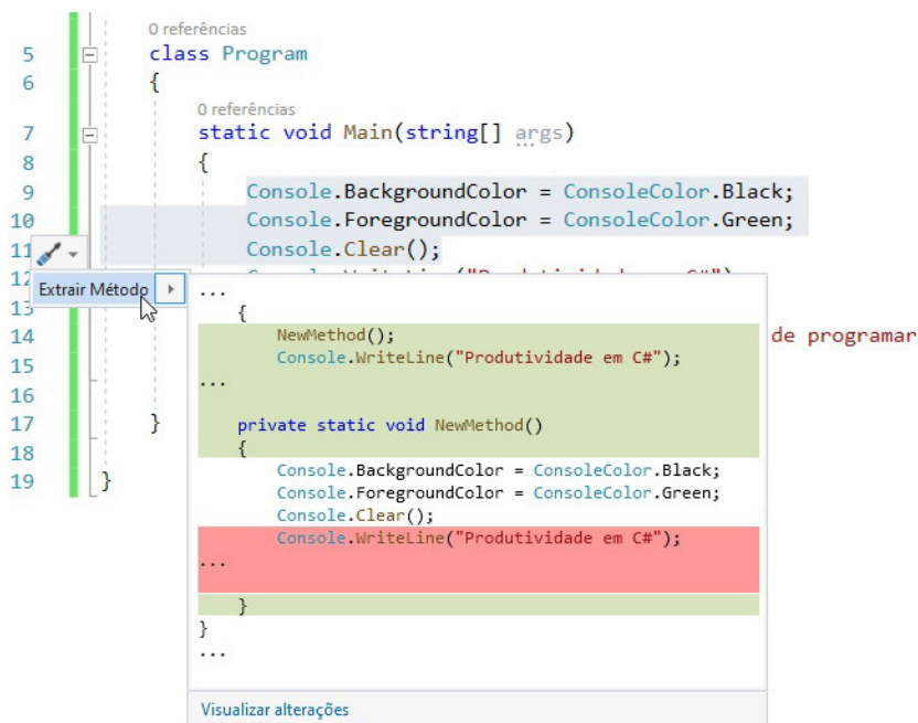
Figura 11.19: Aplicando a ação rápida de extração de método
