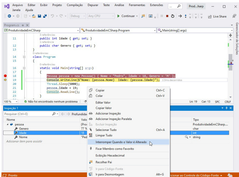
Figura 12.11: Definindo um ponto de interrupção de dados
