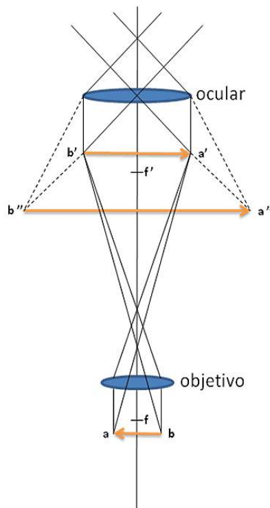
Figura 5. Diagrama do funcionamento de um microscópio óptico composto. ab : objecto colocada diante do foco ( f ); a'b' : imagem real invertida formada pela objectiva; a''b'' : imagem virtual ampliada formada pela ocular que será visualizada pelo observador. Adaptado de Langueron M. 1949.
