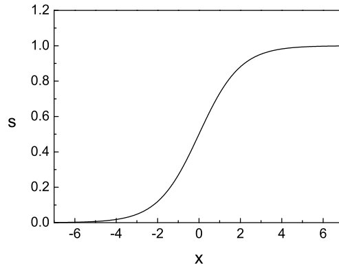
Fig. 11.10. Sigmoid function.
