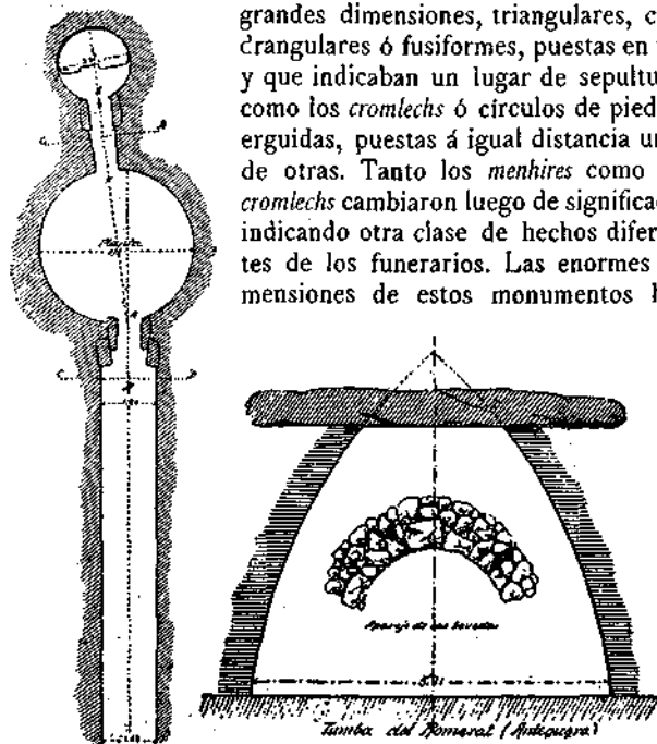
Fig. 9. — Planta y corte de la tumba del Romeral.
