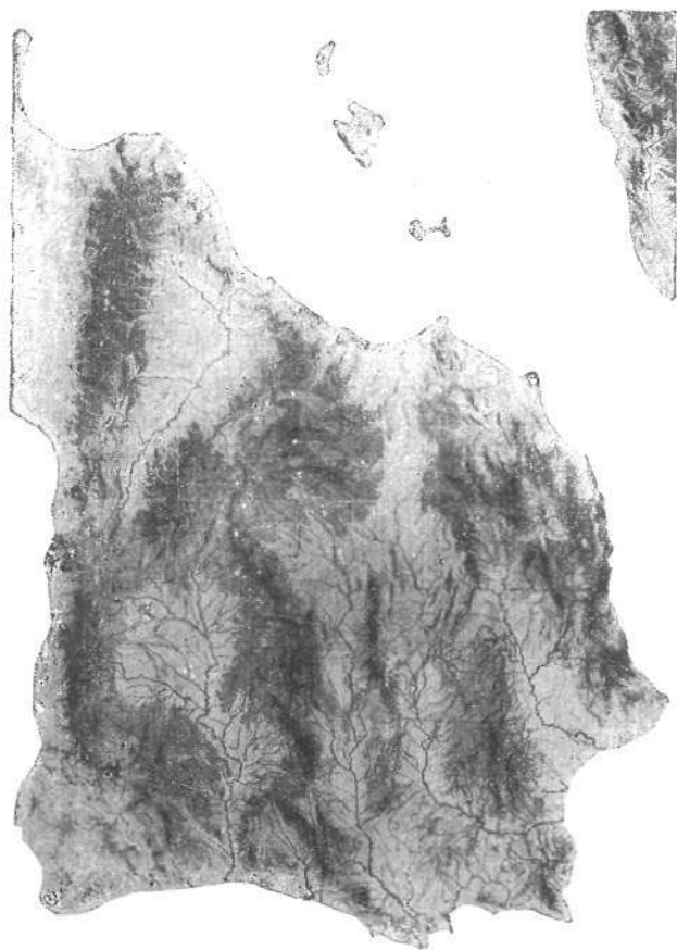
Fig 1. — Mapa hipsométrico, ó de alturas, de la Peninsula, según los datos de Kiepert. (Los trozos más oscuros son los más altos.)
