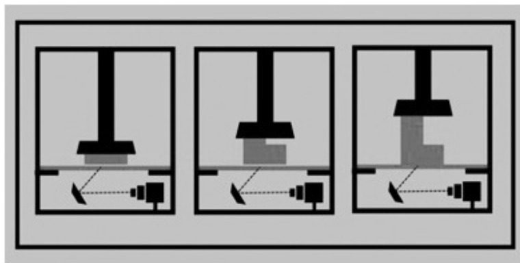
Figura 2.6 – Técnica DLP.
