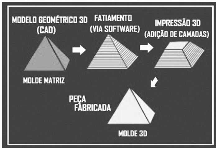
Figura 2.4 – Processo de Camada por Camada (Fatiamento).
