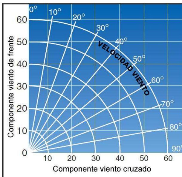
Figura 8-19. Gráfico de componente de viento cruzado.
