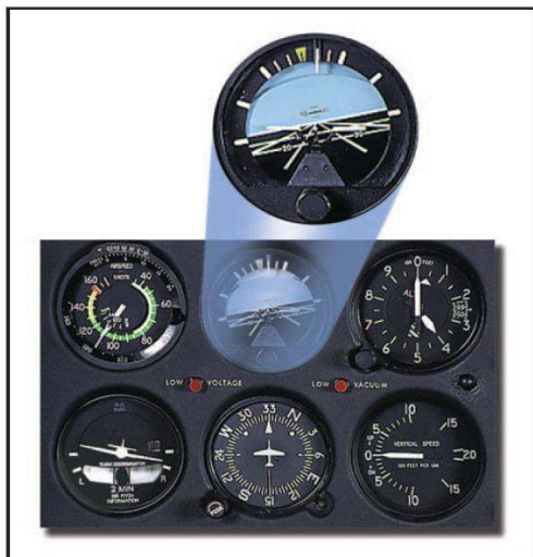
Figura 14-12. Viraje nivelado.
