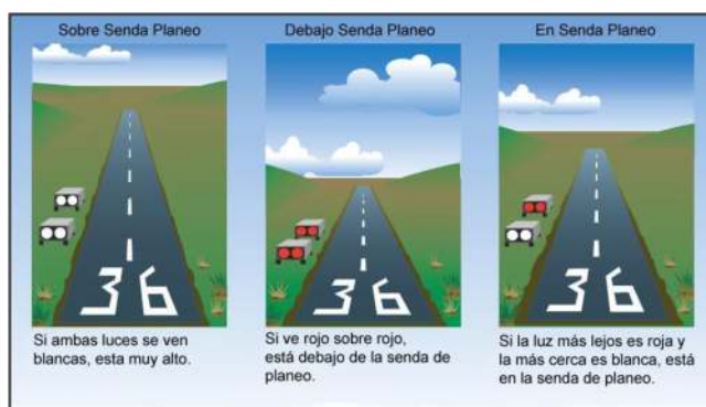
Figura 10-5. VASI.
