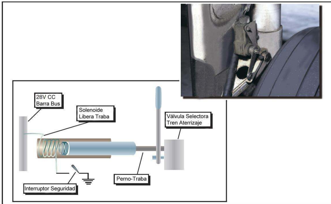
Figura 11-8. Interruptor de seguridad del tren de aterrizaje.
