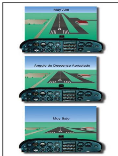
Figura 8-11. Cambio en la forma de la pista si la aproximación es más baja o más alta.
