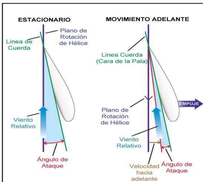
Figura 11-3. Ángulo de pala de la hélice.
