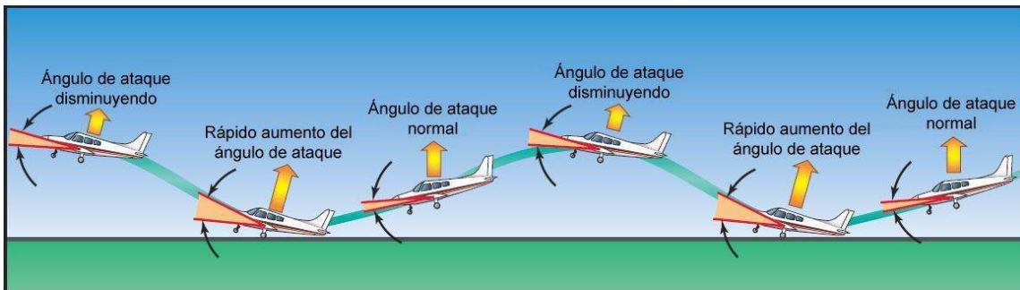
Figura 8-36. Delfineo.
