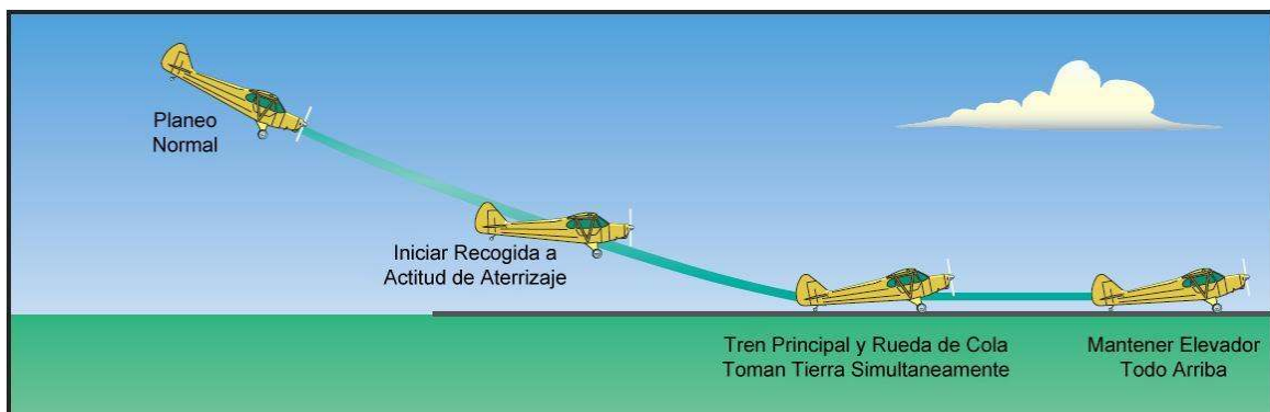
Figura 13-1. Aterrizaje de un avión con rueda de cola.
