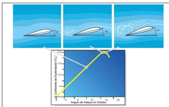
Figura 4-2. Ángulo de ataque crítico y pérdida.
