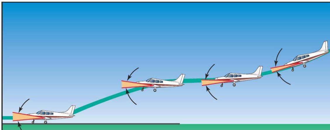
Figura 8-32. Recogida o Flare muy alto.
