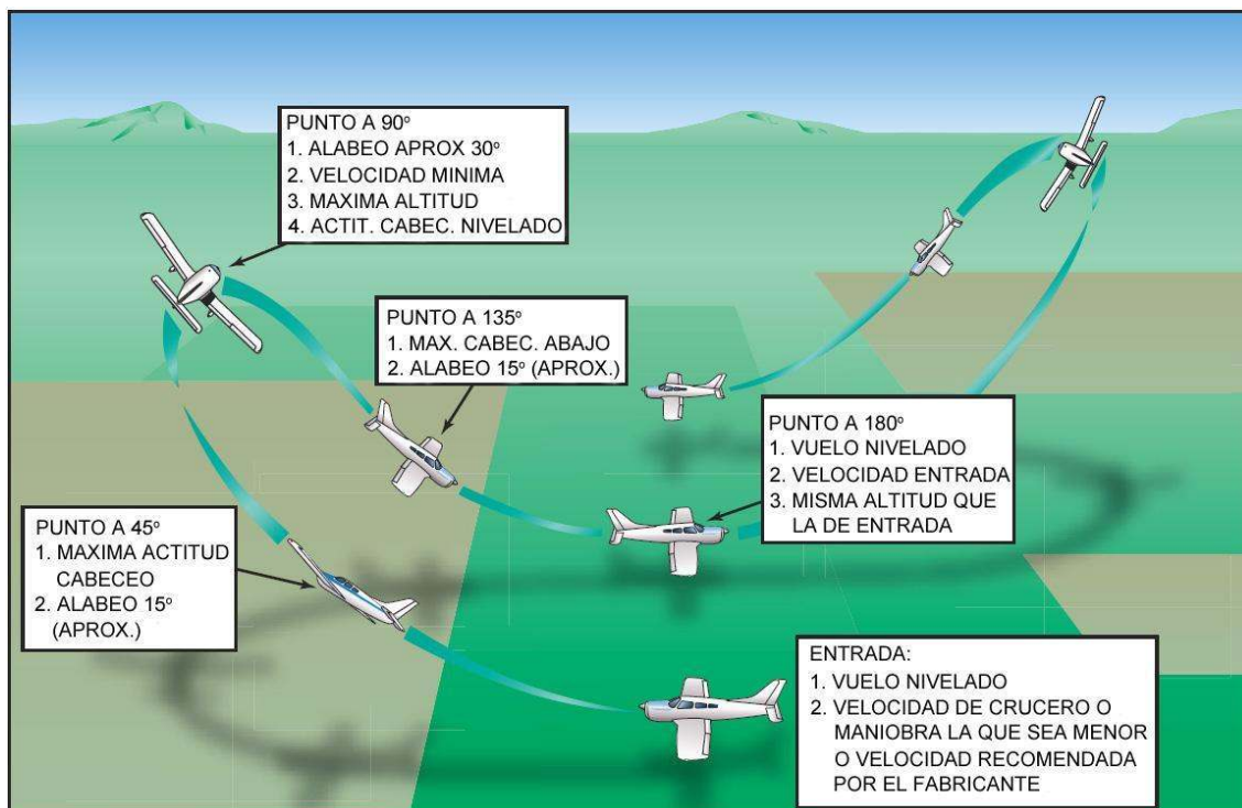
Figura 9-5. Ocho perezoso.
