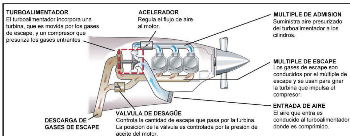
Figura 11-5. Sistema de turboalimentación.
