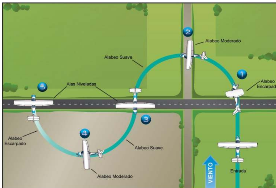
Figura 6-5. “S” sobre camino.
