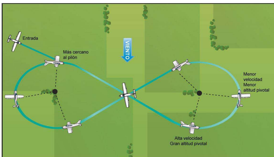
Figura 6-10. Ocho sobre pilones.
