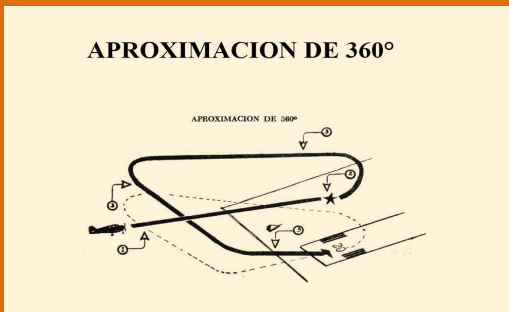
Figura 8-28. Aproximación sin potencia de 360°.
