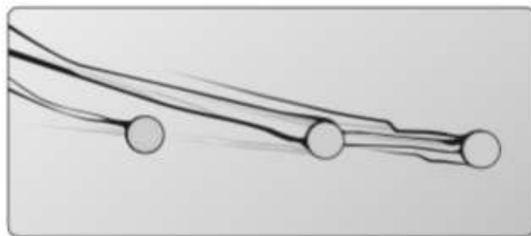
Figura 2-10. Ejemplo de cabezas de remaches donde se formó una película de óxido negro debido a que el remache se afloja en su agujero.
