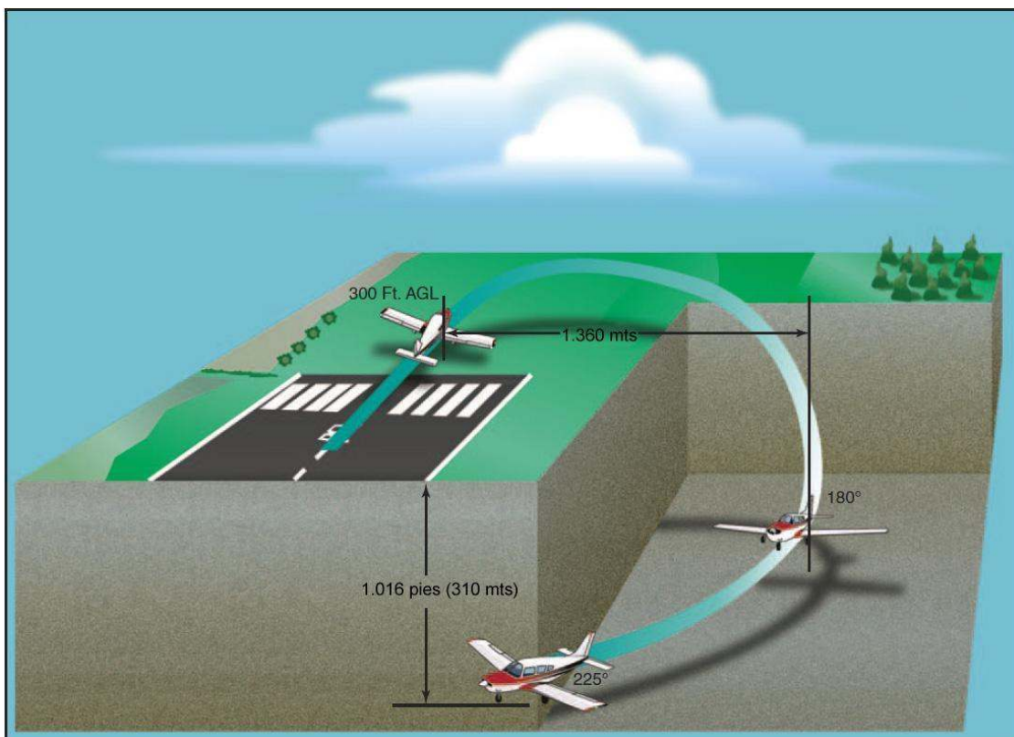
Figura 14-5. Viraje de retorno a la pista después de una falla de motor.
