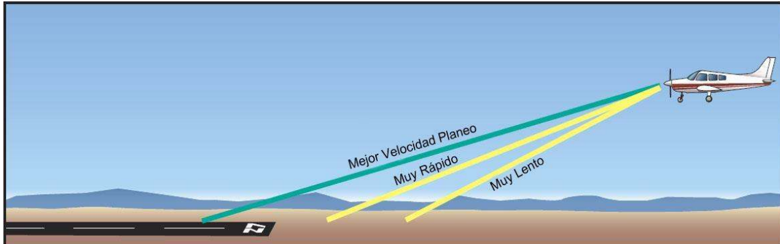
Figura 3-18. La mejor velocidad de planeo proporciona la mejor distancia recorrida para una pérdida de altura dada.
