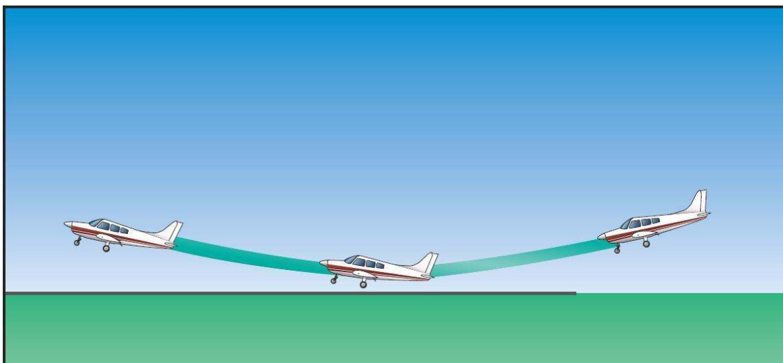
Figura 8-34. Globo durante el Flare.
