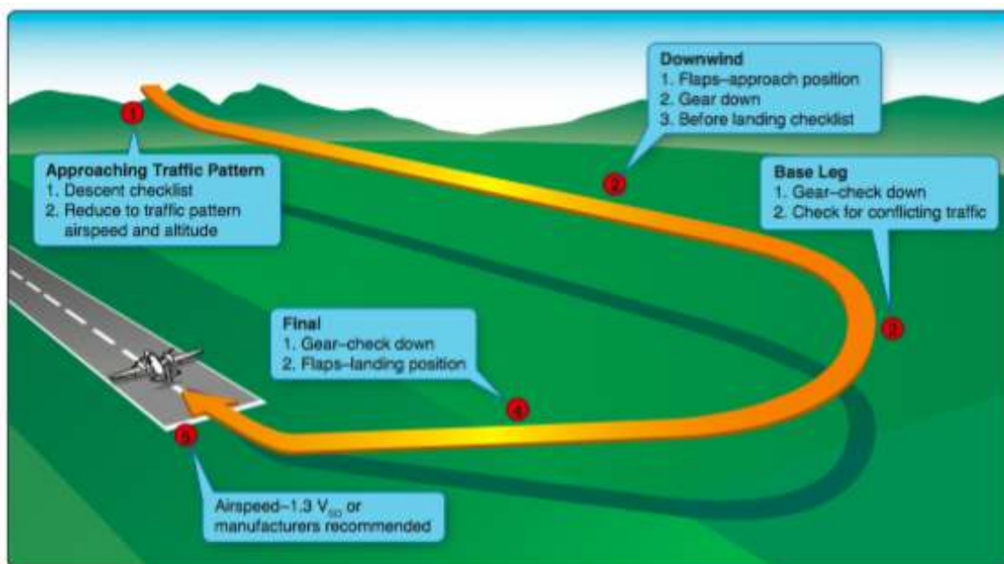
Figura 12-8. Aproximación y aterrizaje normal con un bimotor
