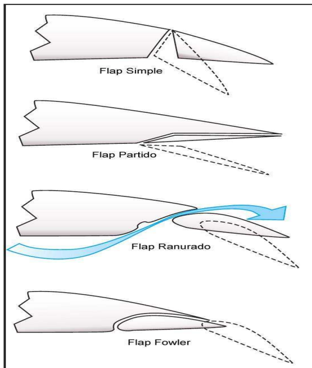
Figura 11-2. Cuatro tipos básicos de flaps.
