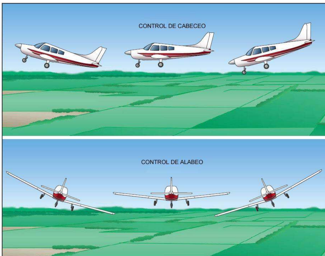
Figura 3-1. La actitud. Posiciones relativas de la nariz y alas con el horizonte natural.
