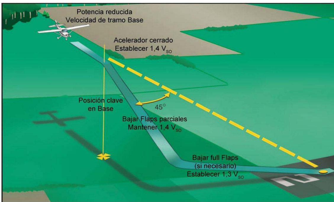
Figura 8-26. Aproximación sin potencia de 90°.
