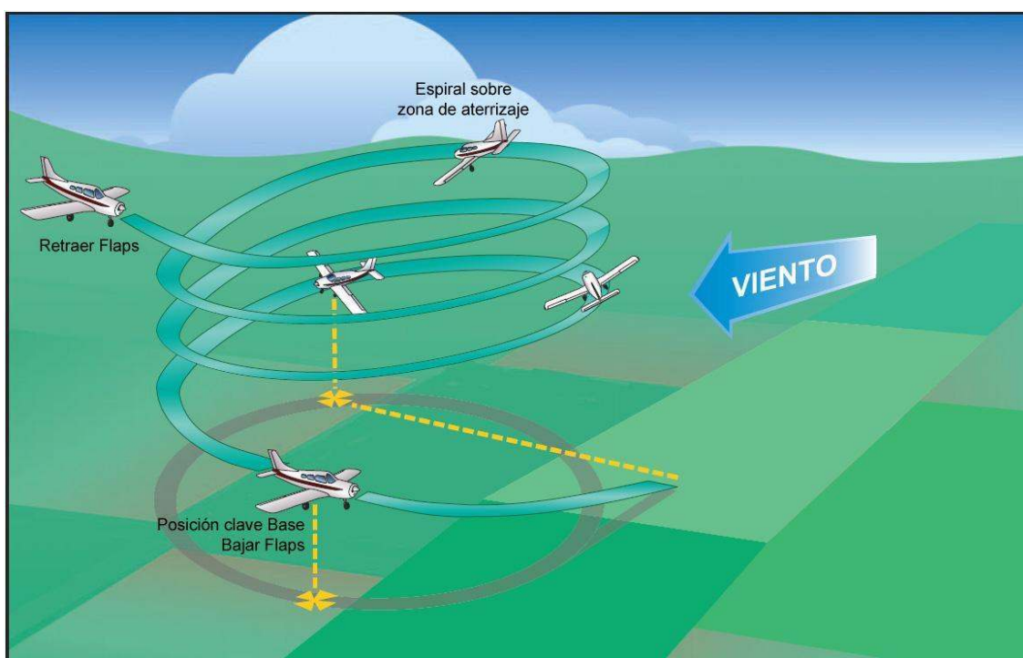
Figura 8-29. Permanezca sobre el área de aterrizaje seleccionada.
