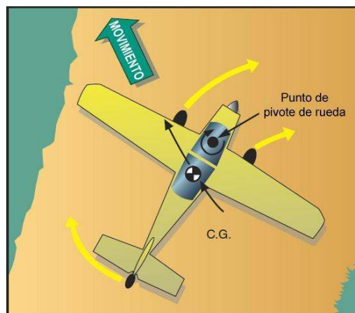
Figura 13-2. Efecto del CG sobre el control direccional.
