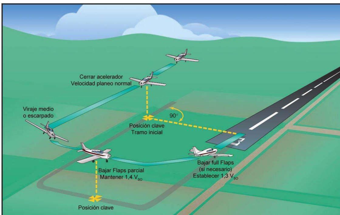
Figura 8-27. Aproximación sin potencia de 180°.
