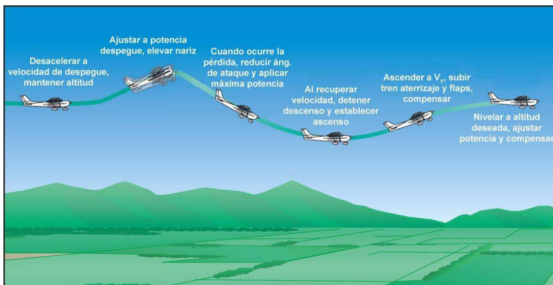
Figura 4-6. Pérdida con potencia y recuperación.
