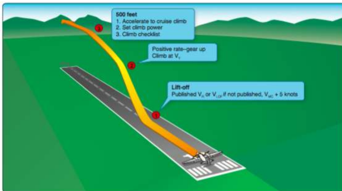
Figura 12-7. Perfil de despegue y ascenso.
