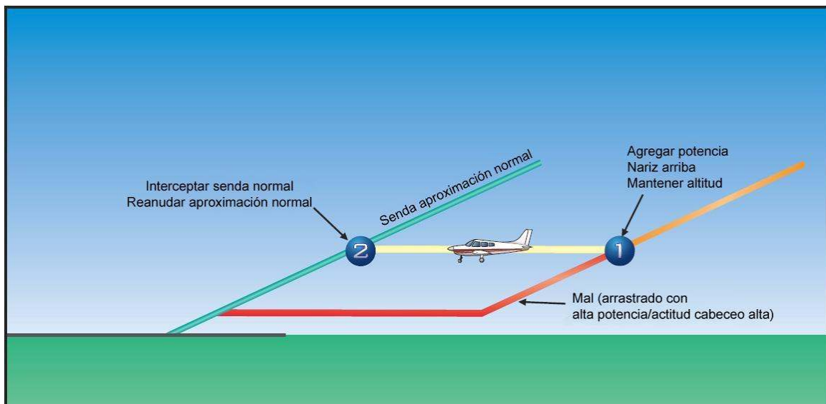
Figura 8-30. Métodos correctos e incorrectos de corregir una baja aproximación final.
