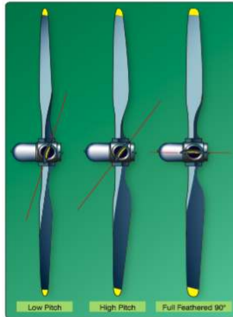
Figura 12-2. Hélice en bandera.
