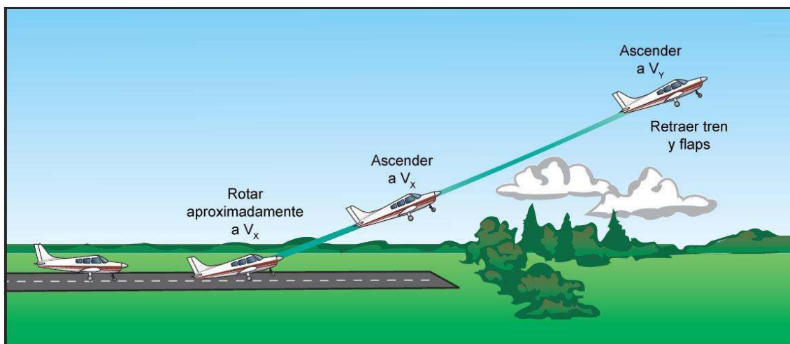
Figura 5-7. Despegue en campo corto.
