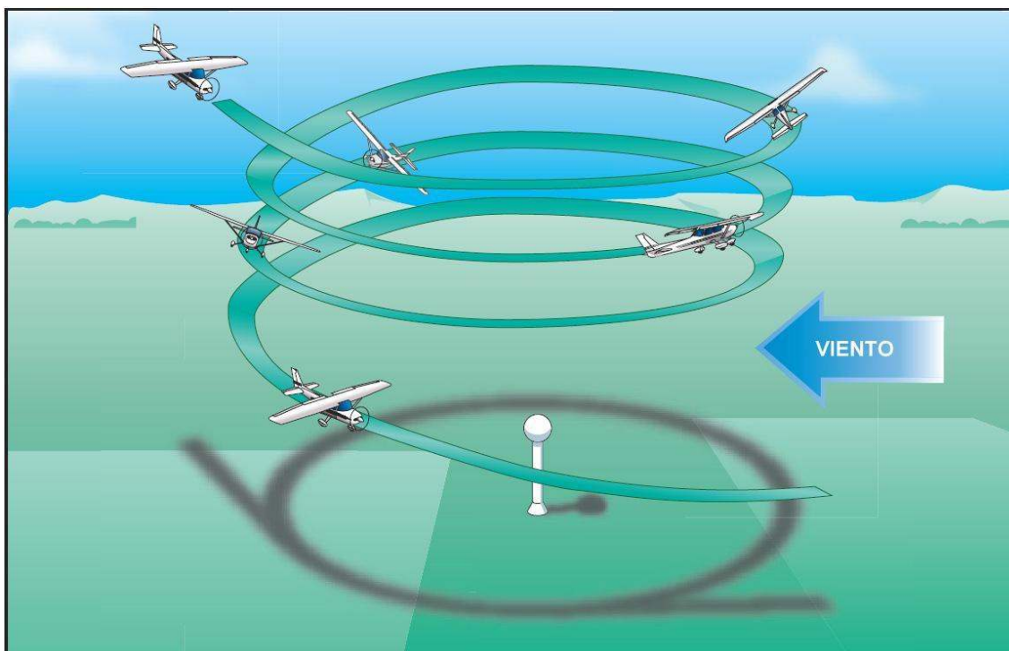
Figura 9-2. Espiral escarpada.
