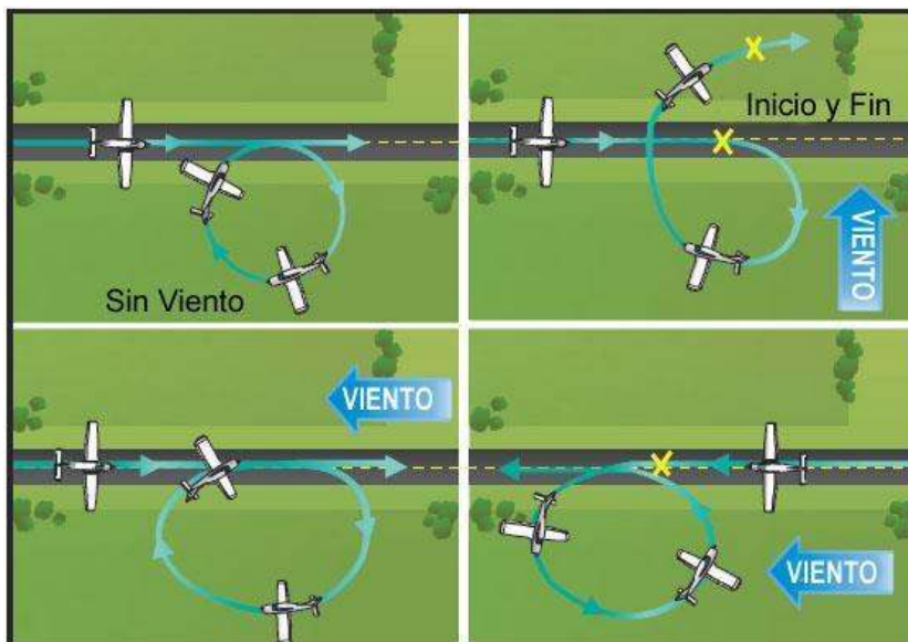
Figura 6-3. Efecto del viento durante virajes.
