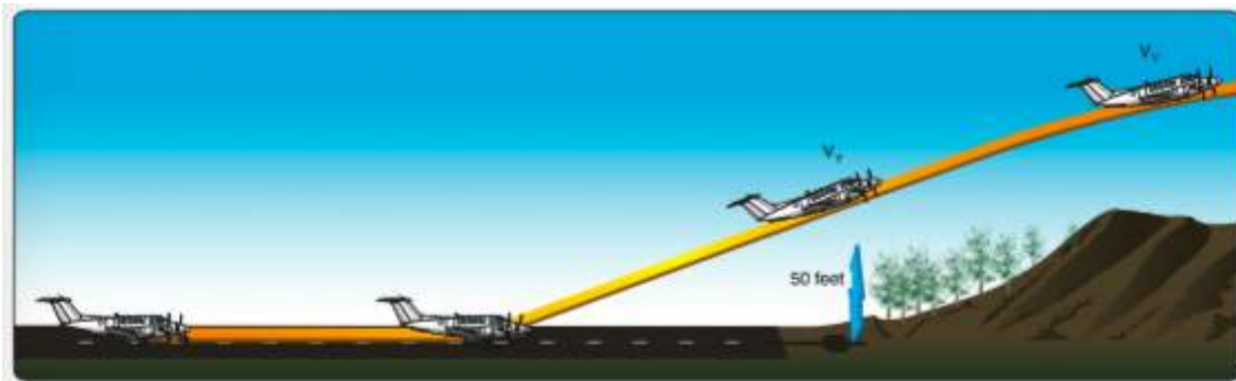
Figura 12-9. Despegue y ascenso en campo corto.
