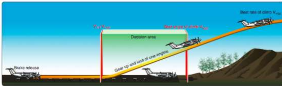
Figura 12-6. Área de decisión para la falla del motor después del despegue.
