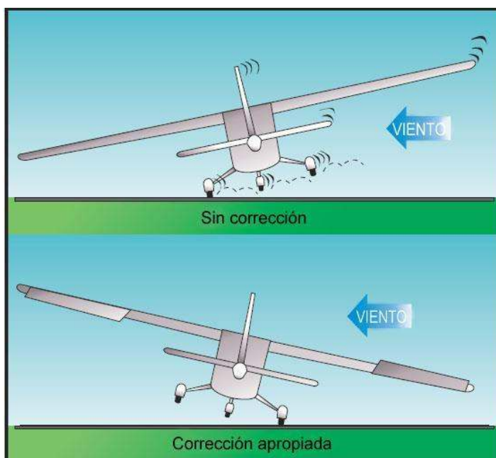
Figura 5-4. Efecto del viento cruzado.
