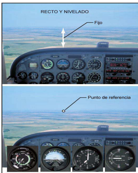
Figura 3-3. Referencia de nariz para vuelo recto y nivelado.
