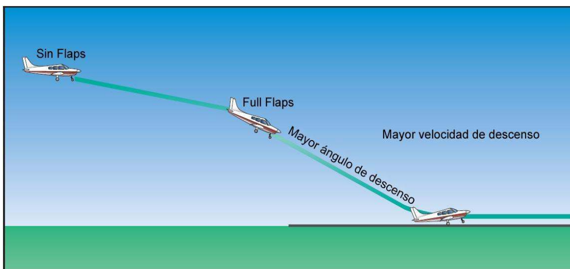
Figura 8-31. Cambio en la senda de descenso e incremento del régimen de descenso por una alta aproximación final.
