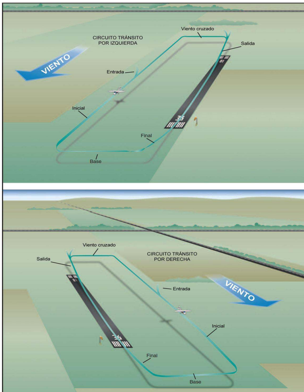
Figura 7-1. Circuitos de tránsito.
