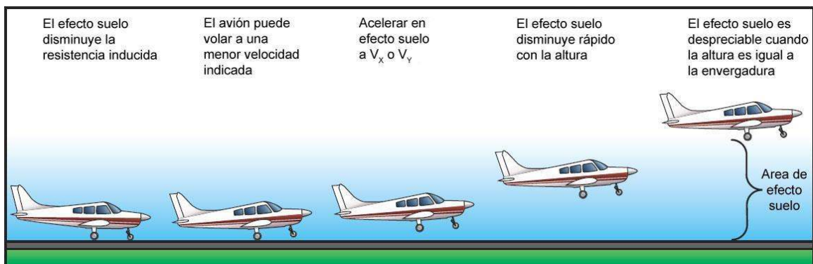
Figura 5-6. Despegue en zona de efecto suelo.
