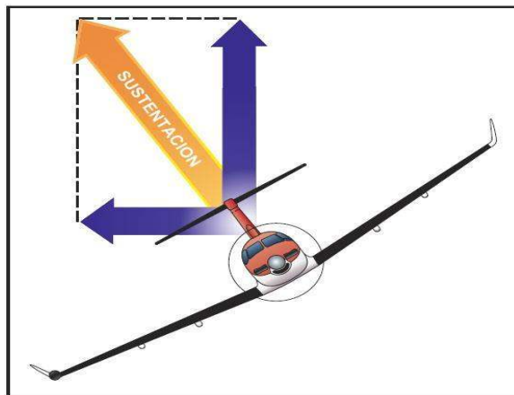
Figura 3-6. El cambio en la sustentación produce que el avión vire.
