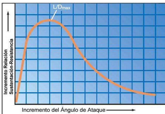
Figura 3-17. L/D MAX .
