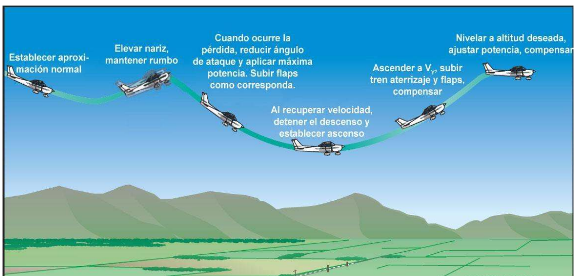
Figura 4-5. Pérdida sin potencia y recuperación.
