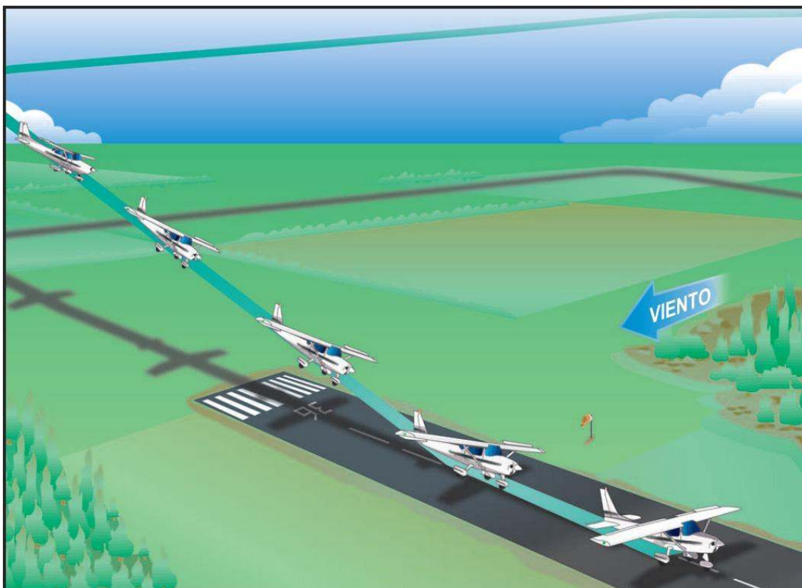
Figura 8-17. Aproximación y aterrizaje con viento cruzado.
