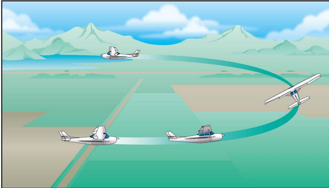
Figura 9-3. Chandelle.
