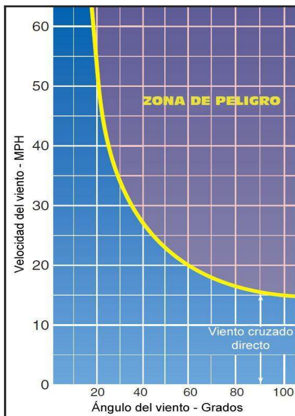
Figura 8-18. Tabla de viento cruzado.
