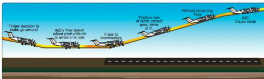
Figura 12-10 Procedimiento de escape
