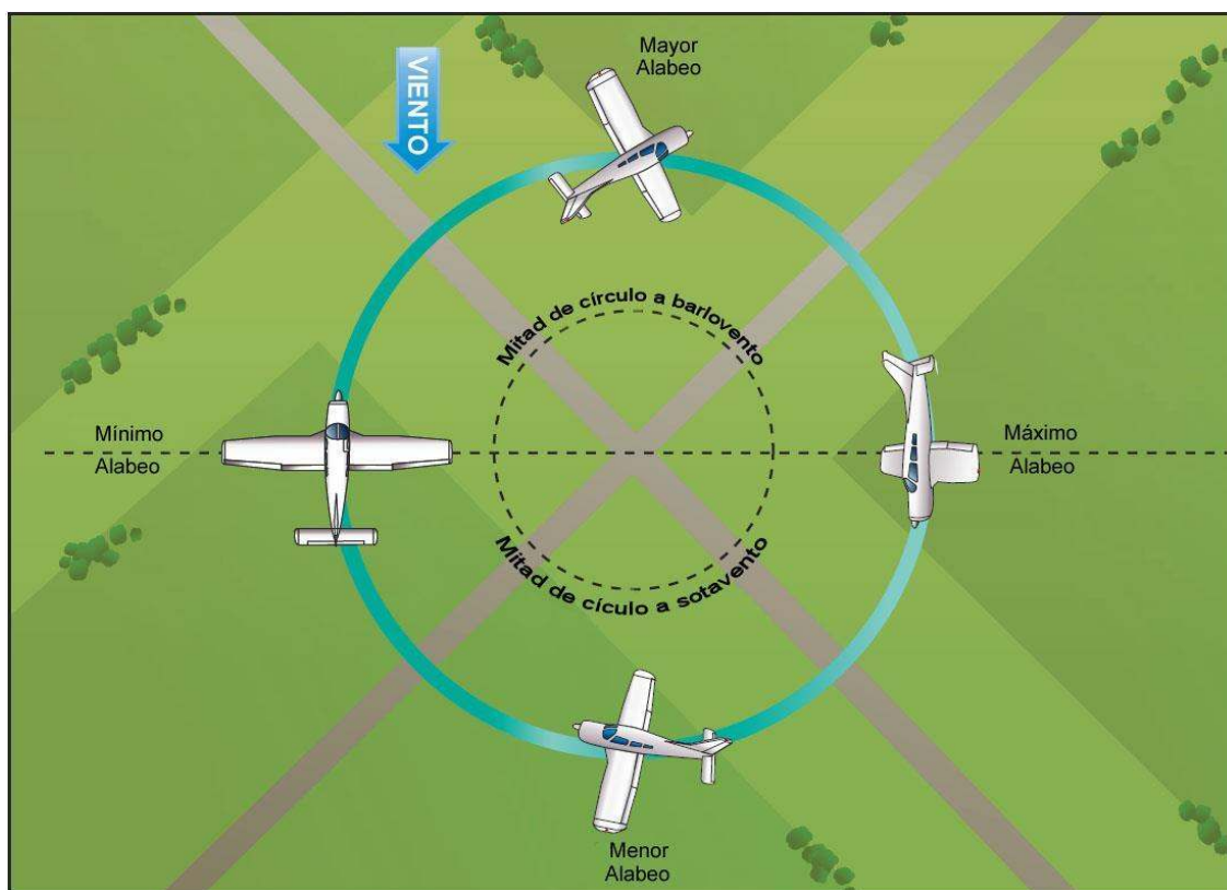
Figura 6-6. Virajes alrededor de un punto.
