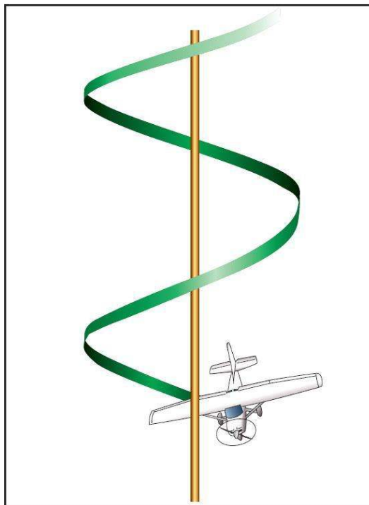
Figura 4-9. Barrena; una pérdida agravada y autorrotación
