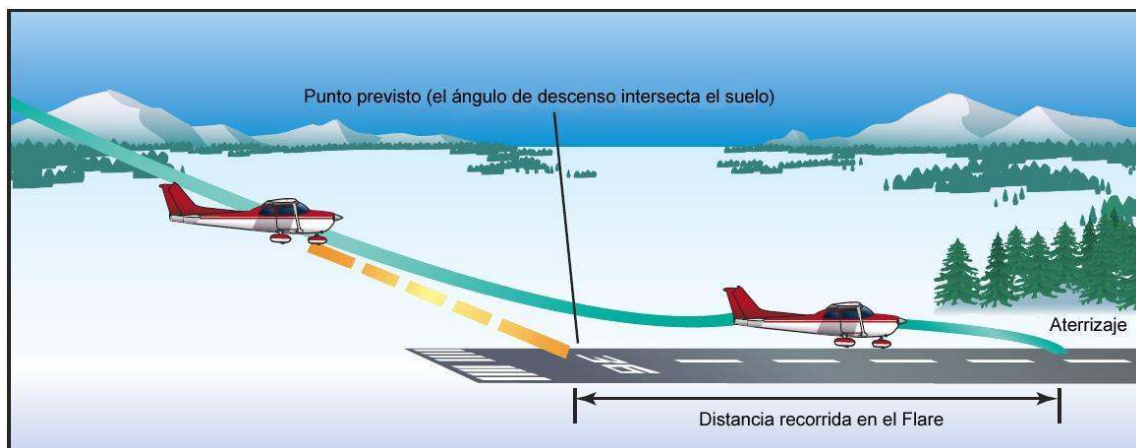
Figura 8-9. Aproximación estabilizada.
