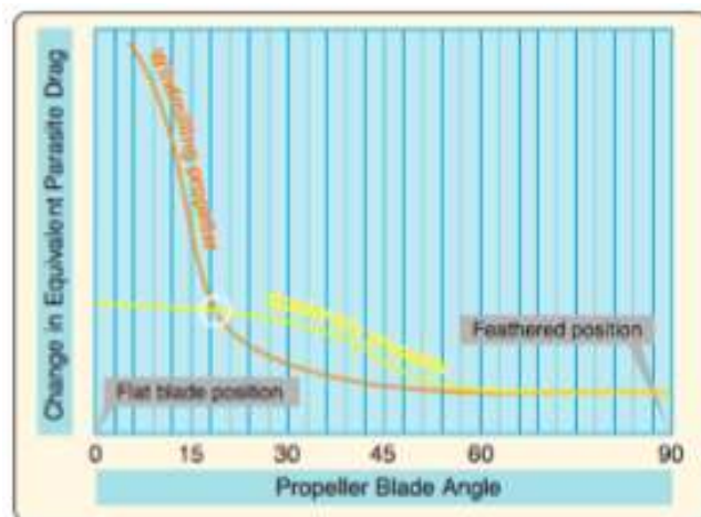
Figura 12-3. Contribución de resistencia aerodinámica de la hélice
