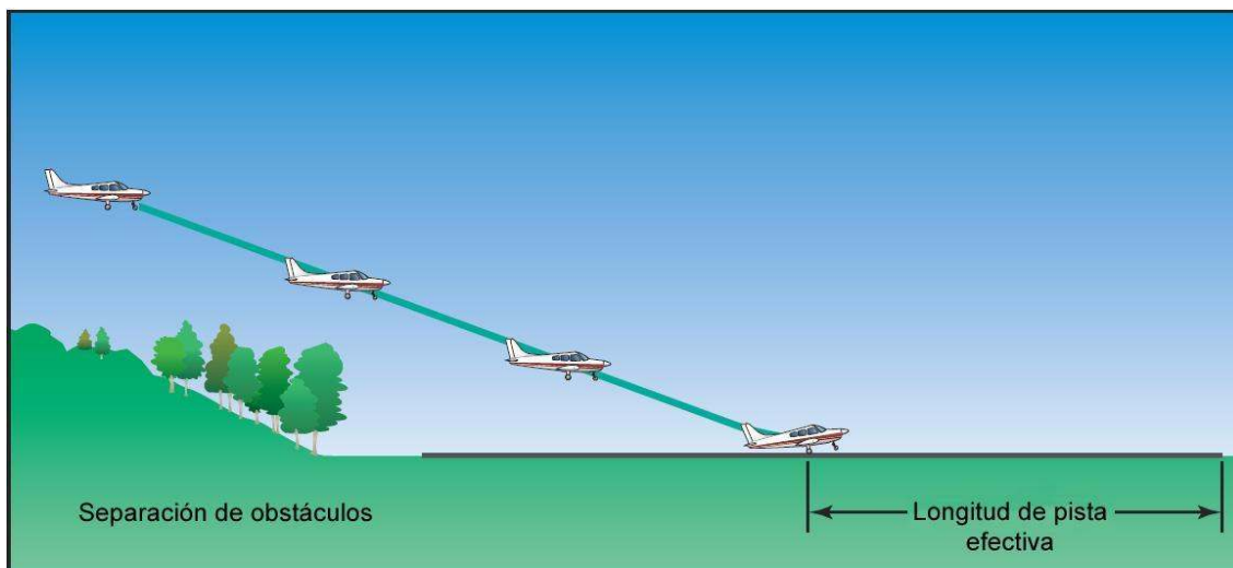
Figura 8-20. Aterrizaje sobre un obstáculo.
