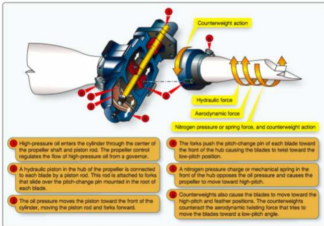
Figura 12-4. Cambio de tono de las fuerzas.
