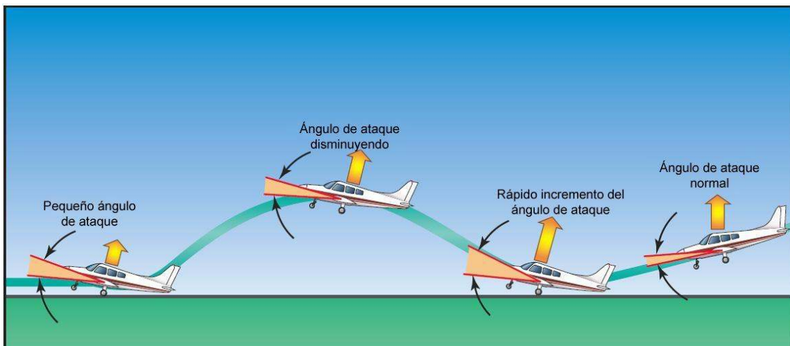
Figura 8-35. Rebote durante la toma.
