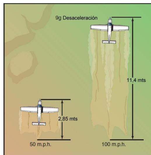
Figura 14-2. Distancia de frenado vs. velocidad.
