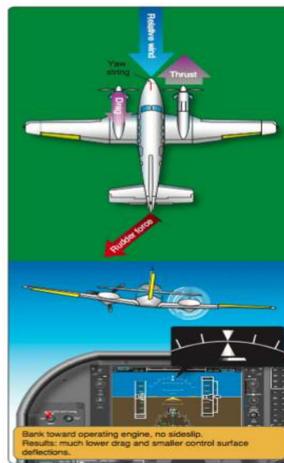
Figura 12-18. Cero deslizamiento lateral.
