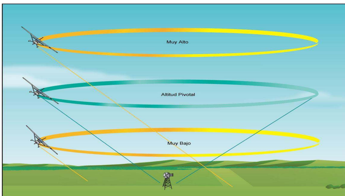
Figura 6-13. Efecto de diferentes alturas en la altura pivotal.
