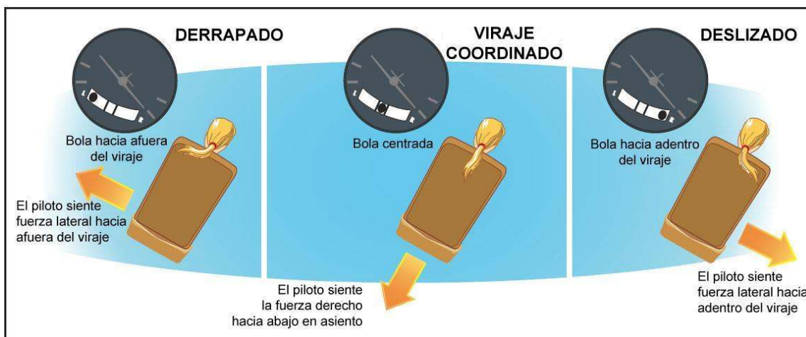
Figura 3-8. Indicaciones de un deslizamiento y derrape.
