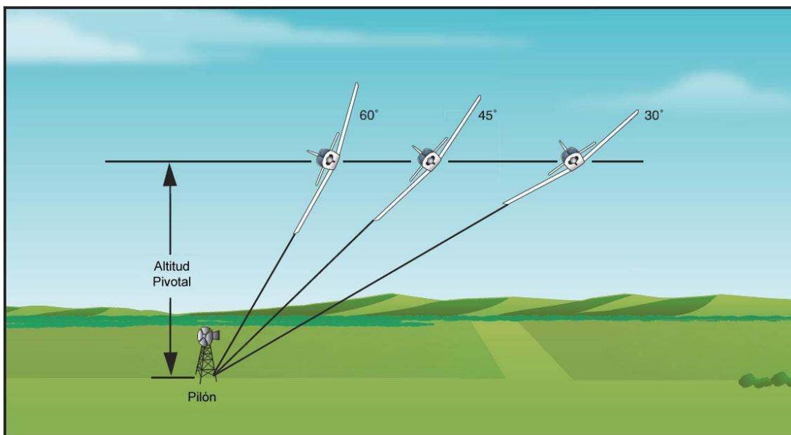
Figura 6-14. Ángulo de alabeo vs altura pivotal.
