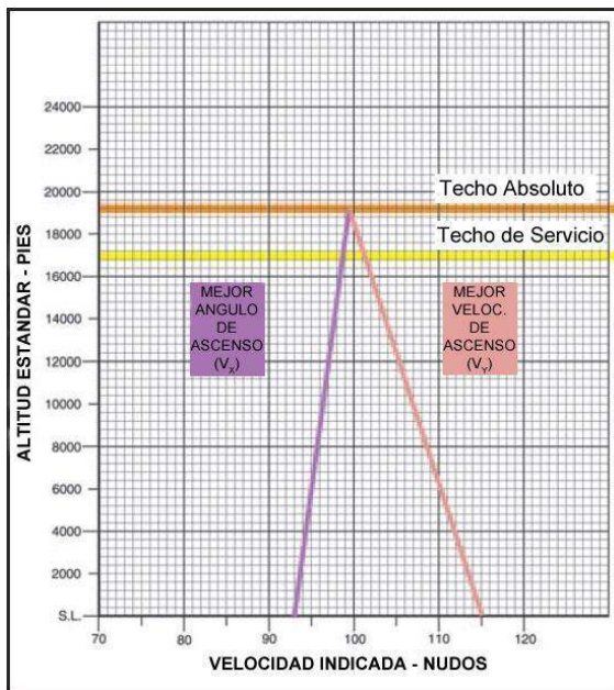
Figura 3-15. Techo absoluto.
