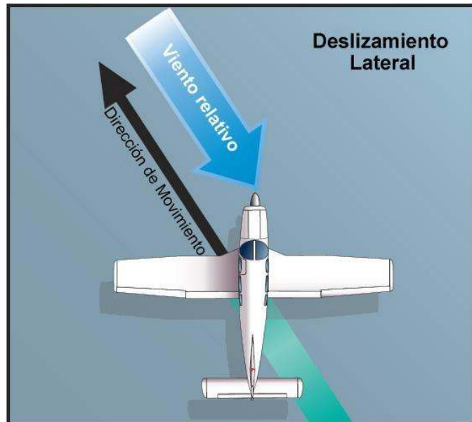
Figura 8-12. Deslizamiento lateral.
