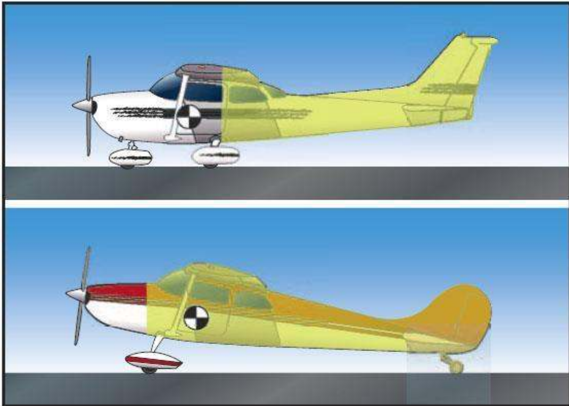
Figura 2-19. Área de superficie más afectada por el viento.
