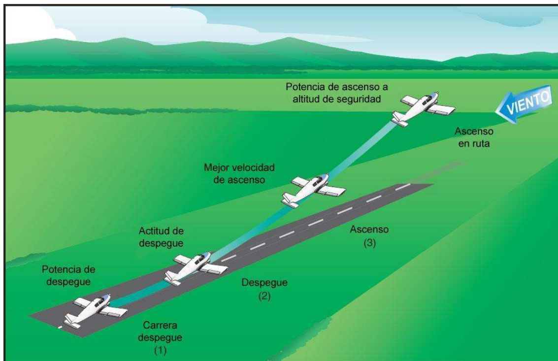
Figura 5-1. Despegue y ascenso.
