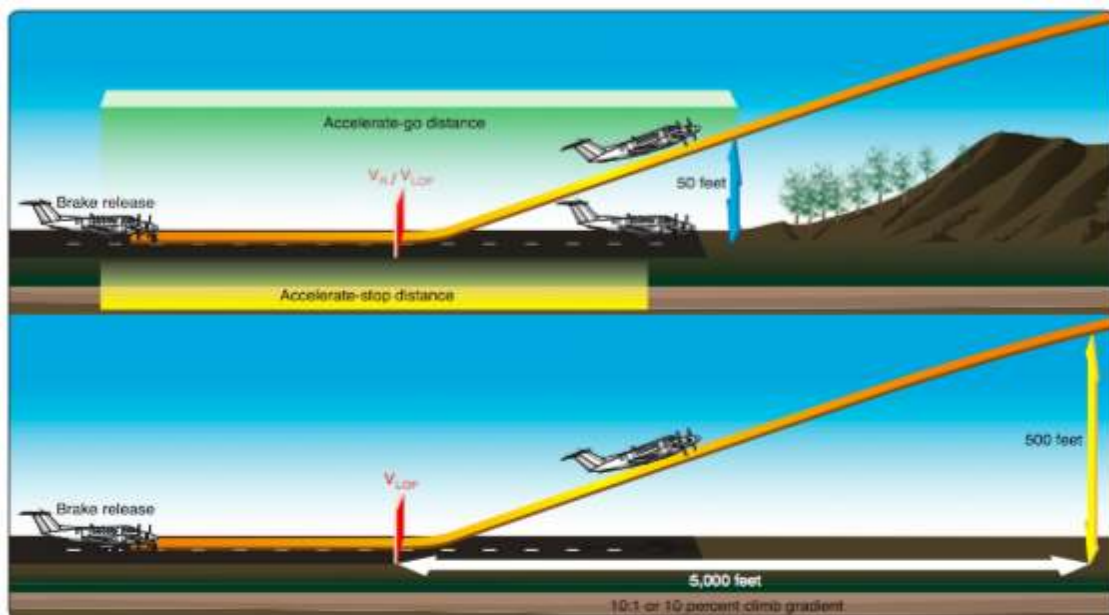
Figura 12-5. Acelere, detenga la distancia, acelere, recorra la distancia y suba el gradiente.
