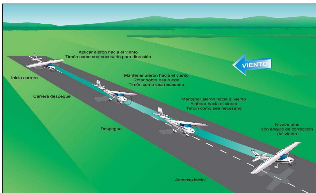
Figura 5-3. Carrera de despegue y ascenso inicial con viento cruzado.
