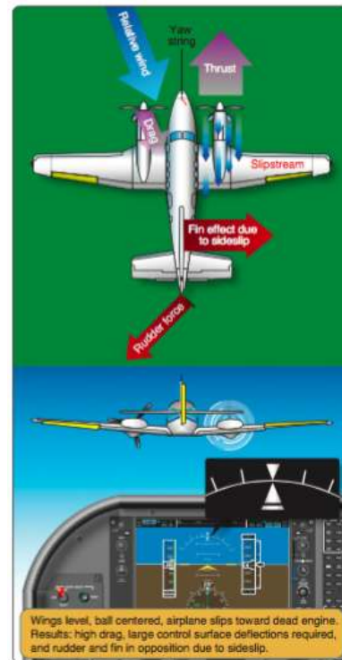
Figura 12-16. Alas niveladas en vuelo con un sólo motor.
