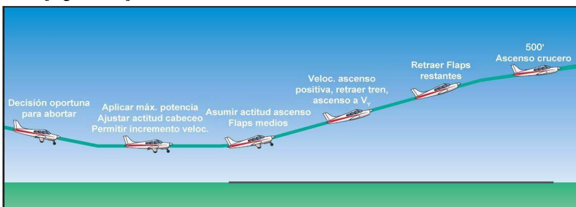
Figura 8-14. Procedimiento de aproximación frustrada.
