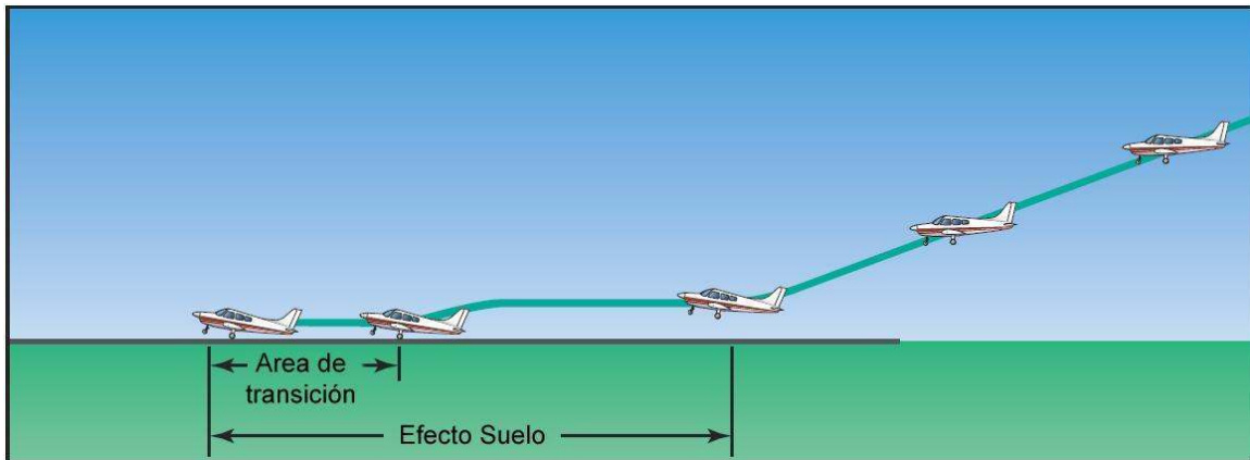
Figura 8-24. Aproximación y aterrizaje en campo blando/rugoso.
