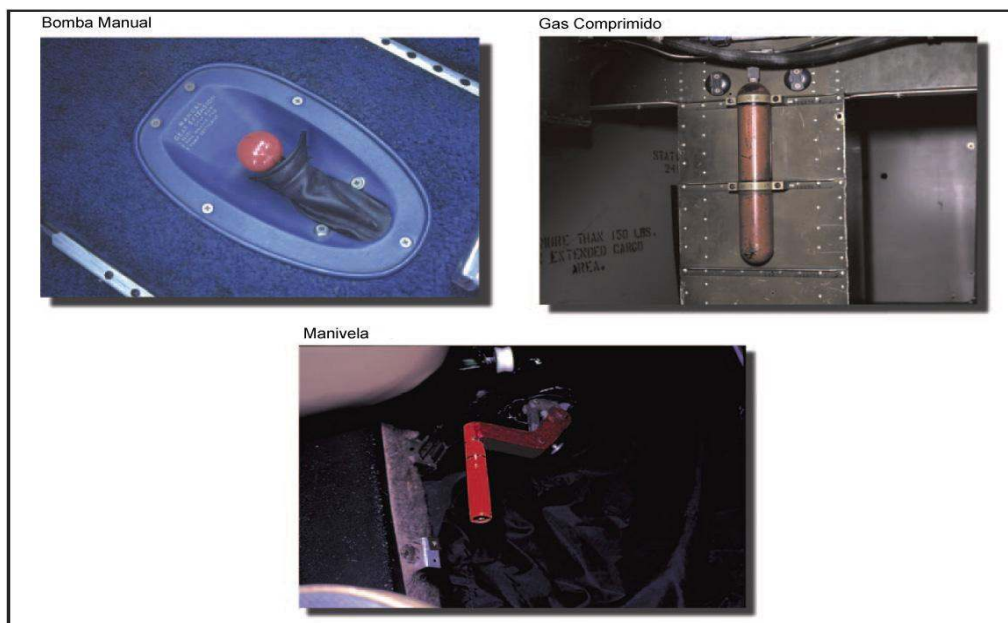
Figura 11-9. Sistemas típicos de extensión del tren de aterrizaje en emergencia.
