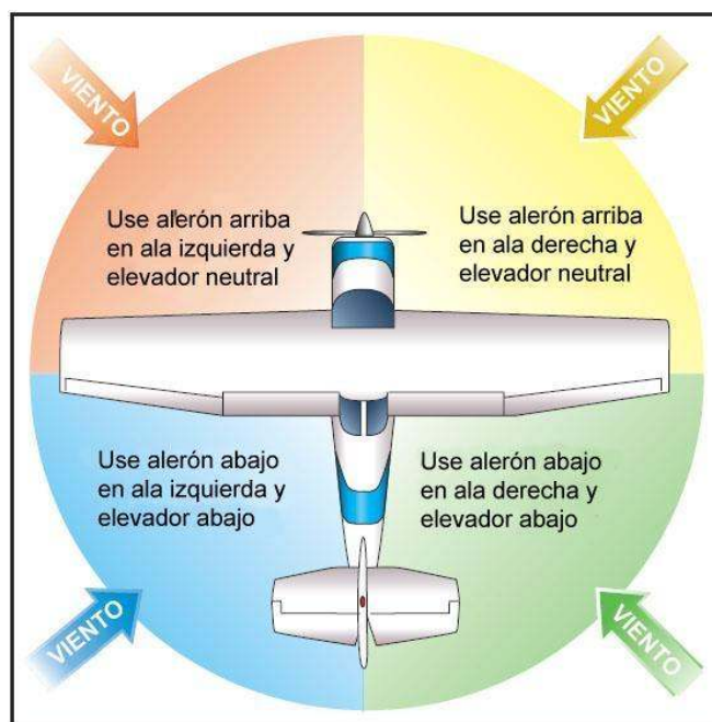
Figura 2-15. Posición de los controles durante el rodaje.
