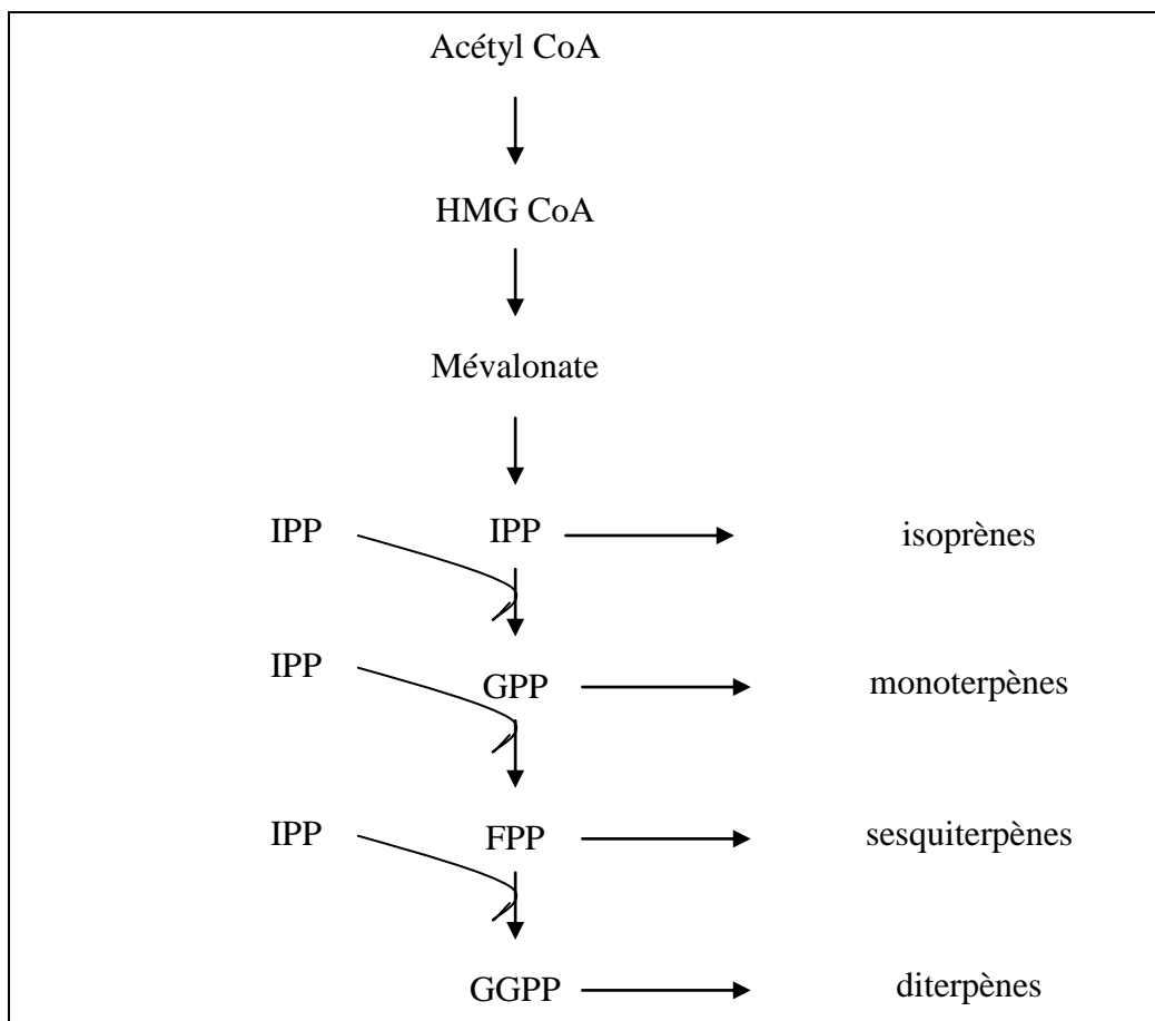
Figure 69 : Schéma simplifié de la voie de biosynthèse des composés terpéniques [238].
