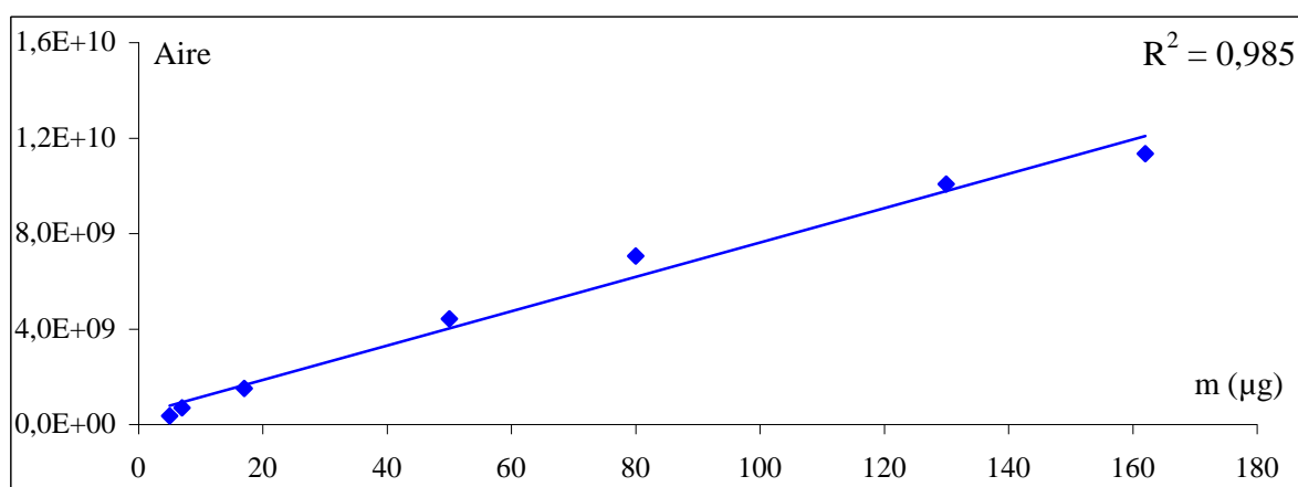
Figure 76 : Droite d'étalonnage de l' \alpha -pinène.
