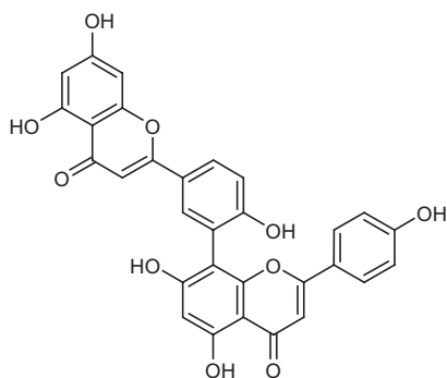
Amentoflavone
