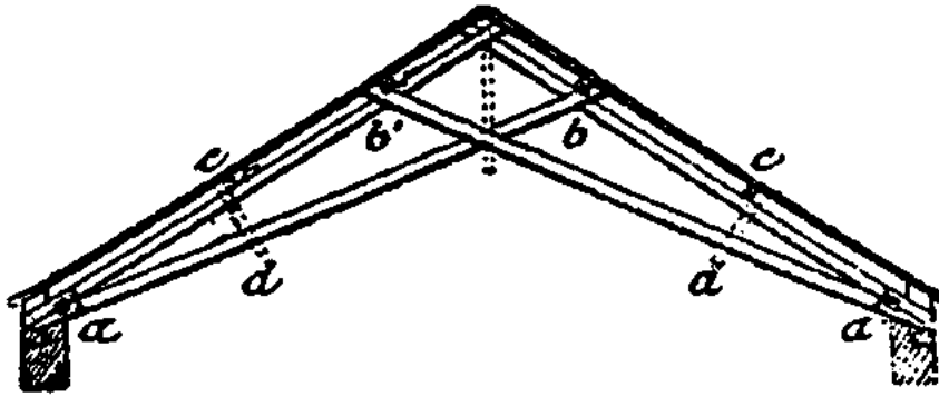
Fig. 226.—Cercha de tijera sin tirante.
