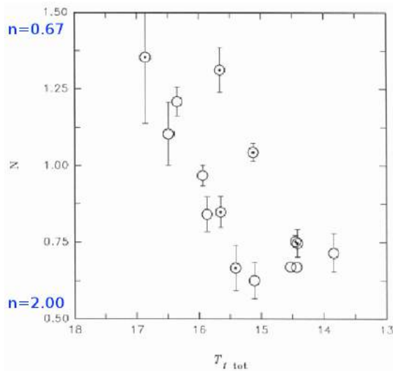
Figura 6.9: Relación entre el parámetro de Sérsic y la luminosidad. Izq. : N(\equiv n^{-1}) contra magnitud aparente integrada T_1 para galaxias del cúmulo de Fornax (Cellone et al., 1994); Der. : \log(n) contra M_B para galaxias tempranas del cúmulo de Virgo (Jerjen & Binggeli, 1997).
