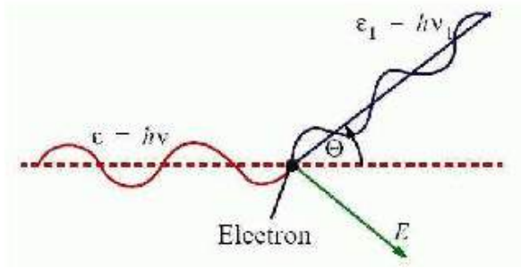
Figura A.4: Geometría del proceso Compton.
