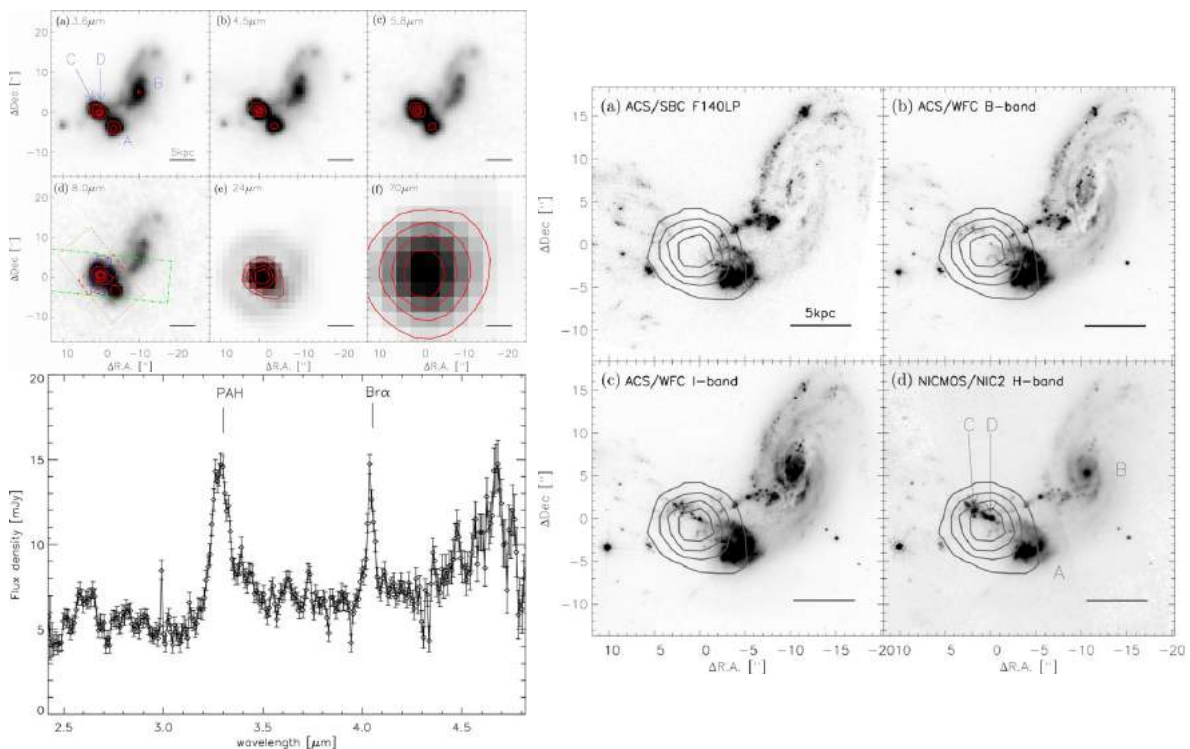
Figura 6.27: Galaxia ULIRG II Zw96. Izq., arriba: imágenes Spitzer, en las bandas indicadas. Der.: imágenes HST, + contornos Spitzer 24 μm. Izq., abajo: espectro IR. (Inami et al., 2010).
