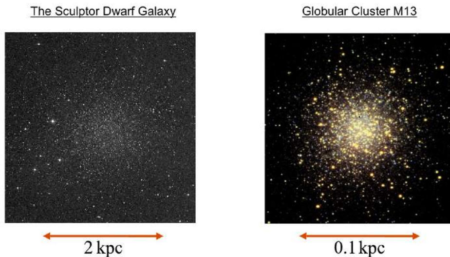
Figura 6.2: Comparaci6n entre la galaxia dSph Sculptor y el c6mulo globular M 13. Tienen luminosidades similares ( M_V = -10.7 \equiv \mathcal{L}_V = 1.4 \times 10^6 \mathcal{L}_\odot ) pero tama1os muy diferentes.
