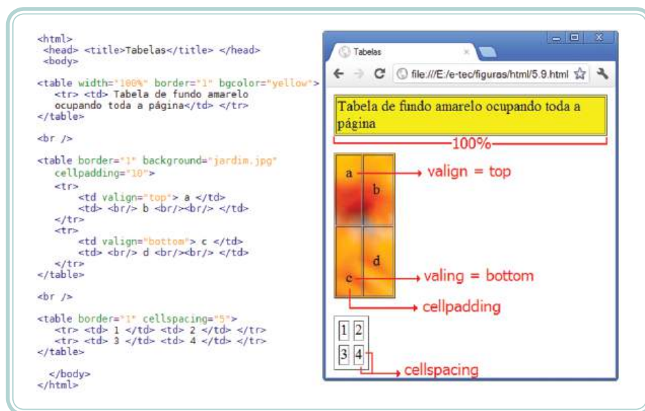
Figura 5.9: Atributos adicionais para estruturação de tabelas
