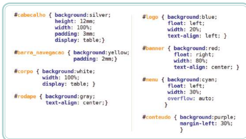
Figura 8.6: Estrutura do documento usando regras CSS
