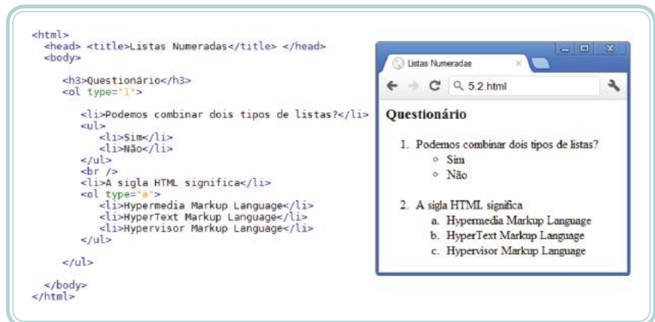
Figura 5.2: Documento HTML utilizando listas numeradas
