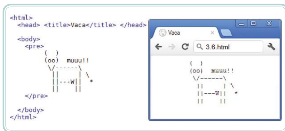
Figura 3.5: Exemplo de utilização da tag <pre>
