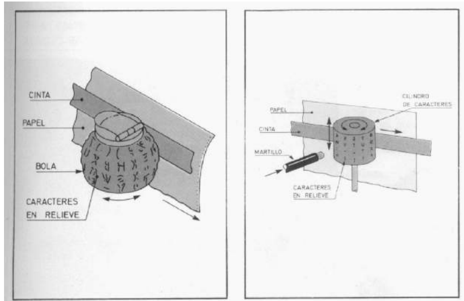
Figura 2.11: Impresora de Bola y Cilindro
