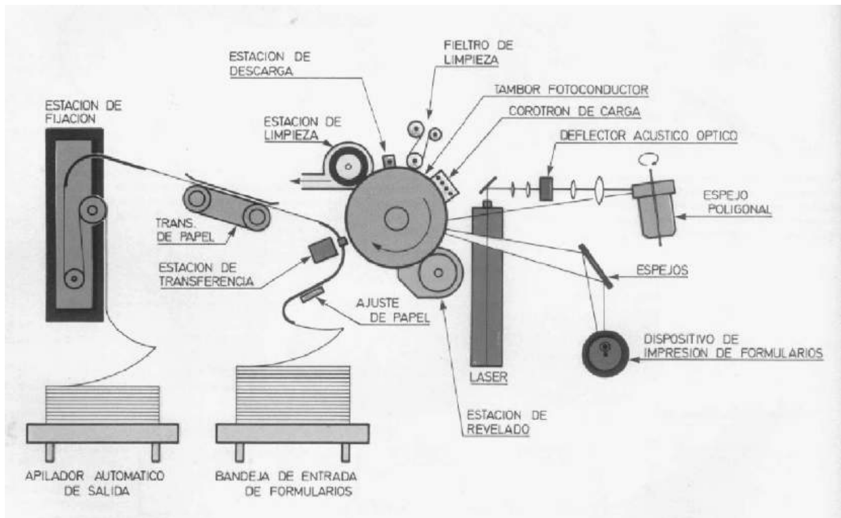
Figura 2.14: Impresora Laser
