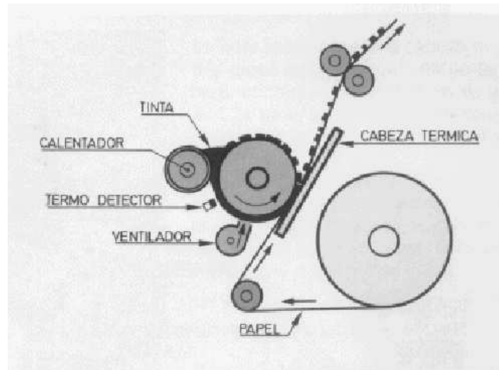
Figura 2.13: Impresora de Transferencia
