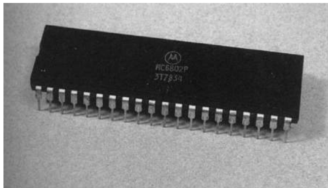
Figura 2.21: Microprocesador
