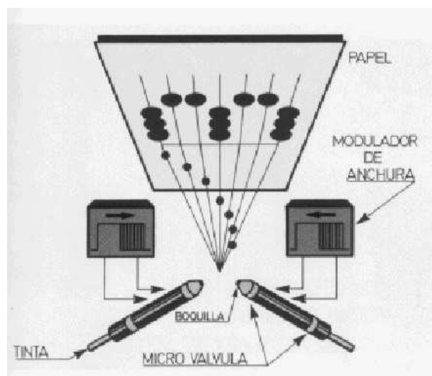
Figura 2.12: Impresora Chorro de Tinta
