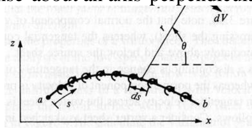
vortex sheet
