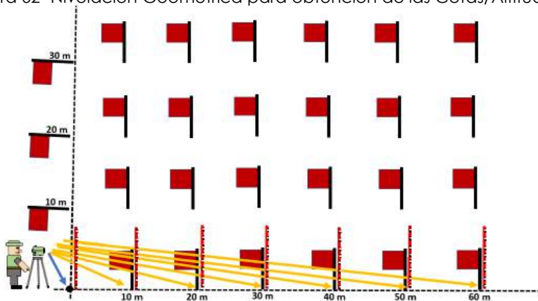
Figura 62- Nivelación Geométrica para obtención de las Cotas/Altitudes.
