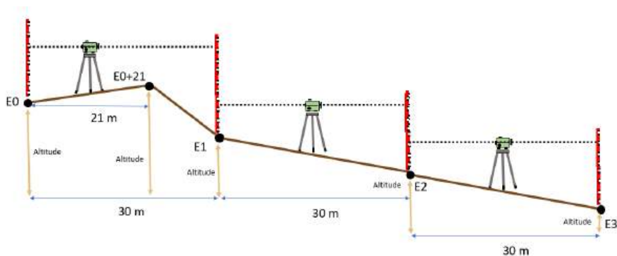
Figura 28 – Estaquiamento con Estacas Fraccionarias.
