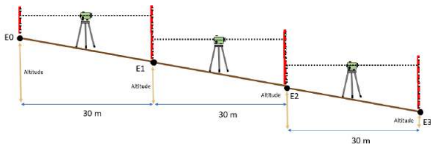
Figura 27 - Estaquiamiento topográfico.
