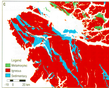
Mapa geológico reclasificado en 3 clases de acuerdo a la litología
