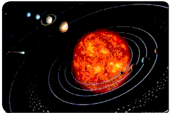
Gambar 7.8. Planet-planet berputar di porosnya. Sumber: http://arisudev.wordpress.com
