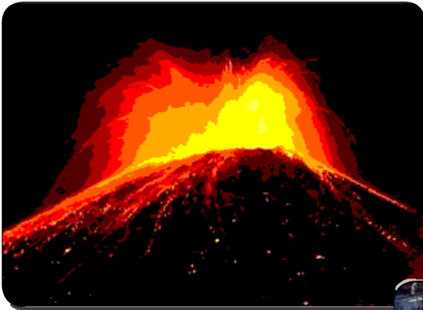
Gambar 2.2. Gunung api meletus. Sumber: http://pixshark.com
