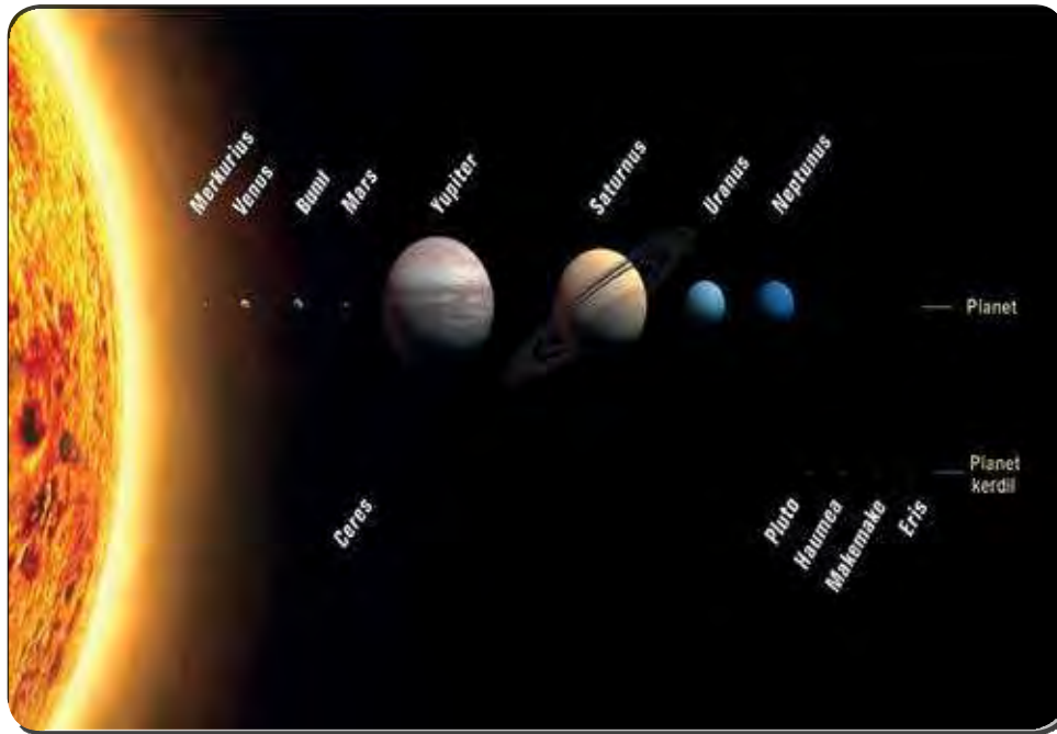
Gambar 2.1. Tata surya. Sumber: http://id.wikipedia.org
