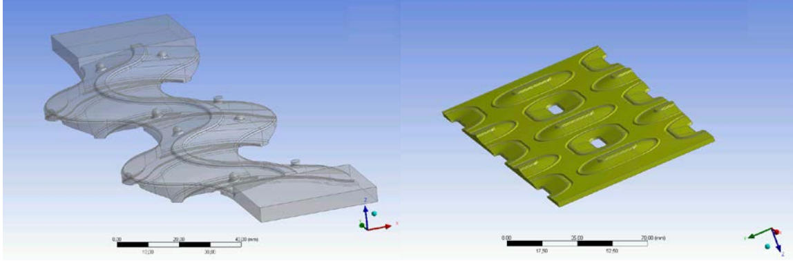
Şekil 2: Plakalı ısı değıştirci yüzeyleri Yüzey (a) ve Yüzey (b).
