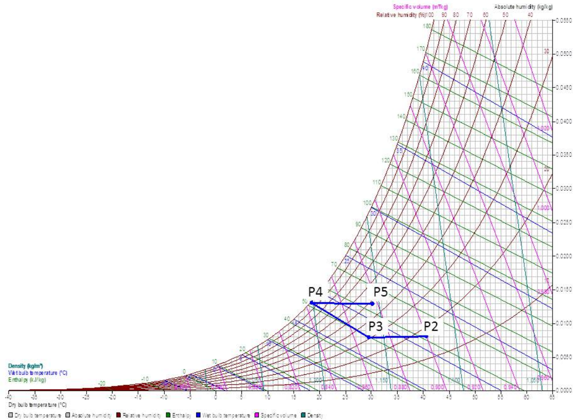
Şekil 4: Performans deney ölçümü, hava akış hızı 10000 m 3 /saat.
