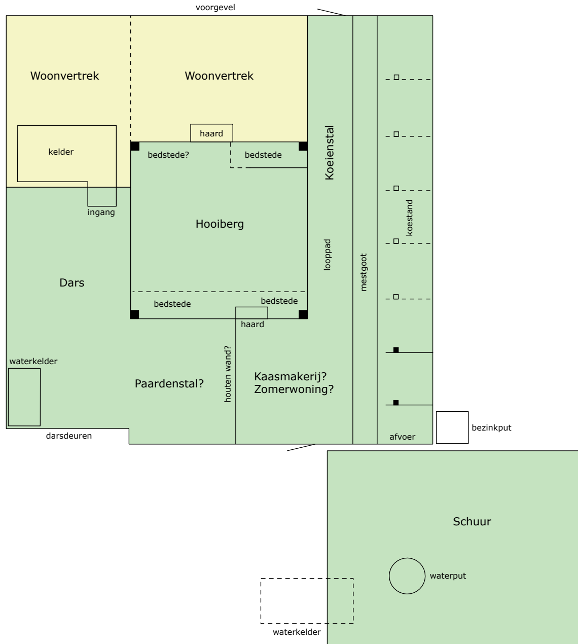
Afbeelding 27. Reconstructie van de plattegrond van de boerderij bij de bouw in 1877.
