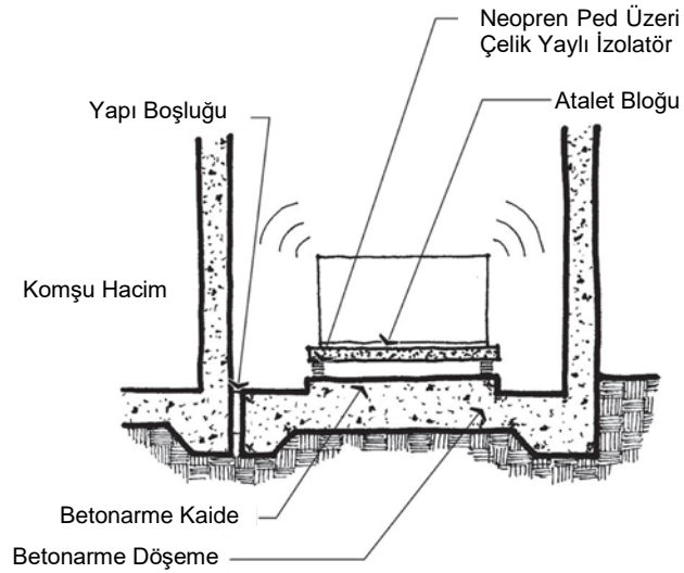
Şekil 1. Ayrılmış Betonarme [4]
