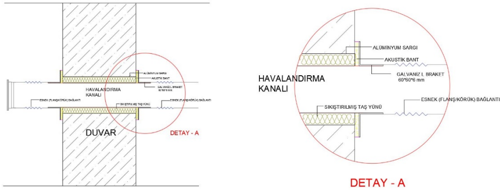
Şekil 5. Havalandırma Kanalı - Duvar Geçiş Detayı Gösterimi
