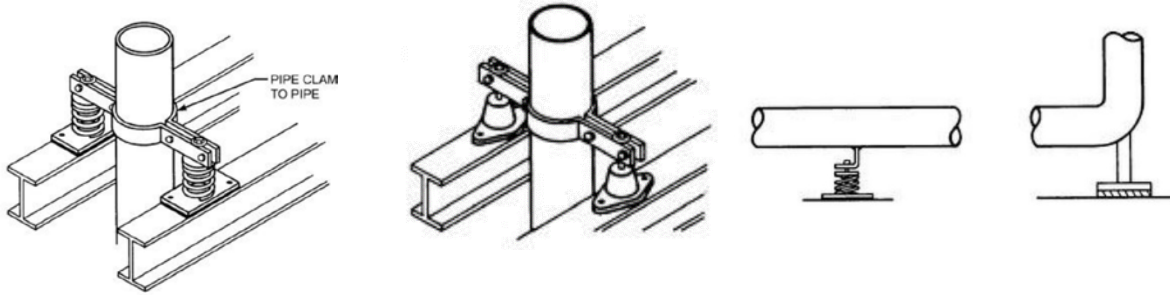
Şekil 2. Boru Esnek Bağlantı Gösterimleri[3]
