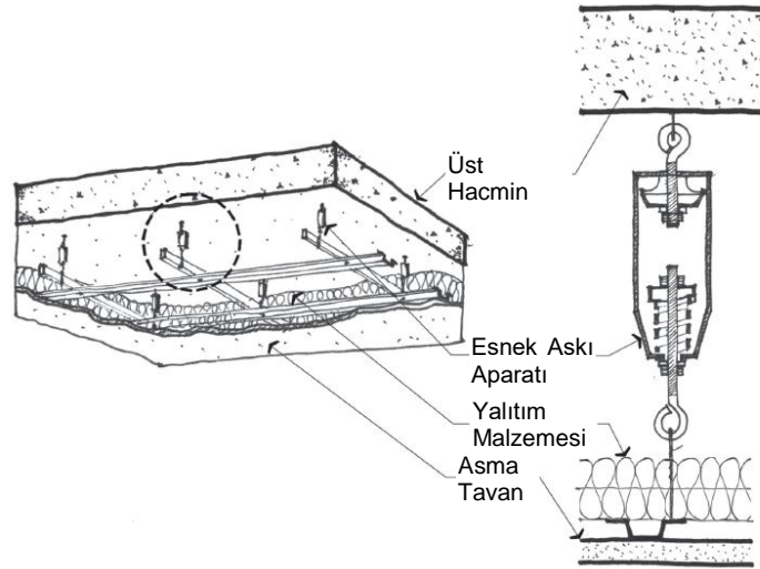
Şekil 9. Esnek Askı Aparatıyla Asma Tavan Uygulaması
