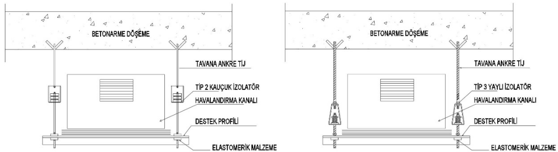
Şekil 3. Havalandırma Kanalı Esnek Bağlantı Gösterimi
