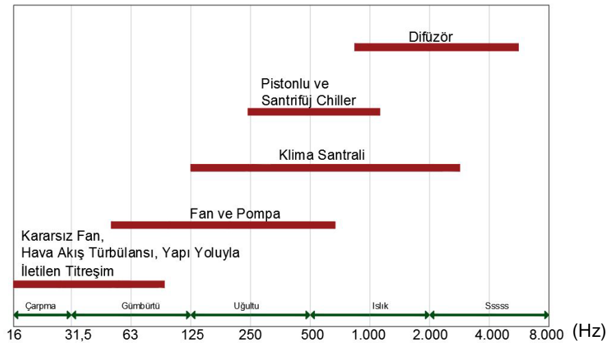
Şekil 6. Mekanik Cihaz Gürültülerinin Frekans Spektrumları [3]
