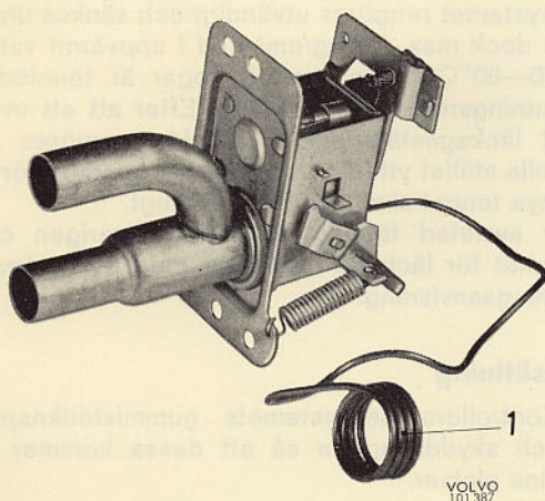
Bild 20. Värmekontrollventil 1. Termostats känslkropp
