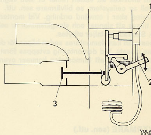
Bild 21. Förenklad skiss över värmekontrollventilens arbetssätt
