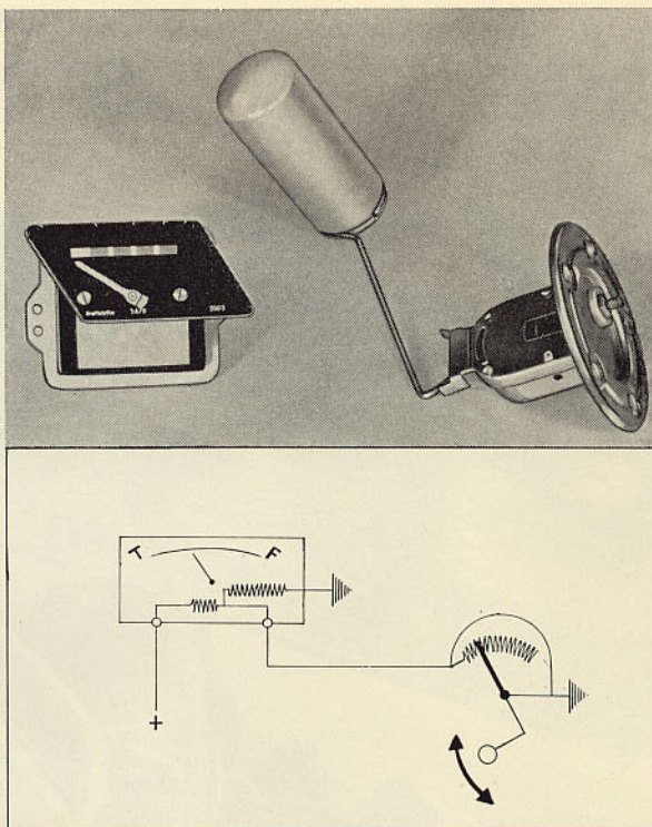
Bild 4. Bränslemätare
