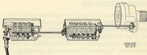
Bild 6. Principskiss på väg- resp. trippmätarens drivning
