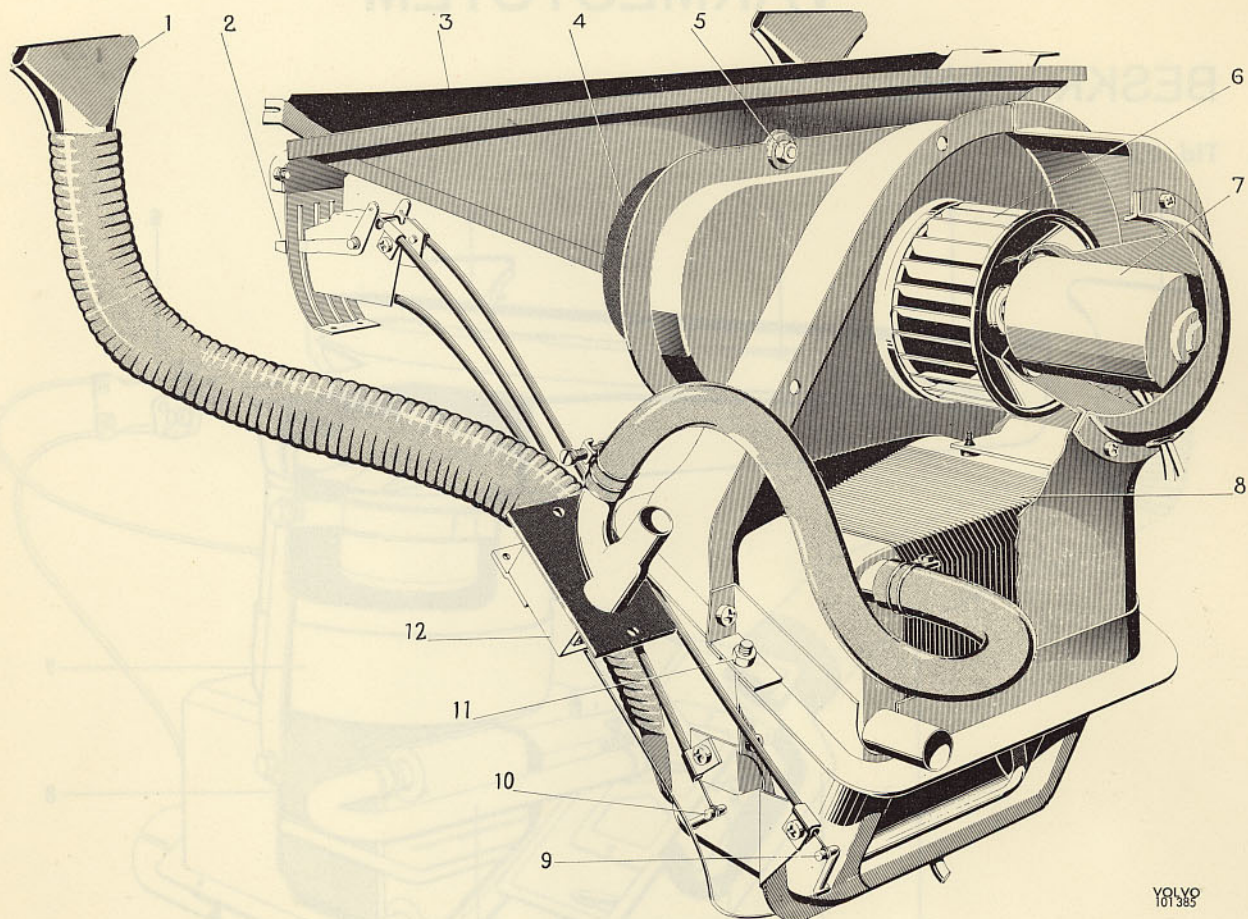
Bild 18. Bilvärmare
