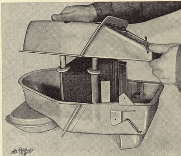
Bild 22. Isärtagning av bilvärmare
