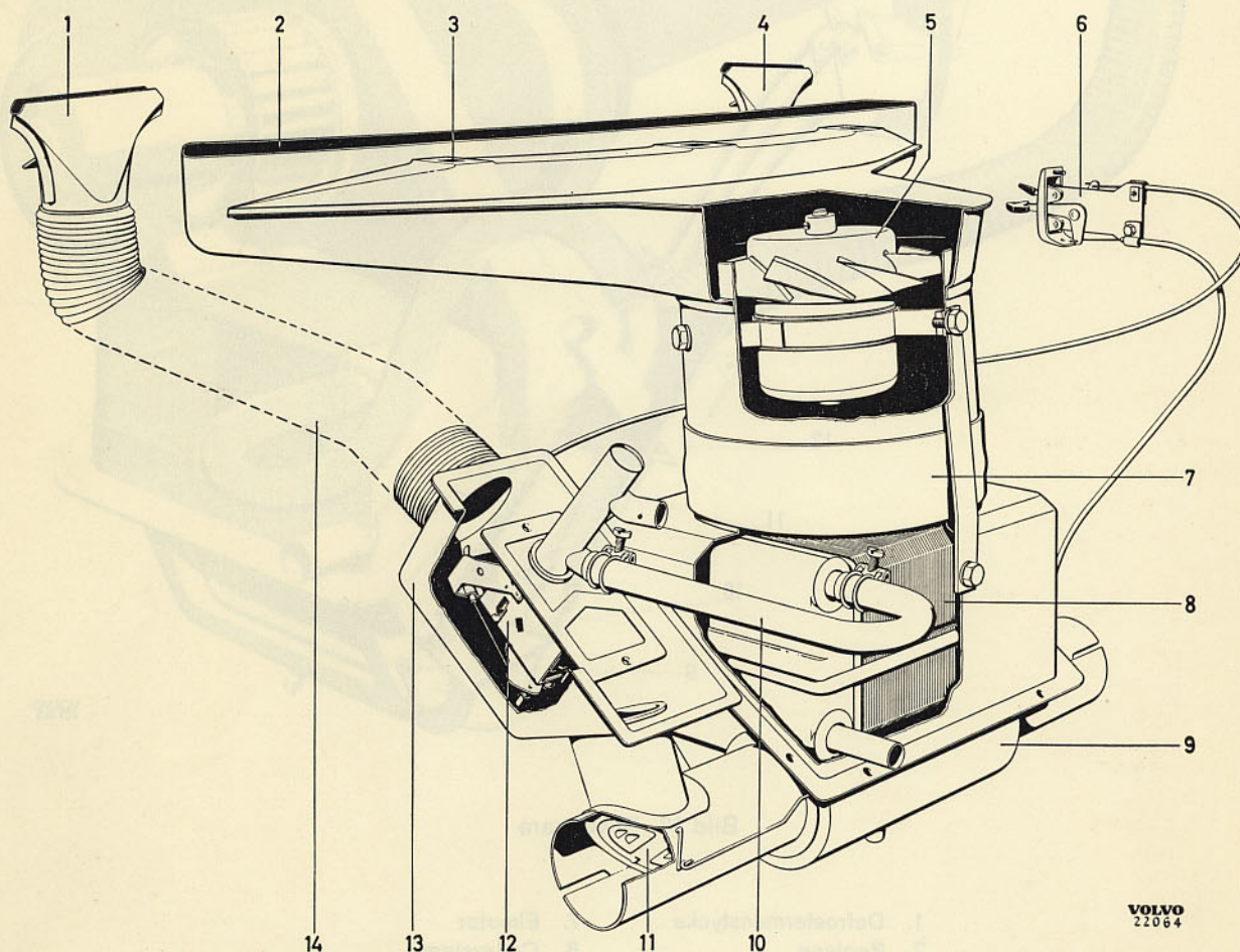
Bild 17. Bilvärmare
