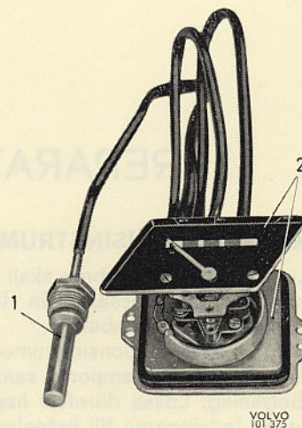
Bild 7. Temperaturmätare
