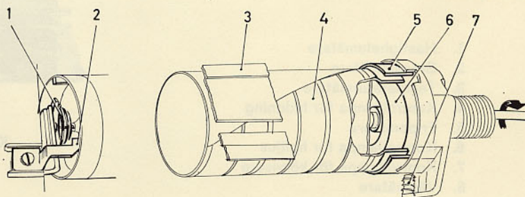
Bild 5. Hastighetsmätarens uppbyggnad
