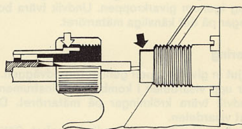
Bild 14. Anslutning av hastighetsmätarkabel, sen. utf.
