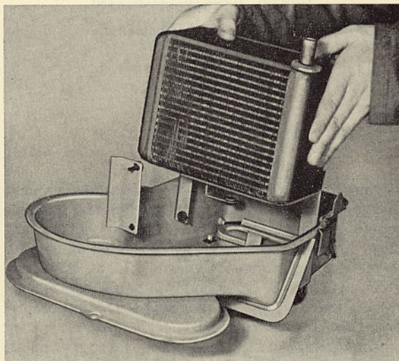
Bild 23. Insättning av bilvärmarens cellsystem
