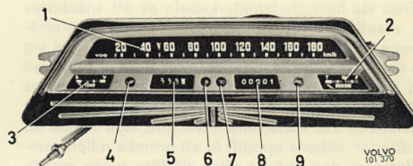
Bild 2. Kombinationsinstrument, framsida
