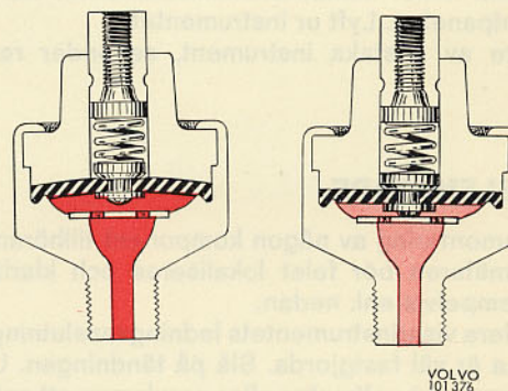
Bild 8. Oljetryckskontaktens funktion
