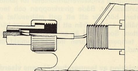
Bild 13. Anslutning av hastighetsmätarkabel, tid. utf.
