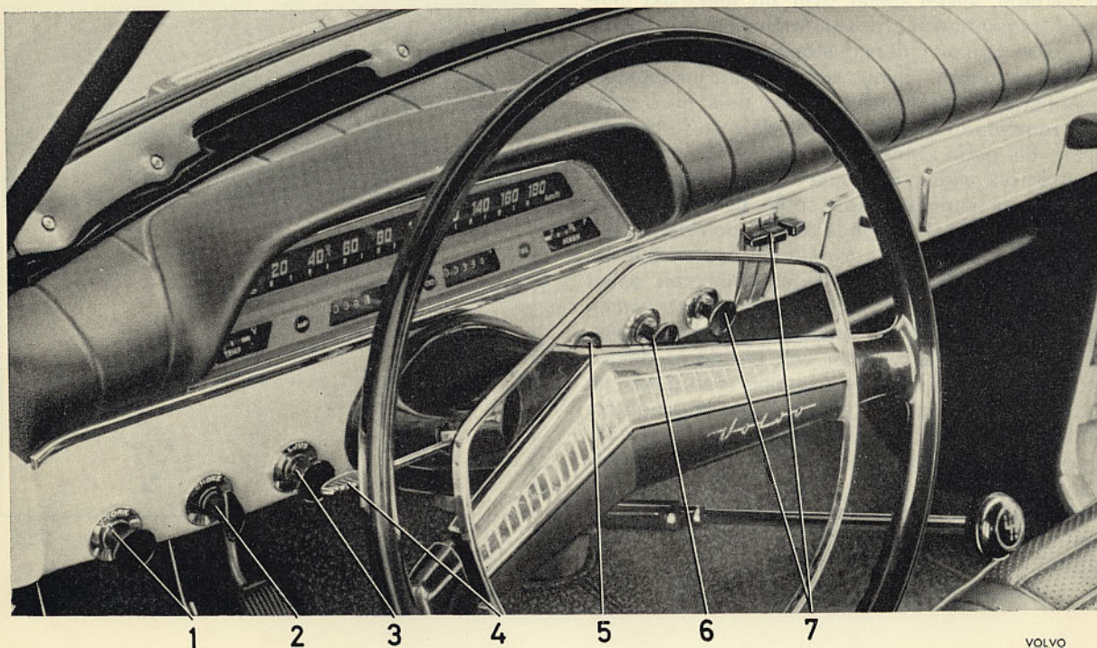
Bild 1. Instrument och manöverorgan
