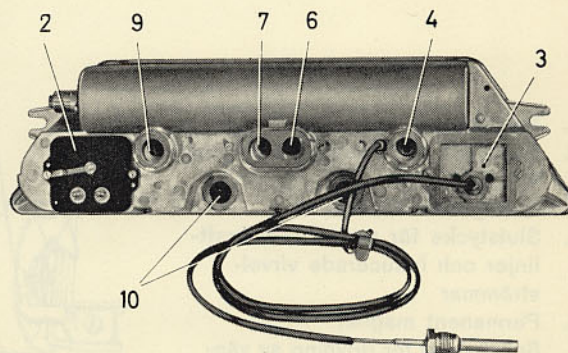
Bild 3. Kombinationsinstrument, baksida
