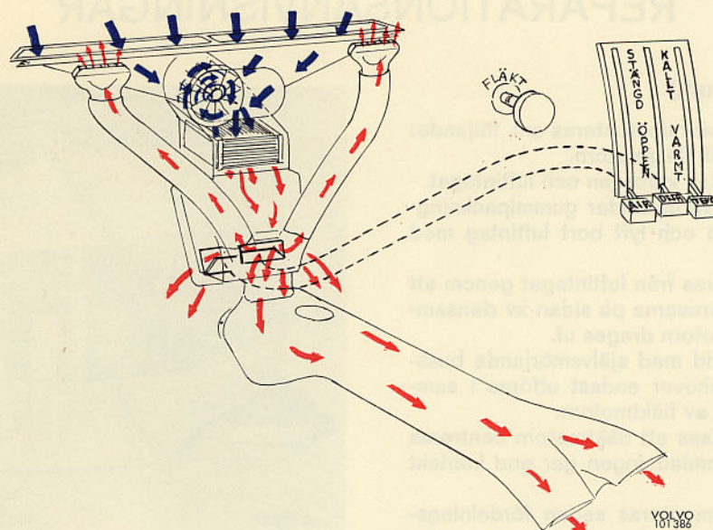
Bild 19. Värmesystemets uppbyggnad och funktion
