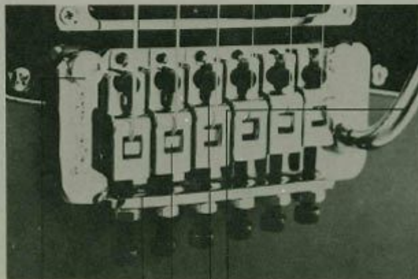
先端リアアクションを可能にしたアイブ メック。
