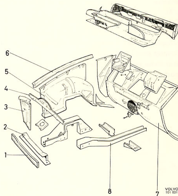
Bild 2. Torpedparti
