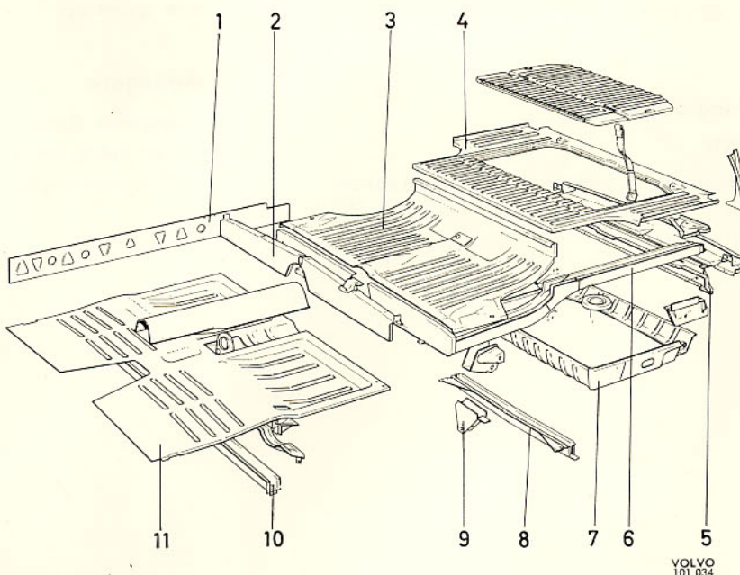
Bild 8. Golvparti, Herrgårdsvagn
