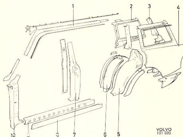
Bild 9. Sidoparti, Herrgårdsvagn
