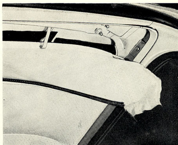
Bild 42. Takklädsel lossas för övre bakluckans gångjärnsmuttrar
