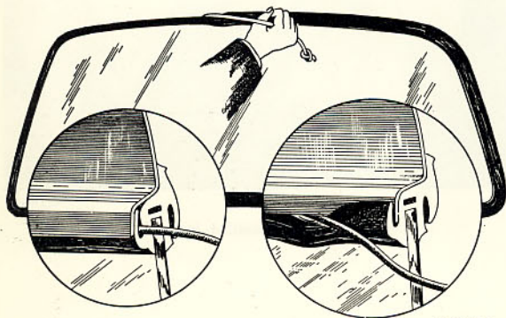
Bild 61. Montering av ruta
