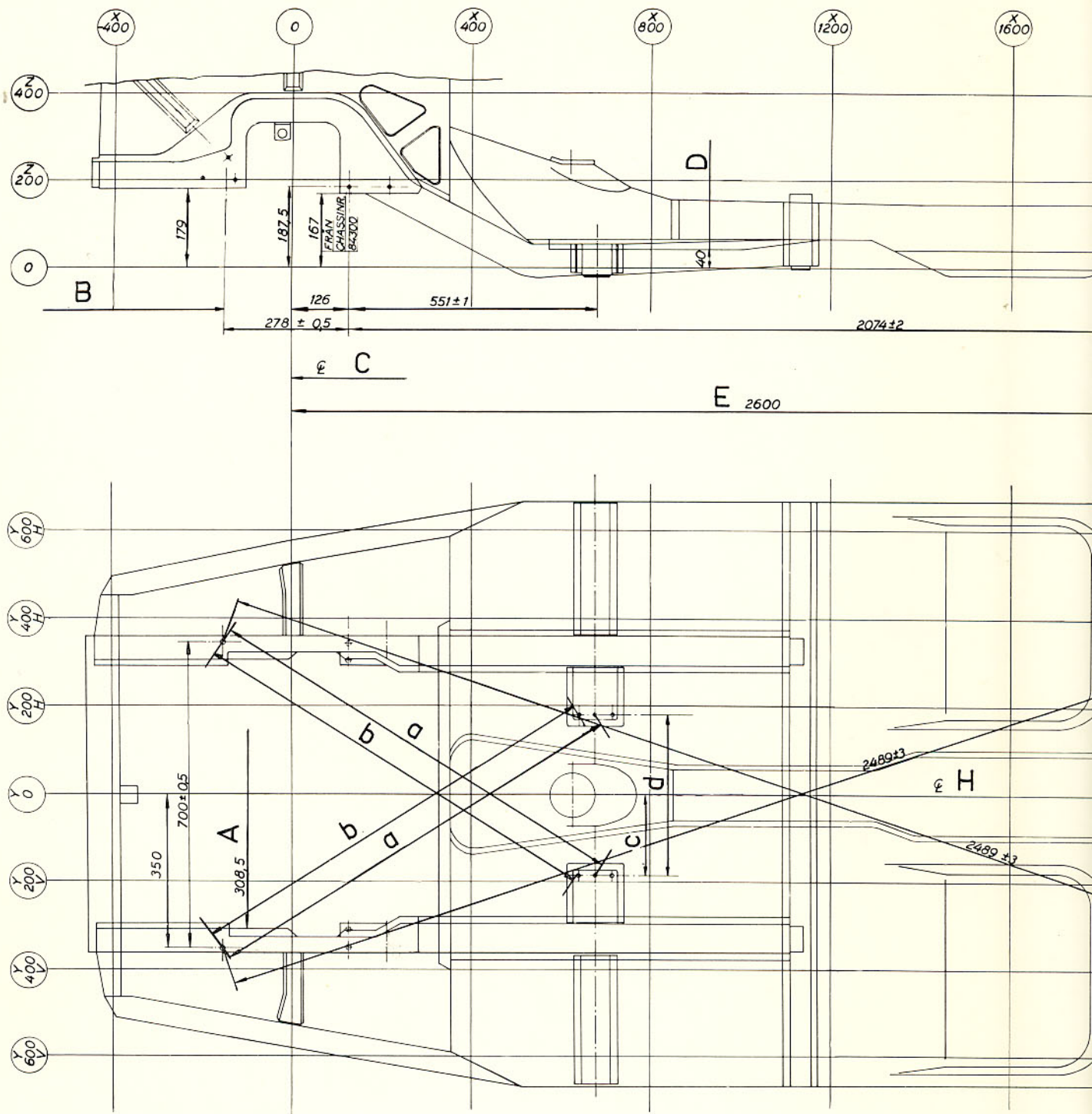
Plansch A. Kontrollritning för kaross t.o.m. chassinummer 4-dörrars 2250
