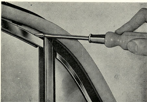
Bild 33. Övre styrlist lossas
