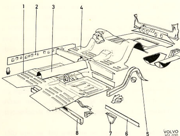
Bild 1. Golvparti (2- och 4-dörrars)
