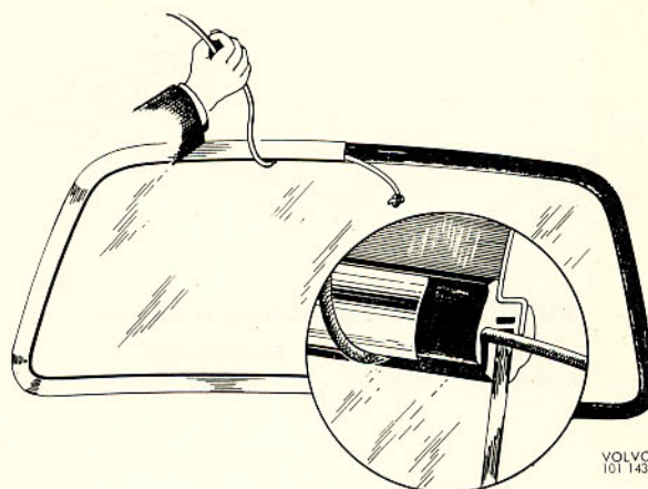
Bild 56. Montering av prydnadslist
