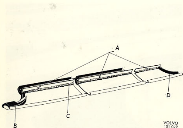
Bild 46. Bältlist
