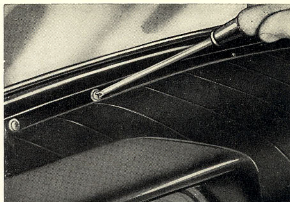
Bild 77. Demontering av prydnadslist för vindruta
