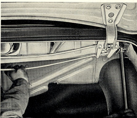
Bild 39. Torsionsstaven demonteras
