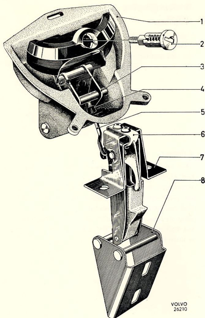
Bild 41. Lås för bagagelucka, sen. utf.
