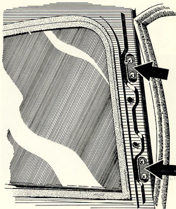
Bild 63. Fäste för bakre ventilationsruta
