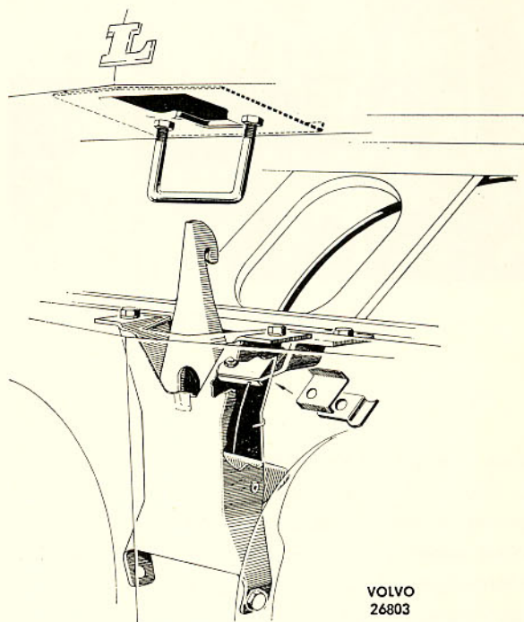
Bild 12. Huvlås, tid. utf.
