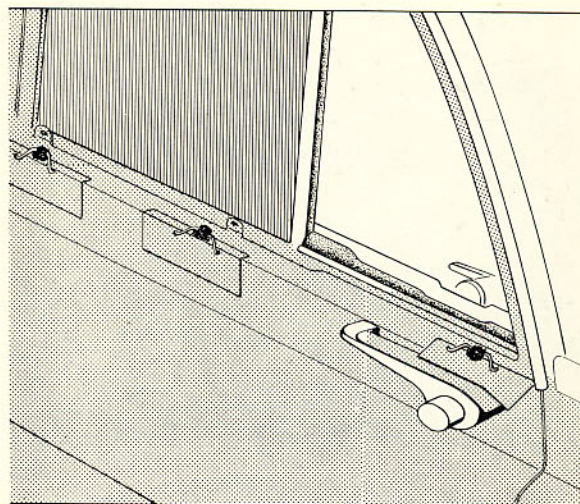
Bild 50. Placering av fjädrar
