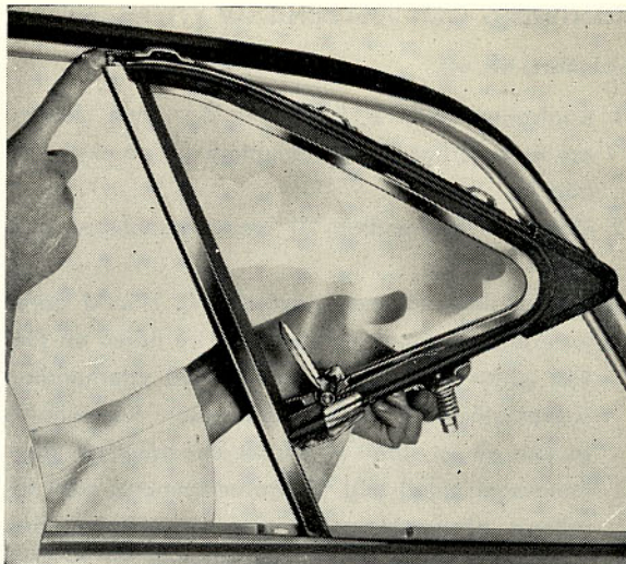
Bild 34. Ventilationsrutan lyftes ur
