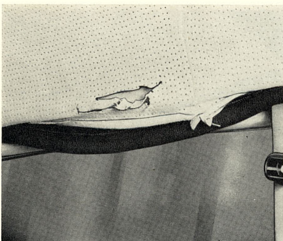
Bild 68. Takklädsel och kederlist lossade
