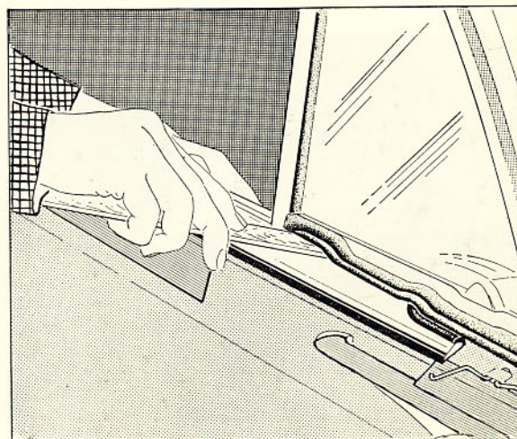
Bild 51. Montering av bältlist
