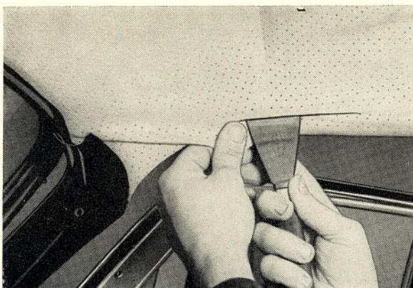
Bild 76. Takklädsel sträckes och fästes på hajlist
