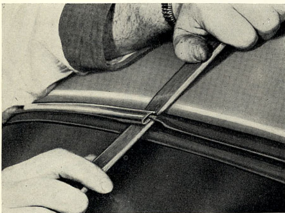
Bild 54. Prydnadslist lossas ur gummilist
