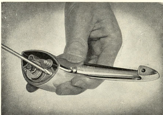
Bild 23. Isärtagning av låshandtag
