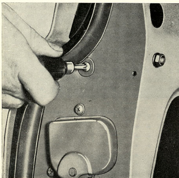
Bild 21. Övre skruv för styrskena lossas
