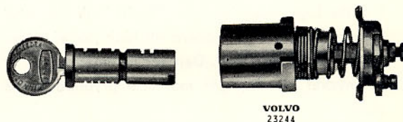
Bild 25. Tryckknappen isärtagen
