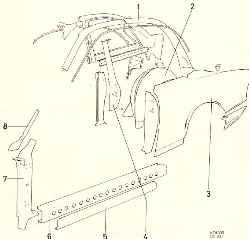
Bild 6. Sidoparti (2-dörrars)
