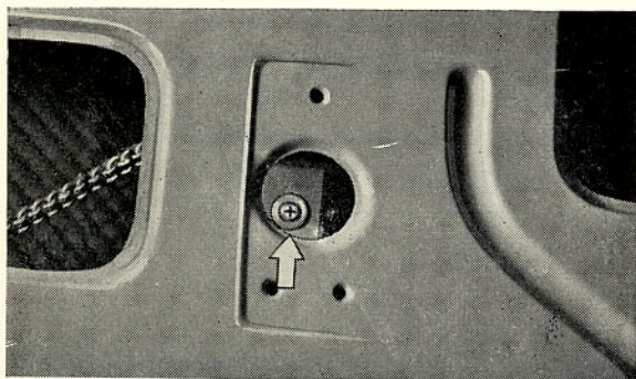
Bild 32. Fästskruv för hissrutans styrskena
