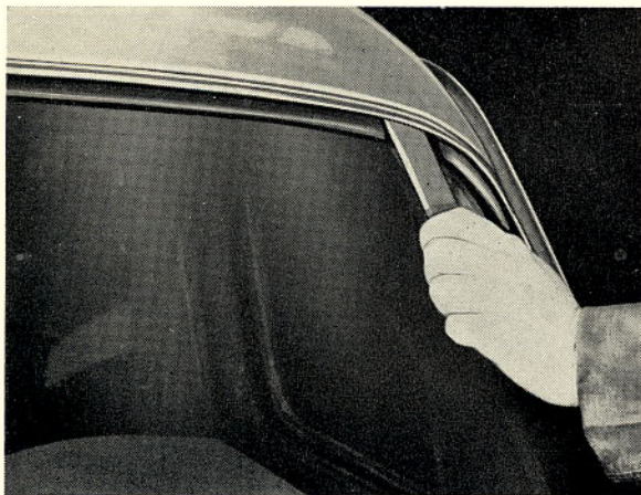
Bild 53. Prydnadslist lossas
