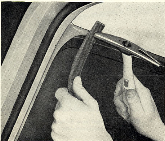
Bild 45. Hålllisten justeras
