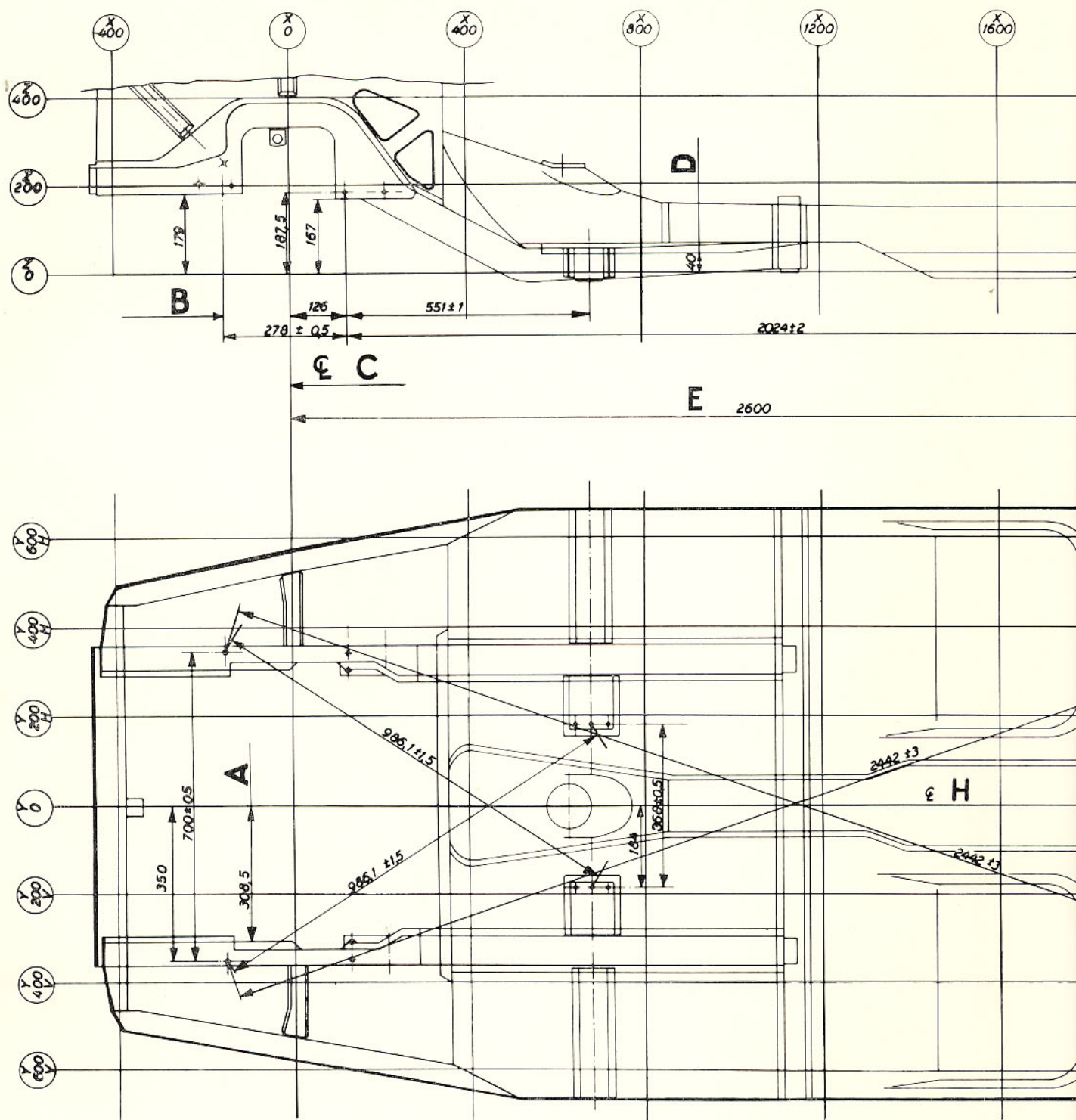
Plansch B. Kontrollritning för kaross fr.o.m. chassinummer 4-dörrars 2250
