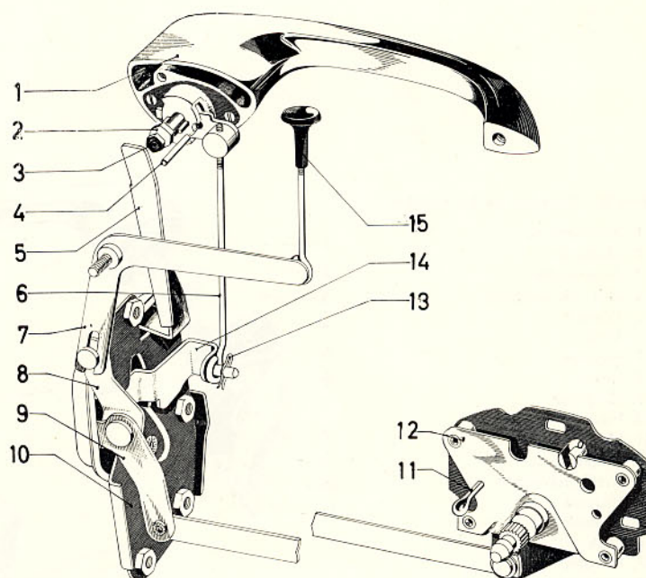
Bild 26. Justering av lås, framdörr
