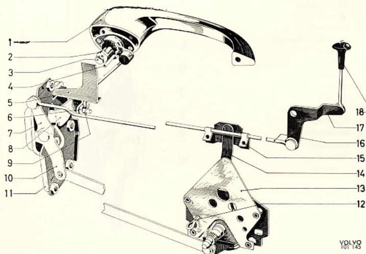
Bild 27. Justering av lås bakdörr
