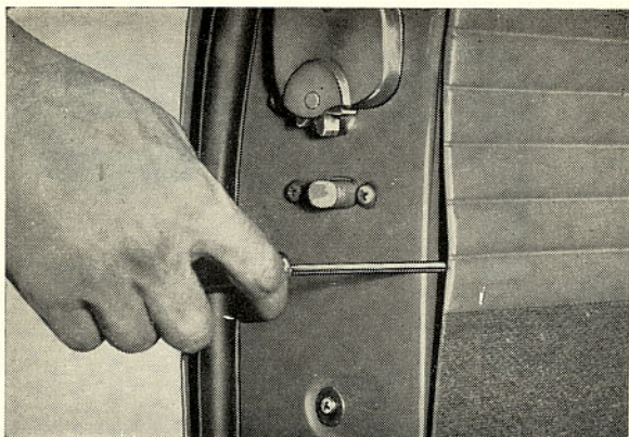
Bild 20. Demontering av dörrklädsel
