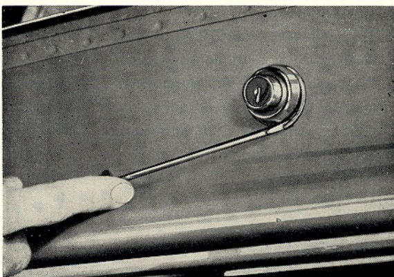
Bild 40. Låsring för låstryckknappen lossas
