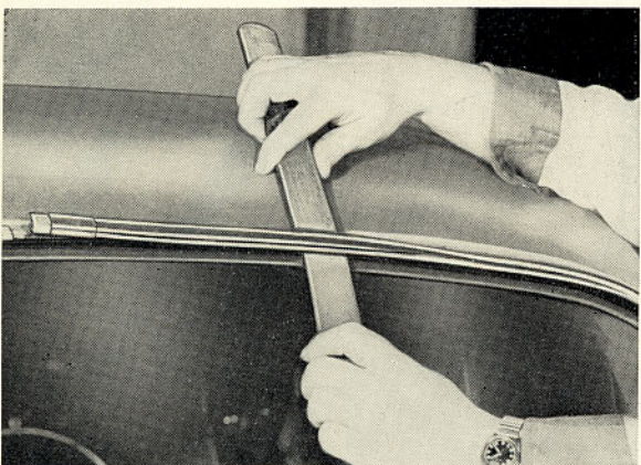
Bild 55. Demontering av prydnadslist
