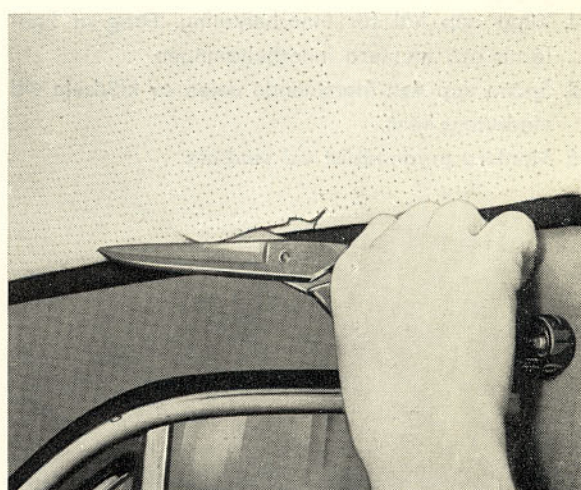
Bild 72. Takklädsel klippes ned
