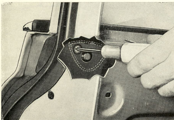
Bild 22. Låshandtag lossas
