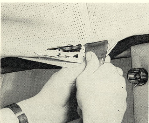
Bild 69. Takklädsel sträckes
