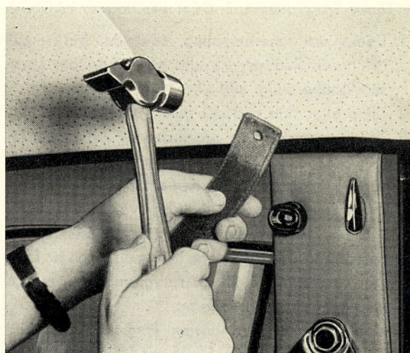
Bild 70. Justering av hajlist
