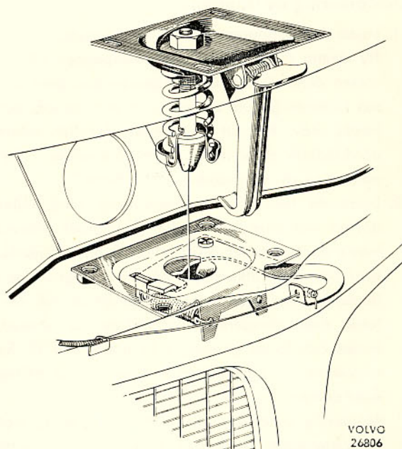
Bild 13. Huvlås, sen. utf.
