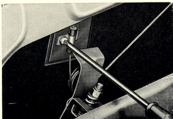
Bild 35. Överfall till medbringare lossas
