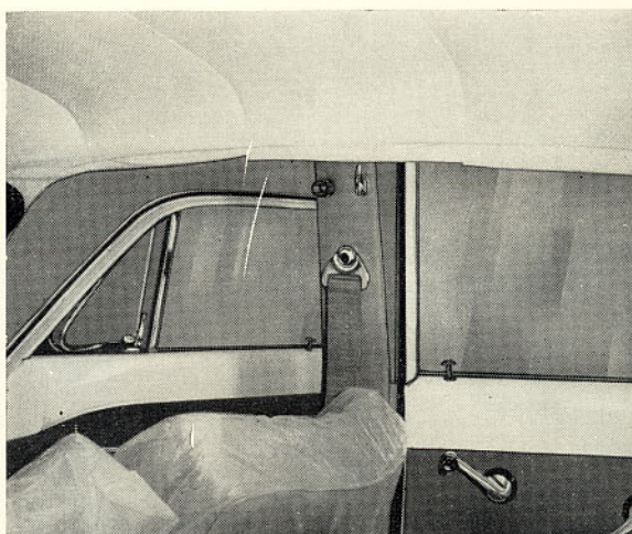
Bild 75. Takklädsel klar för sträckning
