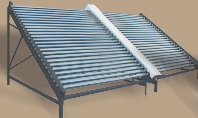
dạng dàn đôi ống thu nhiệt chân không lõi đỏ
