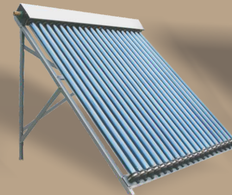
dạng dàn đơn ống thu nhiệt chân không lõi đỏ
