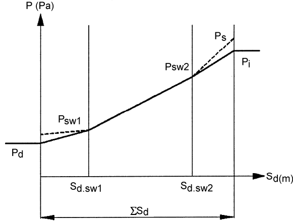
Şekil F.6 - Yapı elemanı içerisinde yüzey boyunca yoğuşma olduğu durumdaki su buhar difüzyonu
