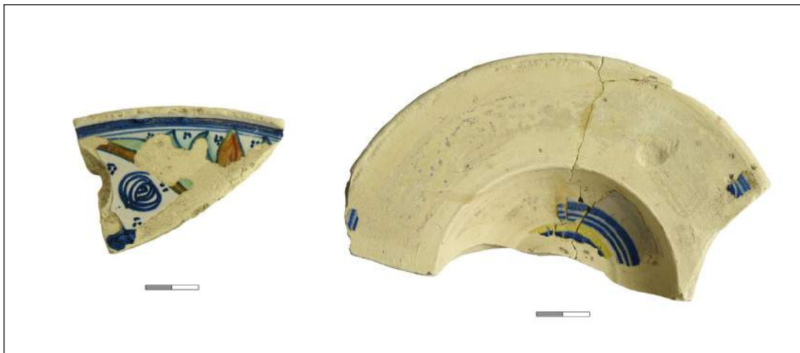
Afb. 49. Scherven van twee borden van majolica uit Montelupo, Italië (87-C01 en 79-C07). Het glazuur van het tweede bord is afgebladderd door vorstschade.
