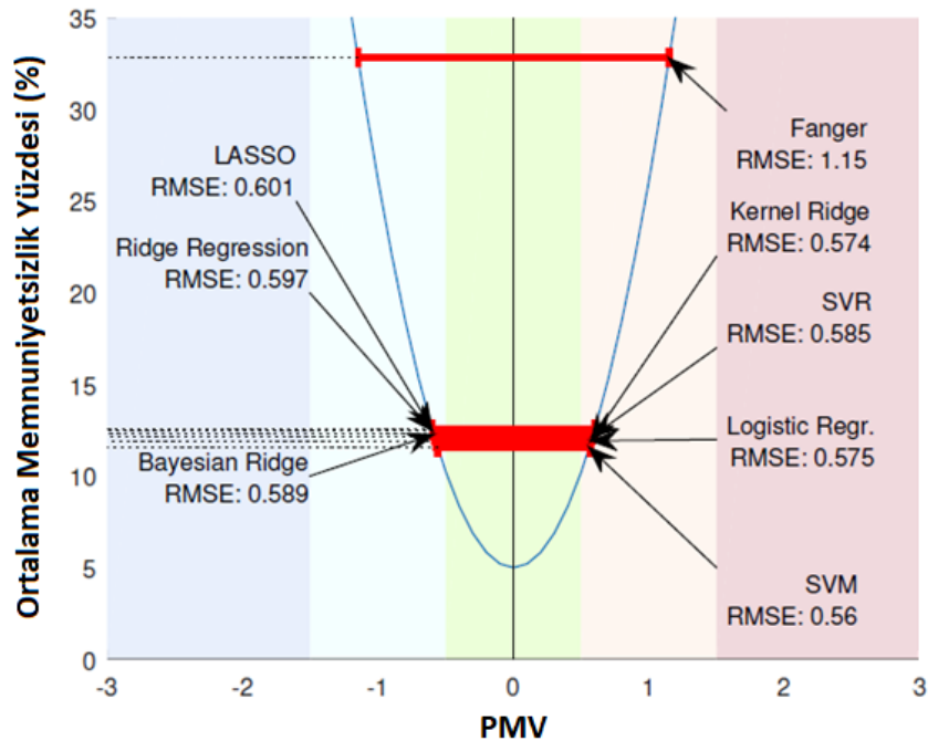
Şekil 8. Isıl konfor modellerinde ortalama hatalarının kare ortalamalarının kökünün (RMSE), Fanger modelinin PPD değerleri ile karşılaştırılması [38].
