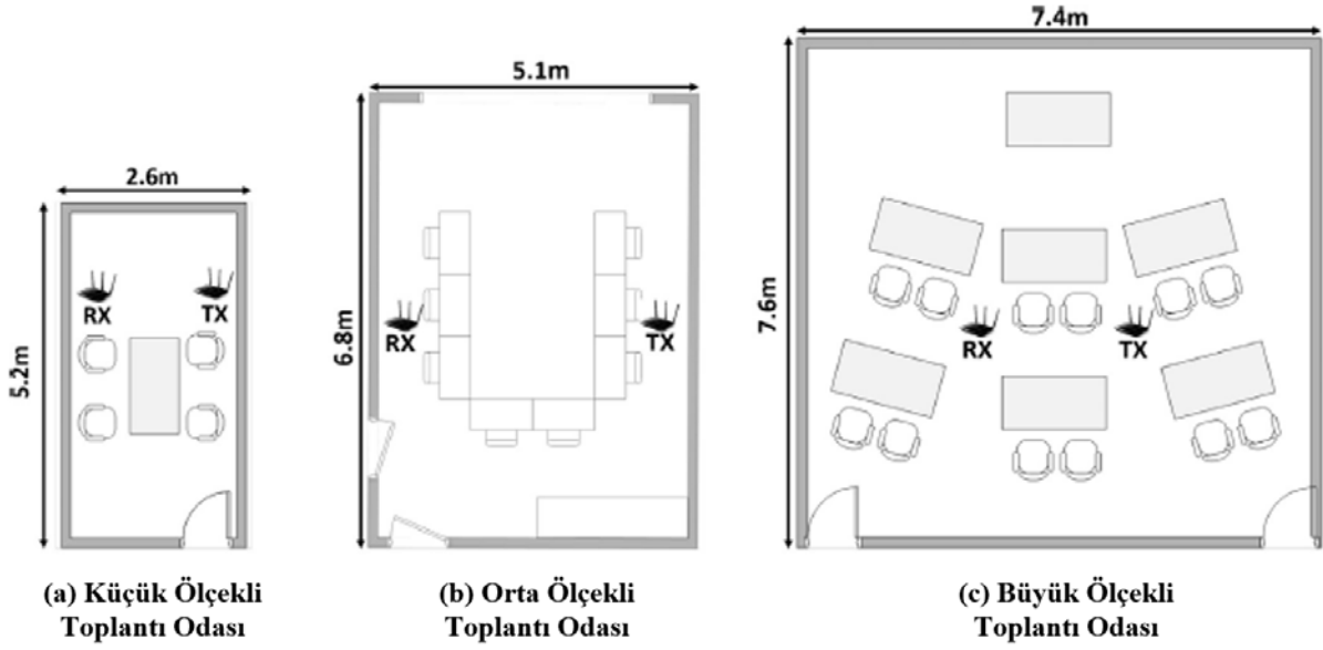
Şekil 3. Algılama testlerinde kullanılan oda tipleri ve ölçüleri.
