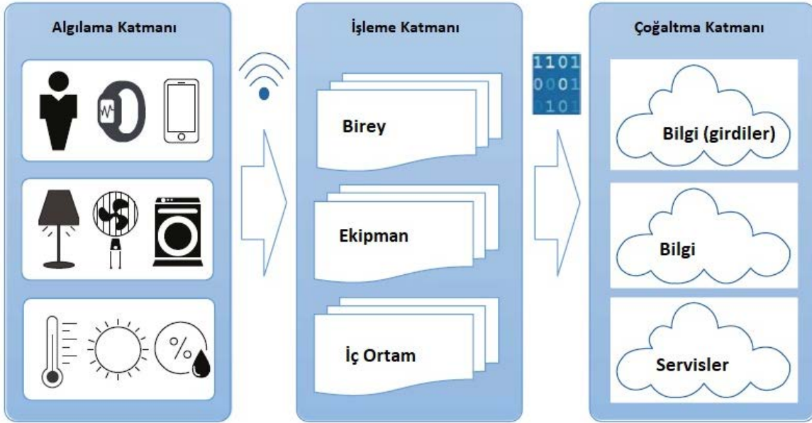
Şekil 9. Akıllı binalarda nesnelerin interneti tabanlı platform mimarisi [39].
