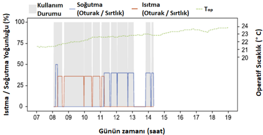
Şekil 13. Kişisel ısı konfor sistemli ofis koltuğu veri grafiği [27].
