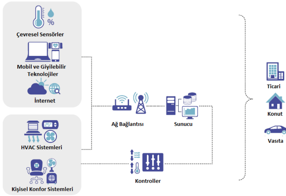
Şekil 5. Kullanıcı odaklı çevresel kontrol sistem mimarisi[26].
