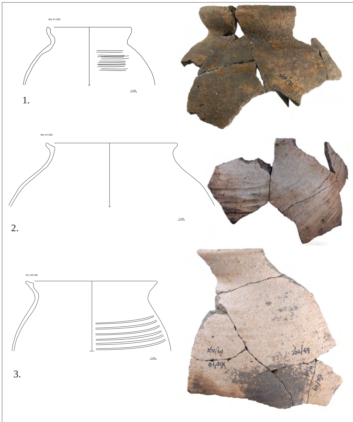
Afbeelding 32. Voorbeelden van kogelpot type 1 (kp-kog-1). Schaal getekend 1:4, foto ca. 1:2.
