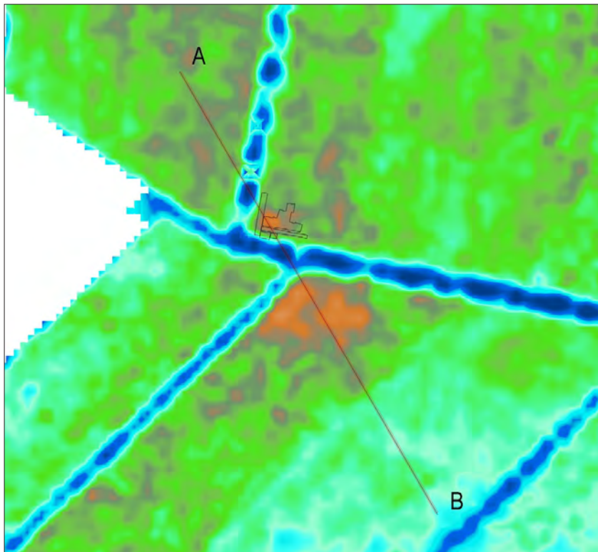
Afbeelding 71. Uitsnede van het AHN in de omgeving van de onderzoekslocatie. De werkputten zijn weergegeven. De rode en oranje delen zijn hoog. De groene en blauwe delen zijn lager. De letters AB en de lijn daartussen geven de locatie van de hoogte-opnamen in afbeelding 72 weer.
