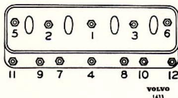
Ätdragningsföljd för cylinderlocksmuttrar, motor B 16
