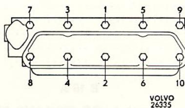
Åtdragningsföljd för cylinderlocksskruvar, motor B 20
