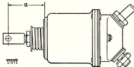
Inställning av manövermagnet (järnkärnan indragen)
