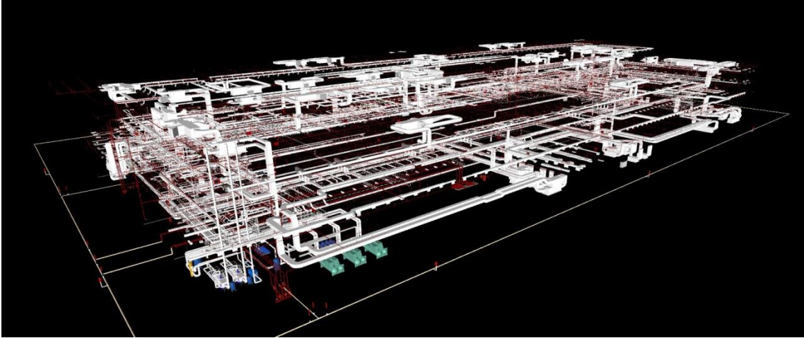
Şekil 12. Havalimanı projesi mekanik tesisat modeli
