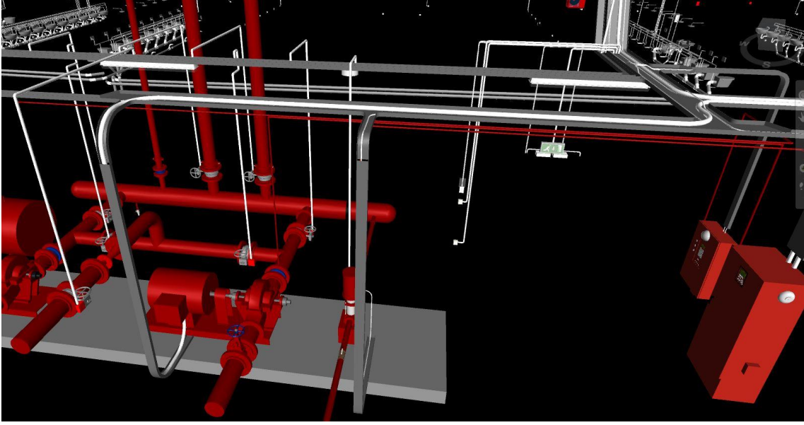
Şekil 13. Havalimanı projesi yangın pompa odası modeli
