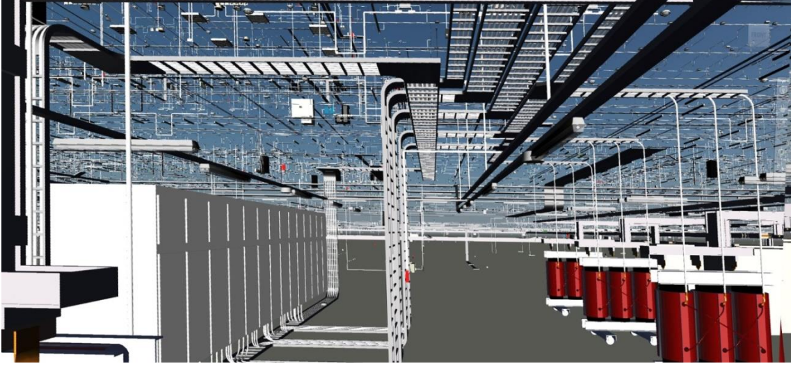
Şekil 11. Havalimanı projesi elektrik tesisatı modeli
