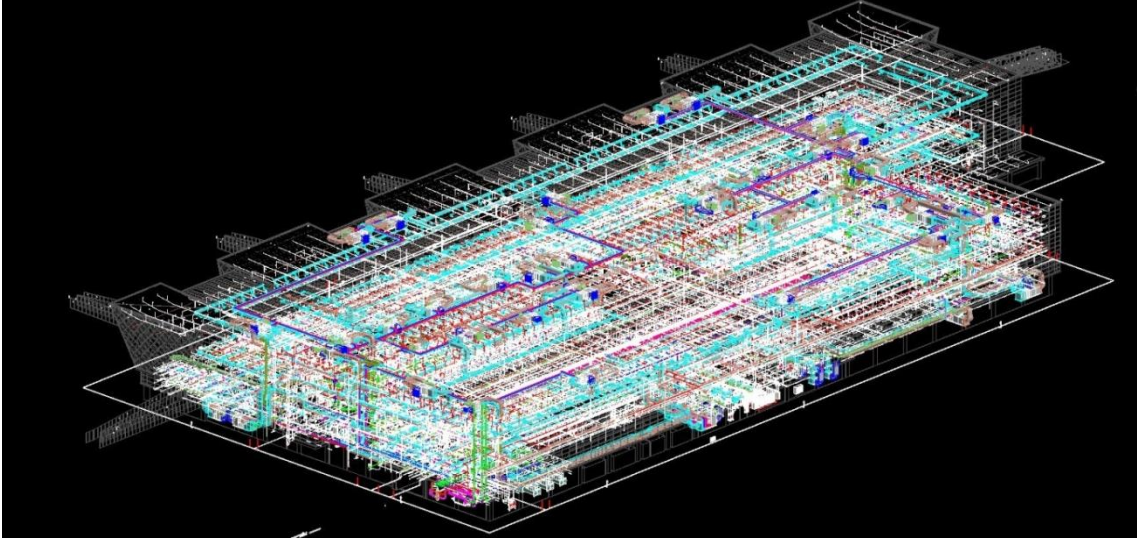
Şekil 10. Havalimanı Projesi MEP Koordinasyon Modeli
