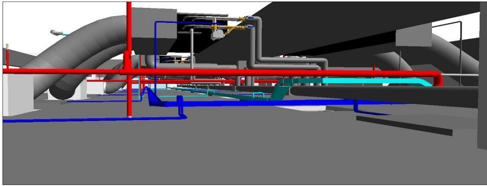
Şekil 6. Koordine edilmiş asma tavan görünüşü [7]
