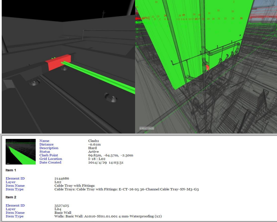
Şekil 5. Çakışma kontrolleri ve raporlanması
