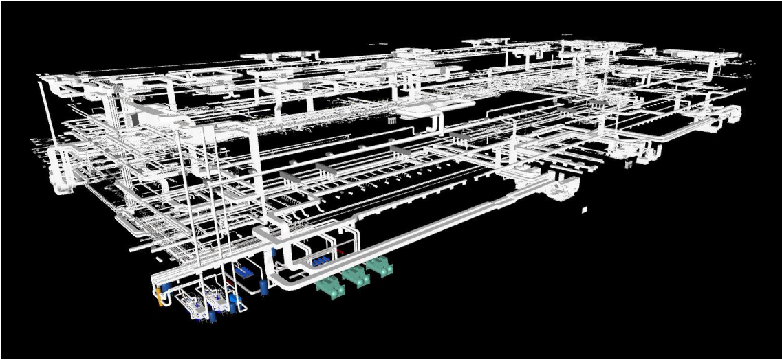
Şekil 14. Havalimanı projesi iklimlendirme tesisatı modeli
