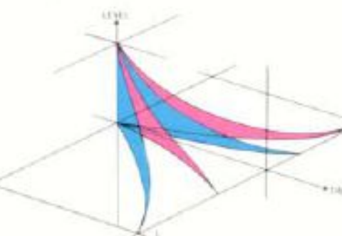
2) Simulation eines Nachhalls beim SDR 1000 (Mono-Eingangssignal)
