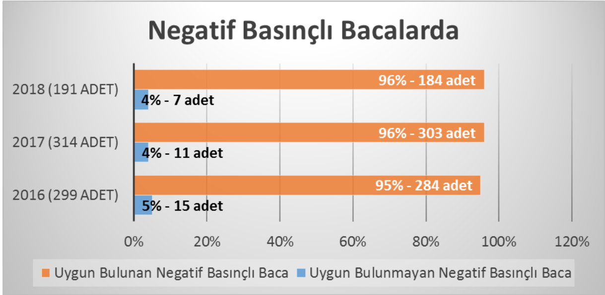
Şekil 5. Negatif Basıncılı Bacalar için Sızdırmazlık Testlerindeki Uygunluk Oranları
