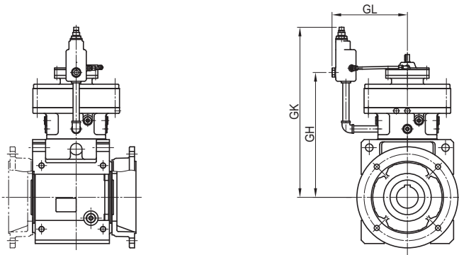
Solid Shaft 4A10DA~4E18DB
