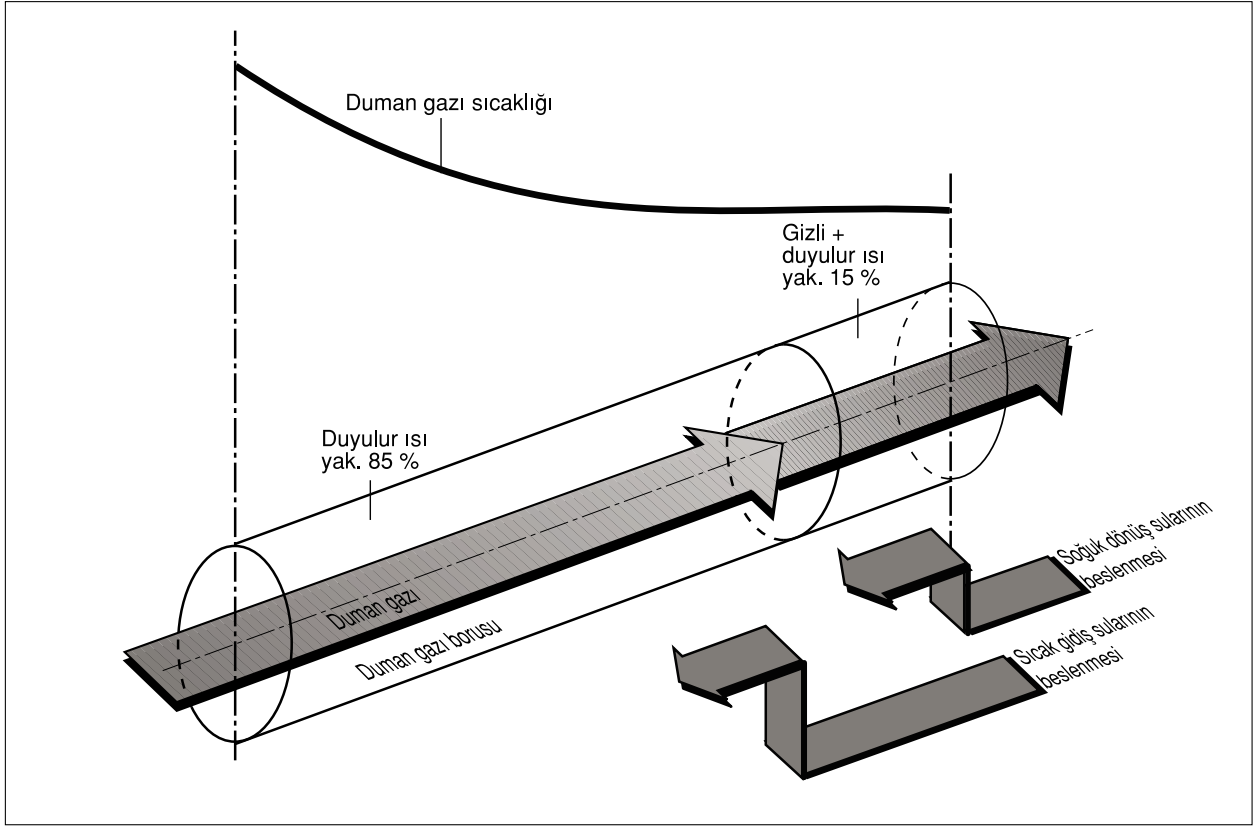
Şekil 3.55 / DÜŞÜK SICAKLIĞI SAHİP DÖNÜŞ SULARININ AYRI OLARAK BESLENMESİ
