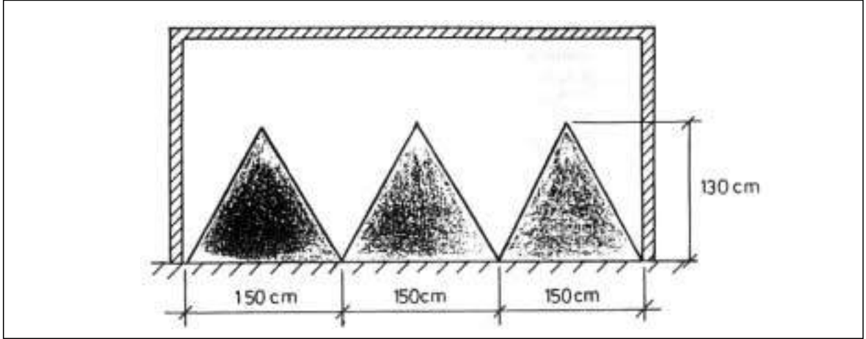
Şekil 5.4 a/ KÖMÜRÜN KAPALI DEPOLANMASI
