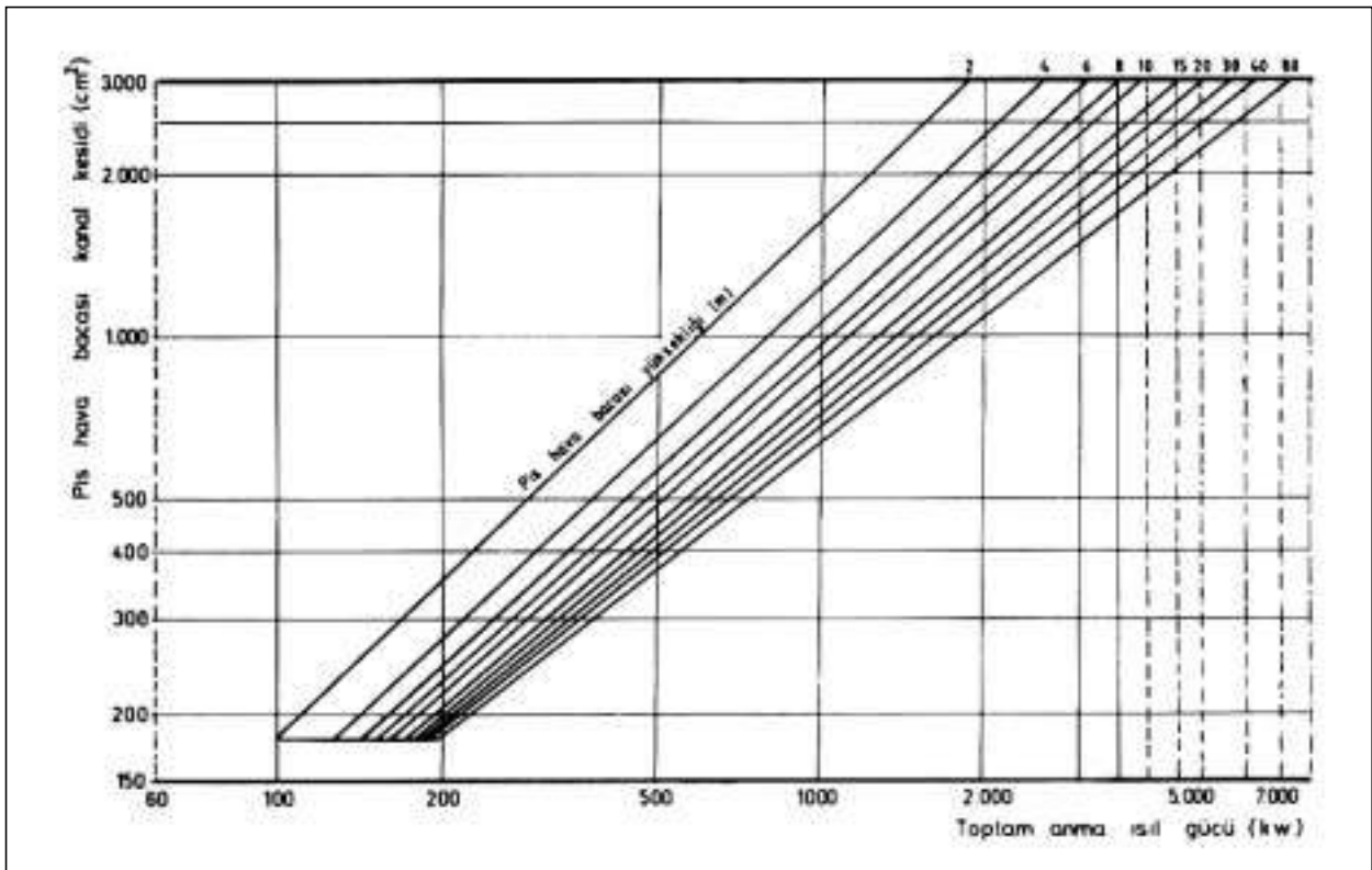
Şekil 9.4 / PİS HAVA BACASI BOYUTLANDIRMASI
