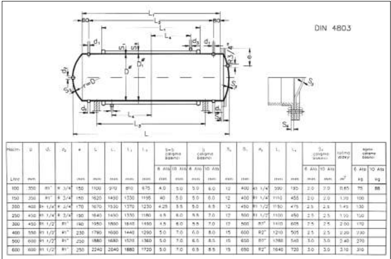
Şekil 5.76/ ÇİFT ÇİDARLI BOYLER
