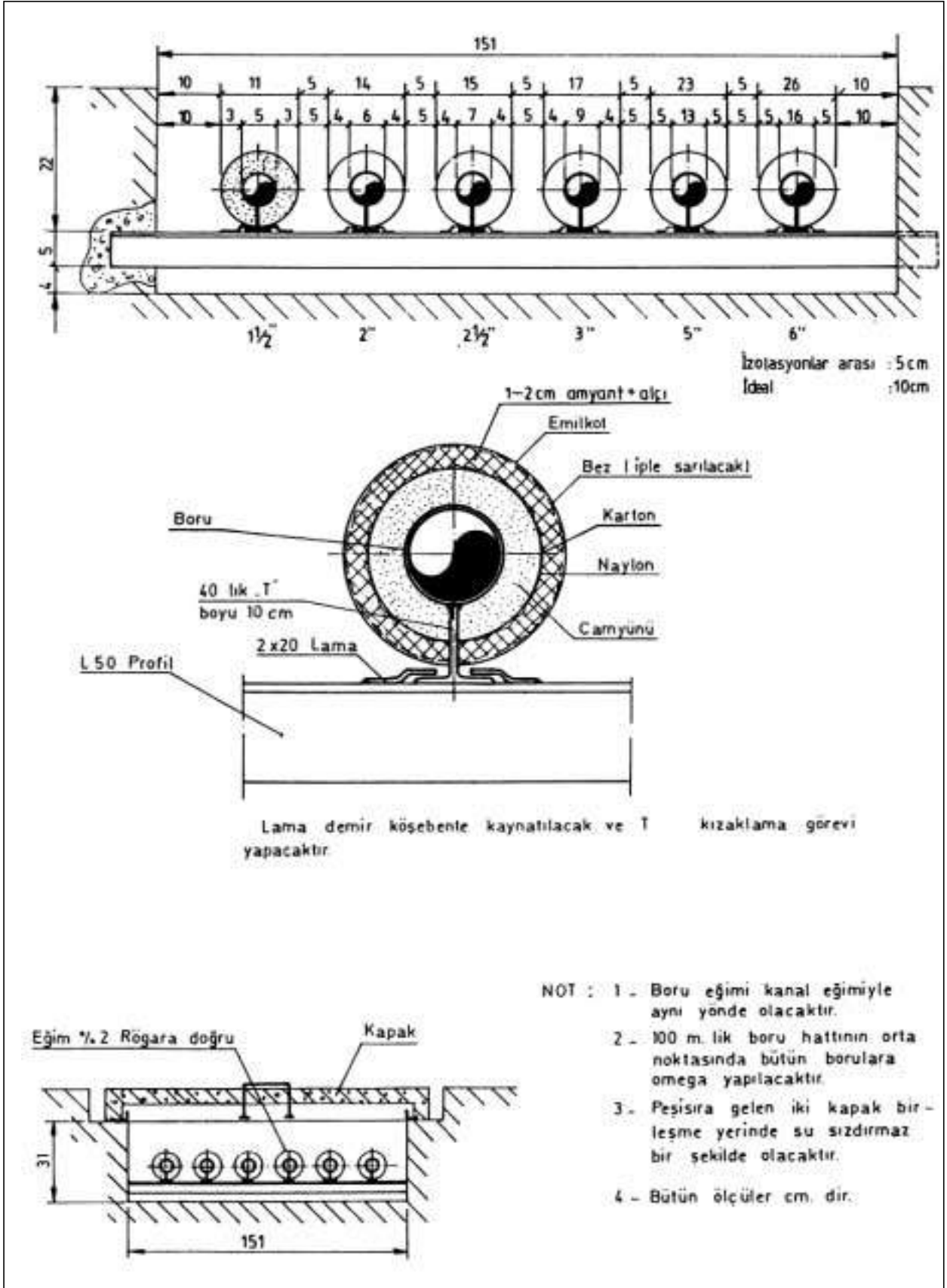
Şekil 7.7 / BORU YERLEŞİMİ
