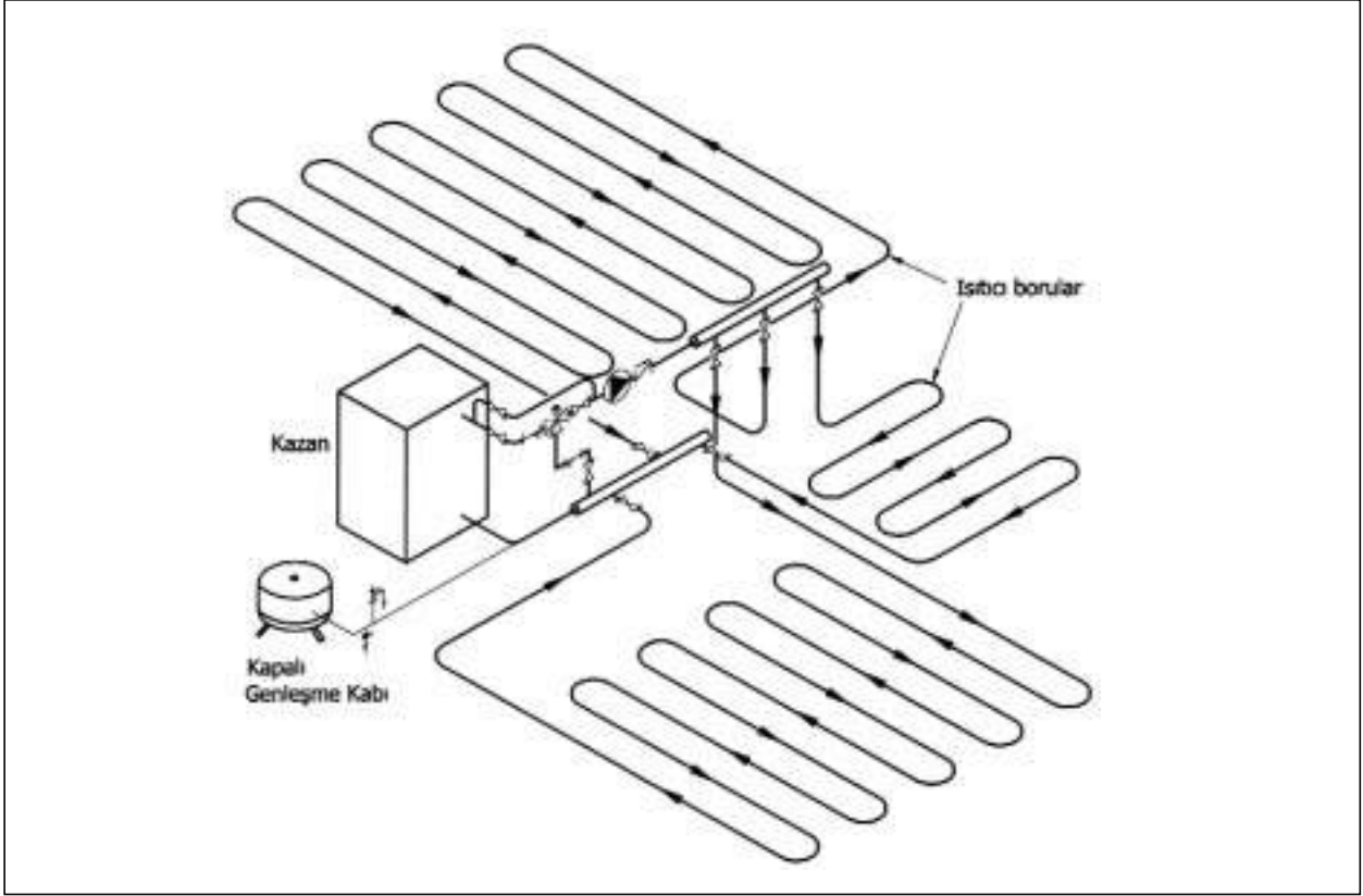
Şekil 4.40 / DÖŞEMEDEN ISITMA TESİSATI
