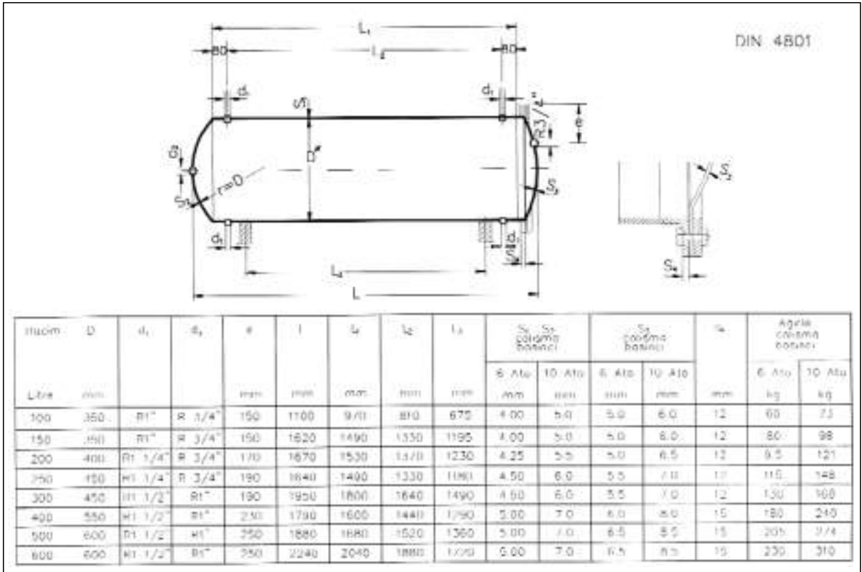
Şekil 5.78/ TEK ÇİDARLI BOYLER (Serpantin eklenecek)
