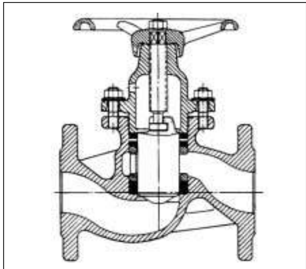
Şekil 7.34 / BUHAR VANASI (GLOBE VANA)
