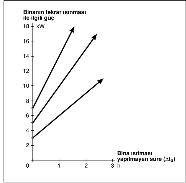
Şekil 3.18/ BİNANIN TEKRAR ISINMASI İÇİN GEREKEN GÜÇ, BİNA ISITILMASI YAPILMAYAN SÜREYE GÖRE
