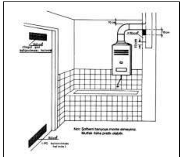
Şekil 10.25 / HAVALANDIRMALI BACAYA BAĞLANTI DETAYI
