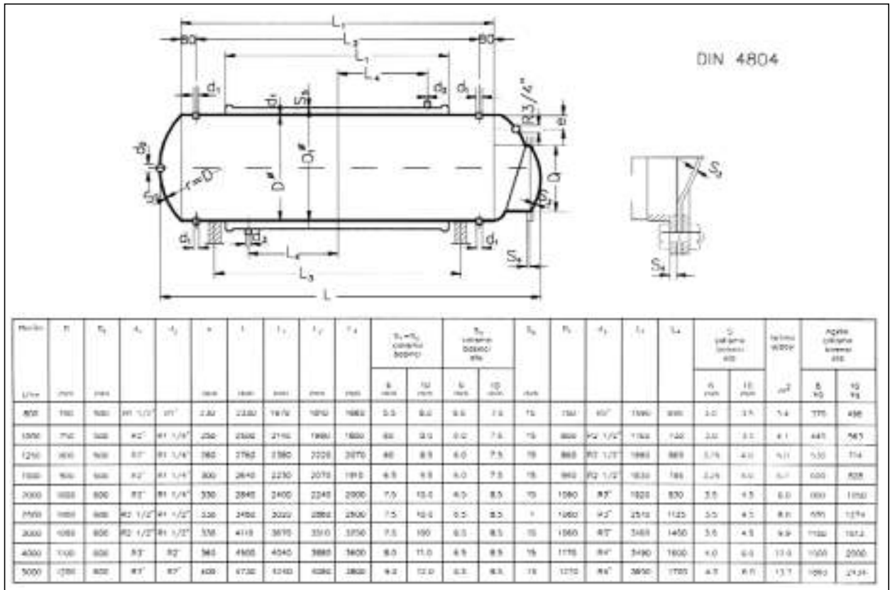
Şekil 5.77/ ÇİFT ÇİDARLI BOYLER
