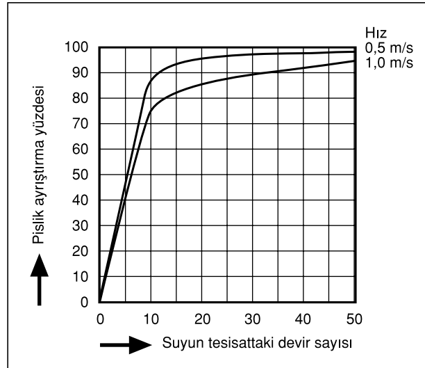
Şekil 6.58/ SPİROVENT PİSLİK AYIRMA ETKENLİĞİ
