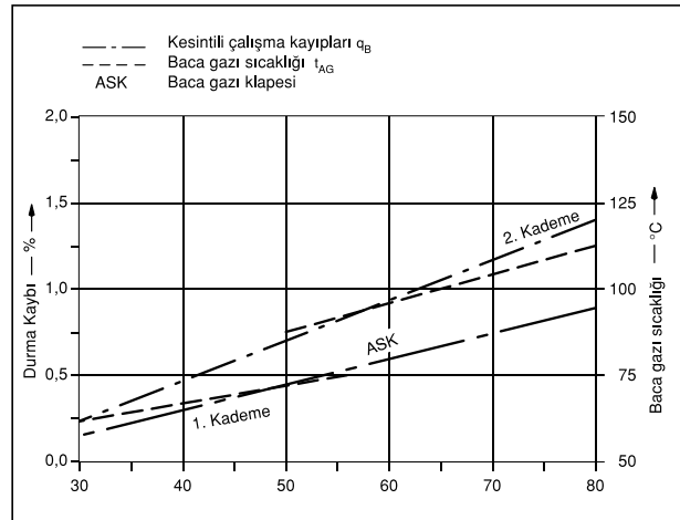
Şekil 5.7/ KESİNTİLİ BACA GAZI KAYIPLARI VE BACA GAZI SICAKLIĞI KAZAN SUYU SICAKLIĞINA BAĞLIDIR. (Baca gazı sıcaklığı davlumbazdan ölçülmüştür)
