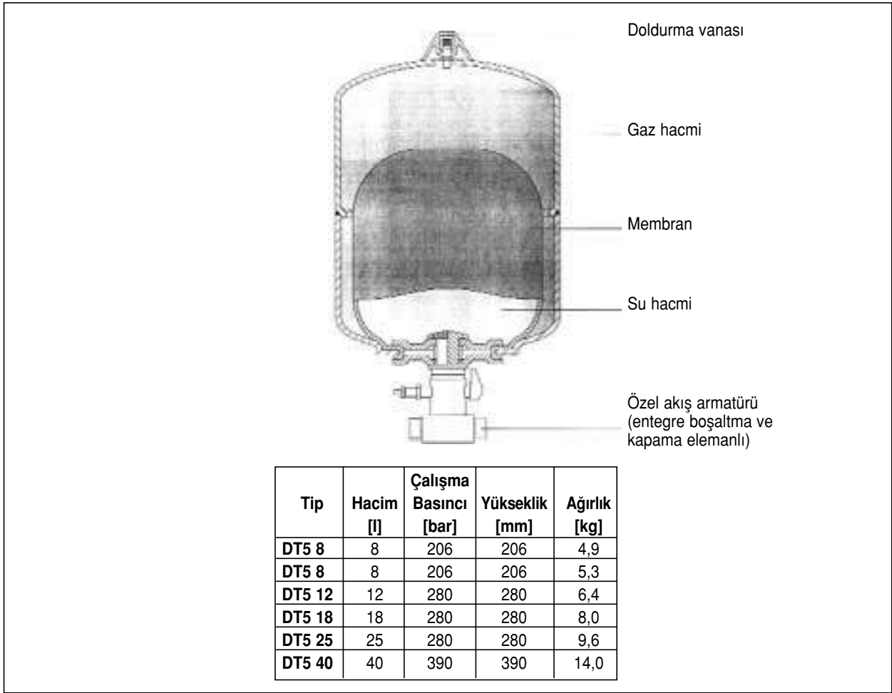
Şekil 6.44/ DT5 KAPALI GENLEŞME KABİ
