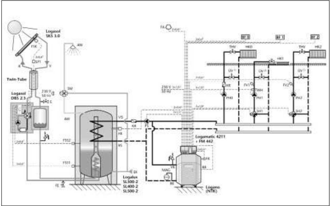
Şekil 4.48/ DÖŞEME TİPİ KAZANLA TAKVİYELİ GÜNEŞ ENERJİSİYLE KULLANMA SICAK SUYU ISITMA SİSTEMİ
