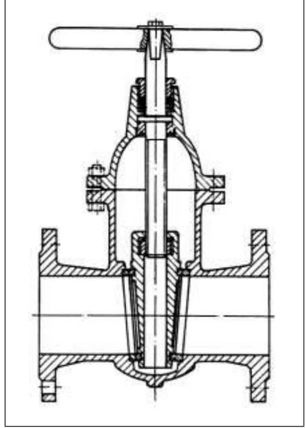
Şekil 7.45 / SÜRGÜLÜ VANA
