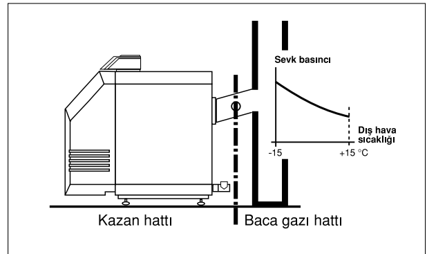
Şekil 3.57 / KAZAN VE BACA GAZI HATLARI BİR FONKSİYON BİRİMİ OLUŞTURMAKTADIR.
