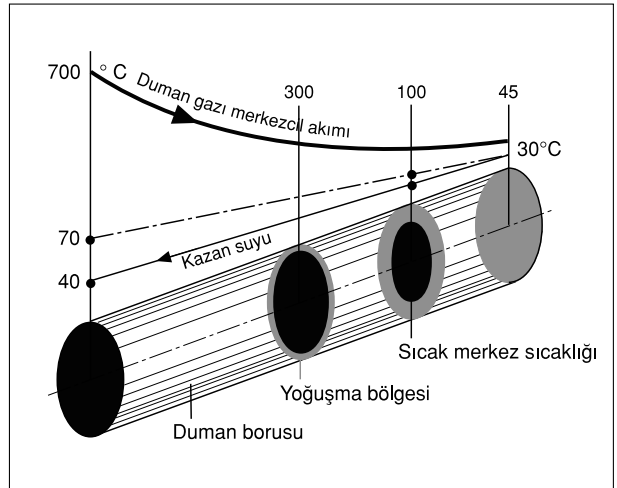
Şekil 3.44 / DUMAN GAZI VE KAZAN SUYUNUN ZIT YÖNLÜ PARELLEL AKIMI KONDENS OLUŞUMUNU İYİLEŞTİRMEKTEDİR. KAZAN DÖNÜŞ SUYU SICAKLIĞI BELİRLEYİCİDİR.
