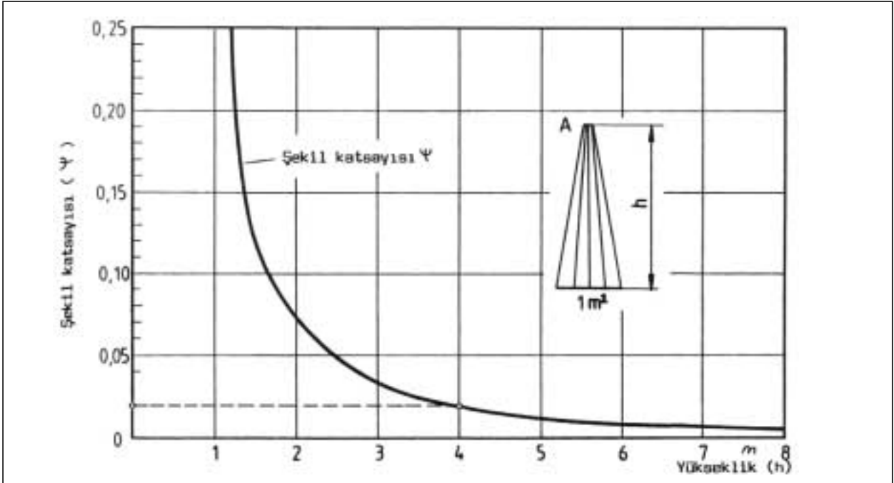
Şekil 6.20/ PARALEL İKİ DÜZ YÜZEY ARASINDAKİ ŞEKİL KATSAYISININ ARADAKİ h YÜKSEKLEĞİNE BAĞLI OLARAK DEĞİŞİMİ
