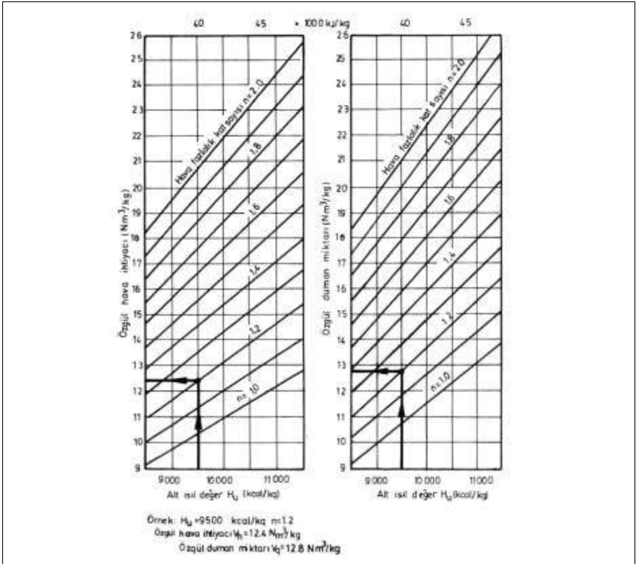
Şekil 5.53/ FUEL-OİL İÇİN ÖZEL HAVA VE DUMAN MİKTARLARI
