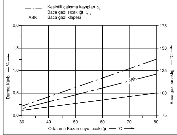
Şekil 5.6/ KESİNTİLİ BACA GAZI KAYIPLARI VE BACA GAZI SICAKLIĞI KAZAN SUYU SICAKLIĞINA BAĞLIDIR. (Baca gazı sıcaklığı davlumbazdan ölçülmüştür)
