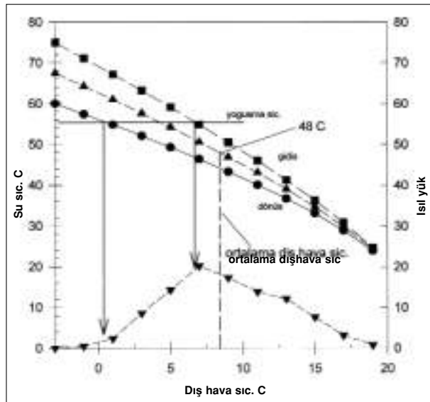
Şekil 3.30/ İSTANBUL KOŞULLARINDA DIŞ SICAKLIĞI GÖRE SU SICAKLIKLARI VE ISI YÜKÜ DAĞILIMI
