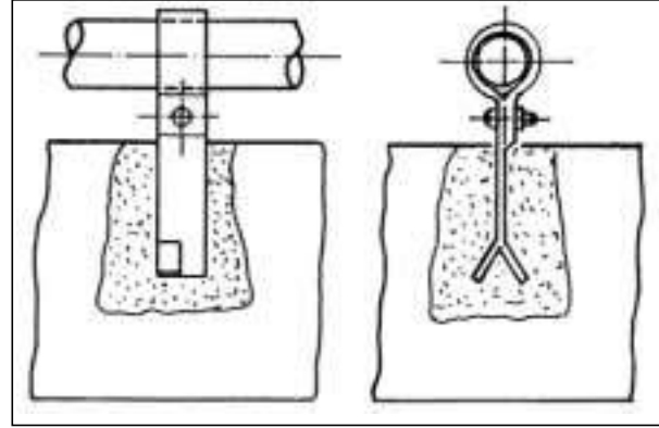
Şekil 7.9 / BORU KELEPÇESİ
