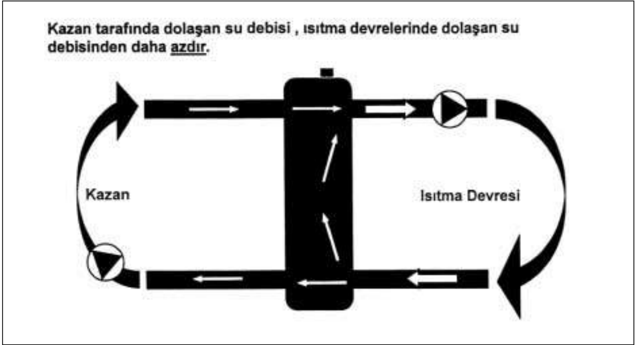
Şekil 5.18 d / DEBİLERİN EŞİT OLMAMASI HALİ
