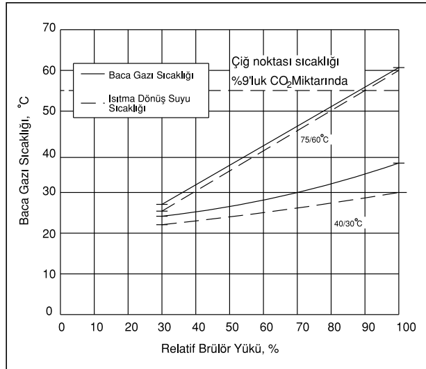
Şekil 5.27/ BACA GAZININ SICAKLIĞININ YÜKE BAĞLILIĞI
