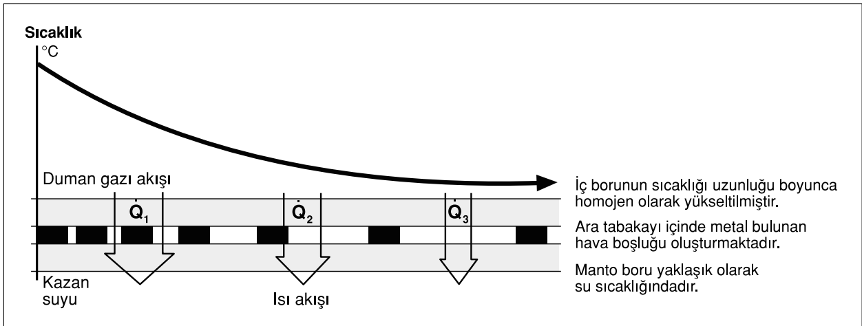
Şekil 3.38 / ISI AKIŞININ COMPOSIT - DUMAN BORUSU İÇİNDE DUMAN GAZI AKIŞI BOYUNCA AYARLANMASI
