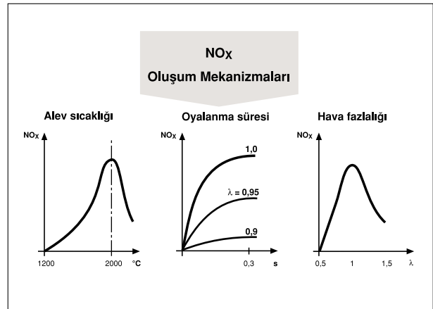
Şekil 3.60 / AZOT OKSİT OLUŞUMU MEKANİZMALARI
