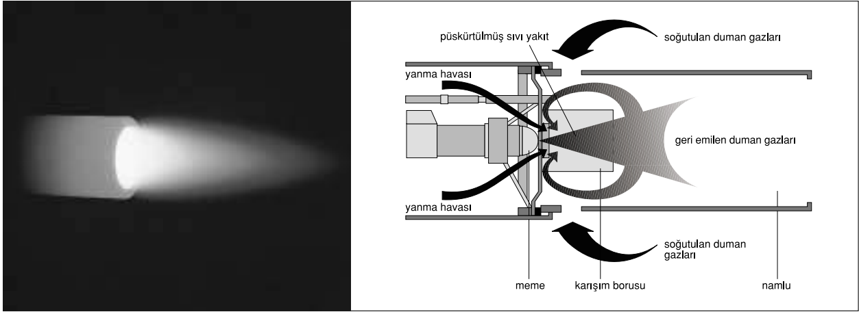
Şekil 3.59 / SIVI YAKIT MAVİ ALEVLİ BRÜLÖRÜN ÇALIŞMA PRENSİBİ
