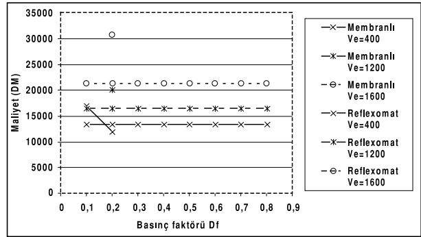
Şekil 6.41/ STATİK BASINÇ Pst=8 bar OLMASI HALİNDE REFLEXOMAT - MEMBRANLI KARŞILAŞTIRILMASI
