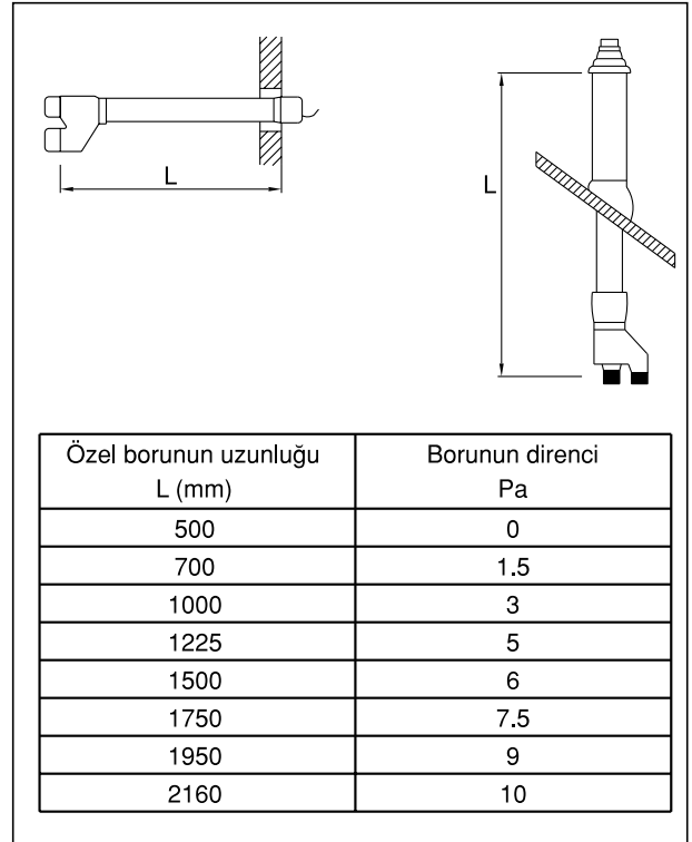
Şekil 5.14/ ÇİFT CİDARLI ÖZEL BORU DİRENÇ DEĞERLERİ
