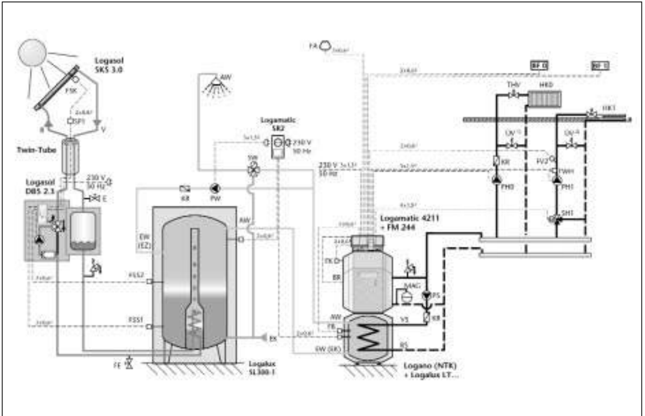
Şekil 4.51/ BOYERLİ ISITMA SİSTEMİNE DESTEK VEREN GÜNEŞ ENERJİ SİSTEMİ
