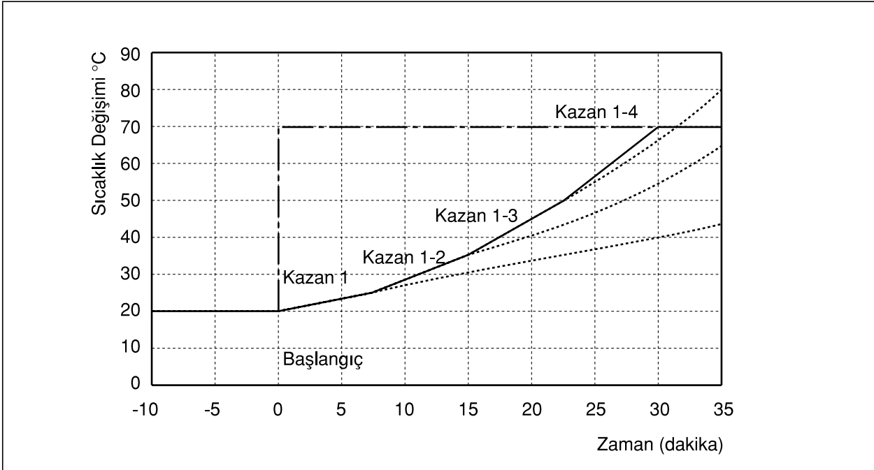
Şekil 5.39/ İLK ÇALIŞMA SIRASINDA SICAKLIK DEĞİŞİMİ
