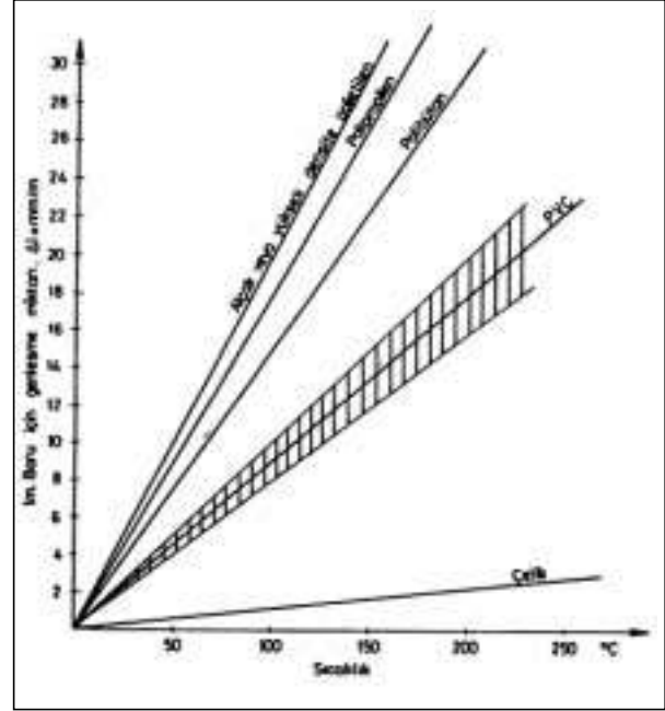
Şekil 7.18 / ÇELİK VE PLASTİK BORULARIN GENLEŞME MİKTARLARI
