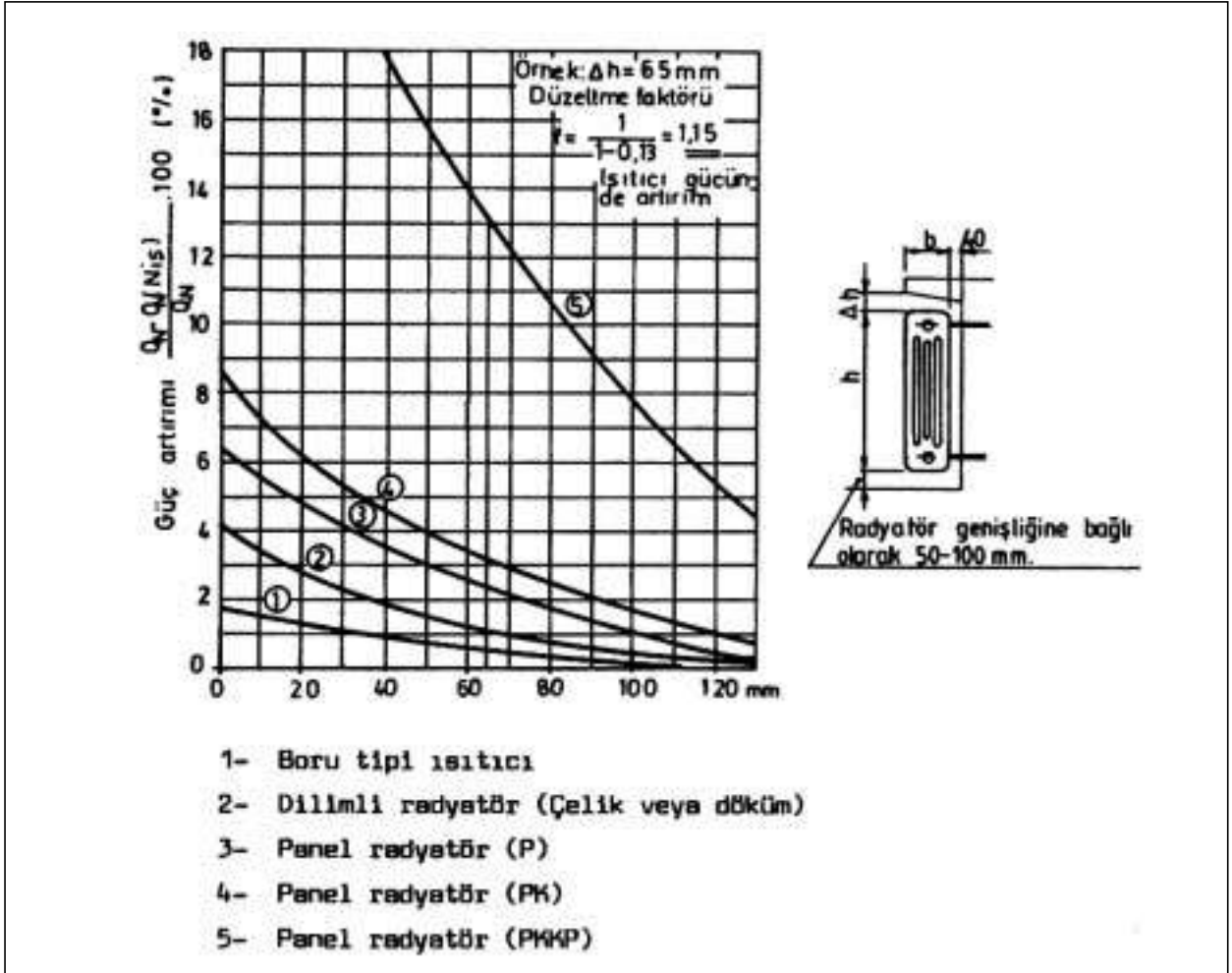
Şekil 6.5/ NİŞ İÇERİSİNE MONTE EDİLEN RADYATÖRLERDE, RADYATÖR ÜSTÜNDE KALAN MESAFEYE ( \Delta h ) BAĞLI OLARAK YAPILMASI GEREKEN KAPASİTE ARTTIRIMI (DIN 4703 bölüm 3)
