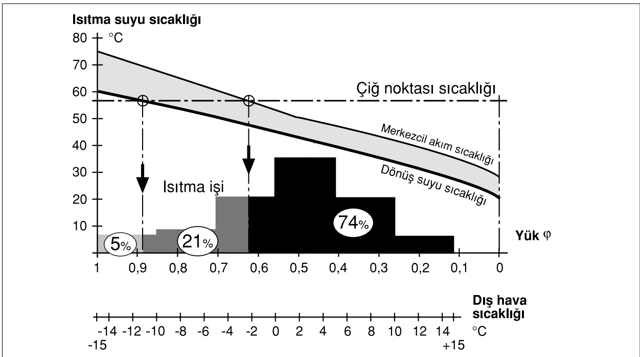
Şekil 3.47 / A YOĞUŞMASIZ DURUMDAKİ, KİSMİ VE TAM YOĞUŞMADAKİ ISITMA ZAMANI YÜZDELERİ, MODÜLASYONLU (ORANSAL) BRÜLÖRDE
