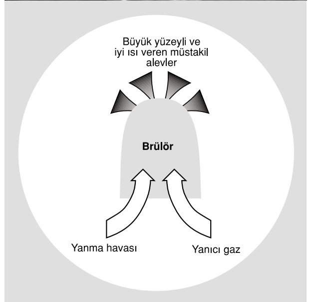
Şekil 3.62 / GAZ YAKITLI ÖN KARIŞIMLI BRÜLÖR, ÇOK SAYIDA MÜSTAKİL ELEMANTER ALEV İLE KARAKTERİZE EDİLMEKTEDİR. TİPİK REJİM DEĞERLERİ: NO_x = 30 \text{ mg/kWh} civarında CO = 5 \text{ mg/kWh} altında
