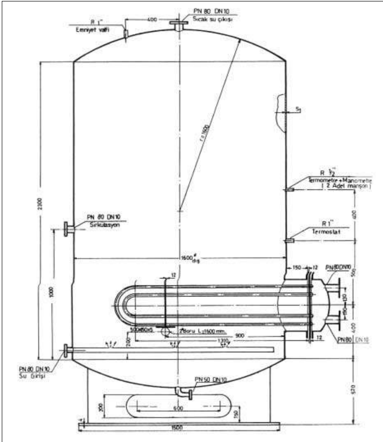
Şekil 5.80/ SERPANTİNLİ DİK BOYLER (5000 Litre)
