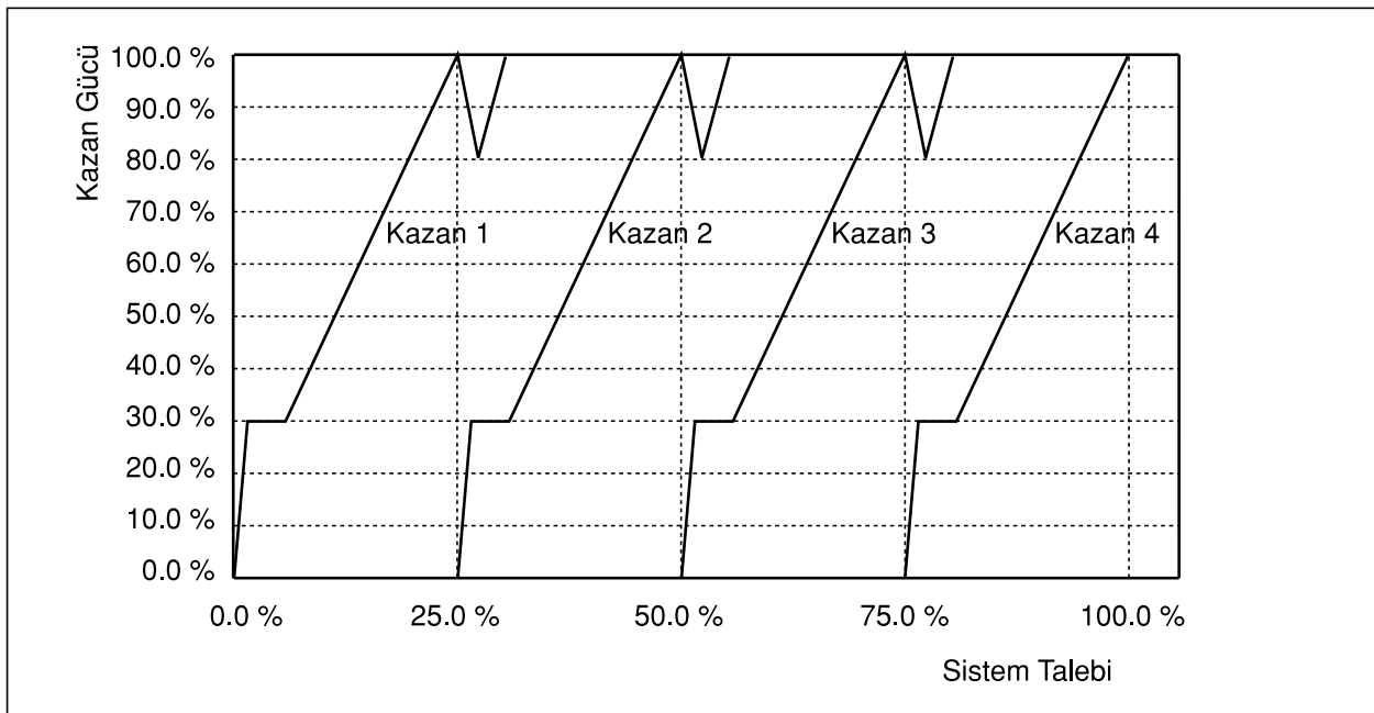
Şekil 5.40/ KAZANLARIN ISITMA DURUMUNDA DAVRANIŞLARI
