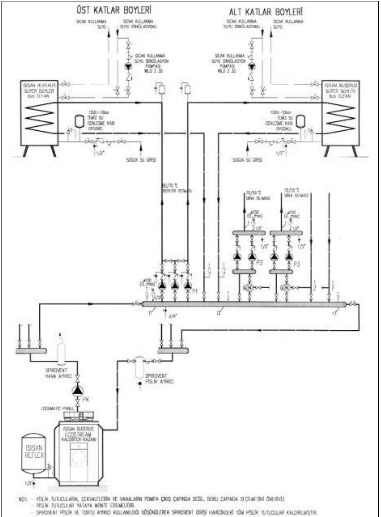
Şekil 4.30/ SİSTEM - 2
