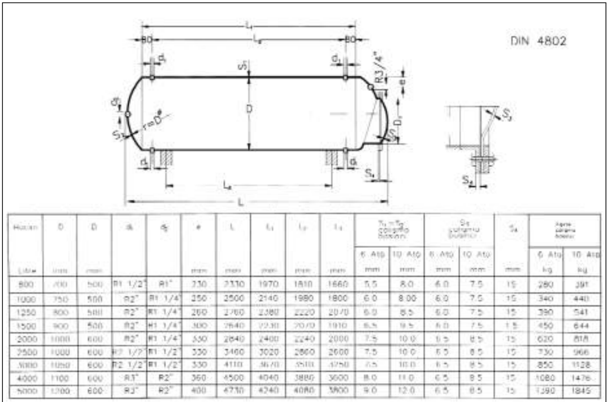
Şekil 5.79/ TEK ÇİDARLI BOYLER (Serpantin eklenecek)
