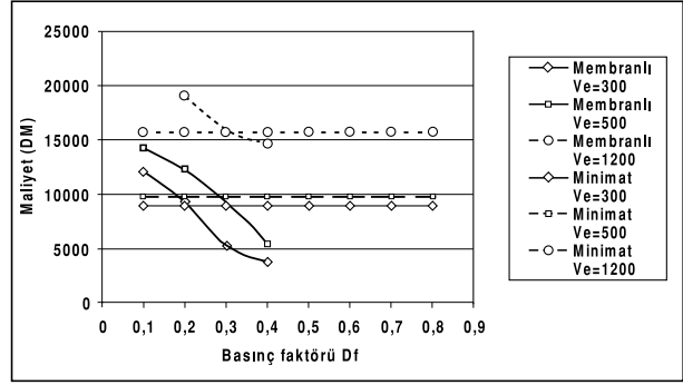
Şekil 6.39/ STATİK BASINÇ Pst=5 bar OLMASI HALİNDE MEMBRANLI - MİNİMAT KARŞILAŞTIRILMASI
