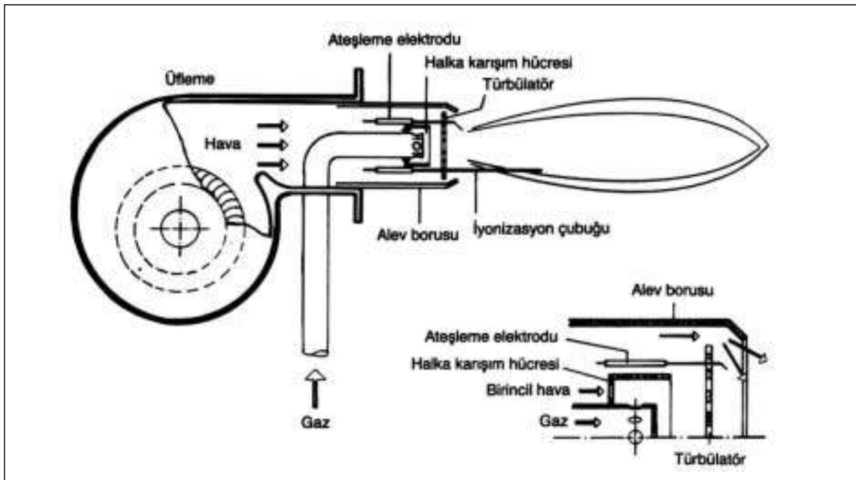
Şekil 5.67/ ÜFLEMELİ GAZ YAKICI BRÜLÖRÜ
