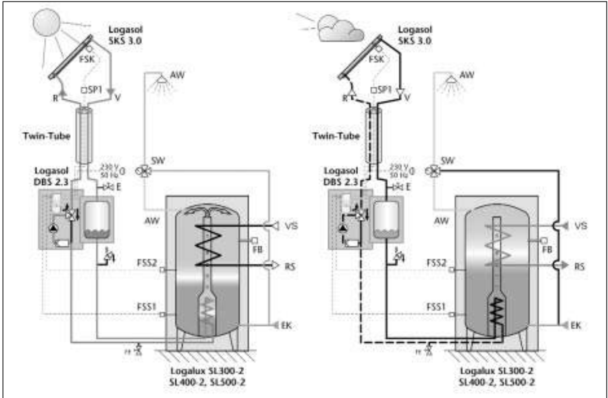
Şekil 4.43 / LOGASOL DBS 2.3 KUMANDA PANELİNİN KULLANILDIĞI, GERİ TOPLAMA SİSTEMİNİN İŞLETME VE BEKLEMEDE FONKSİYON PRENSİP ŞEMASI
