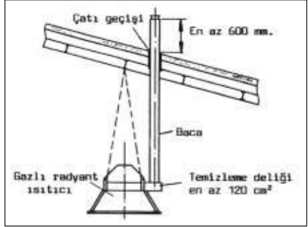
Şekil 6.21/ ÇATIDAN EGZOST GAZI AKIMI
