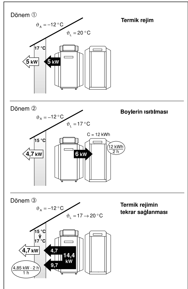
Şekil 3.16 / SU ISITILMASI VE BİNA ISINMASI İLE İLGİLİ FONKSİYONEL ADIMLAR VE ISI İHTİYACI DEĞERLERİ, BOYLERİN 2 SAAT ISITILMASINDA
