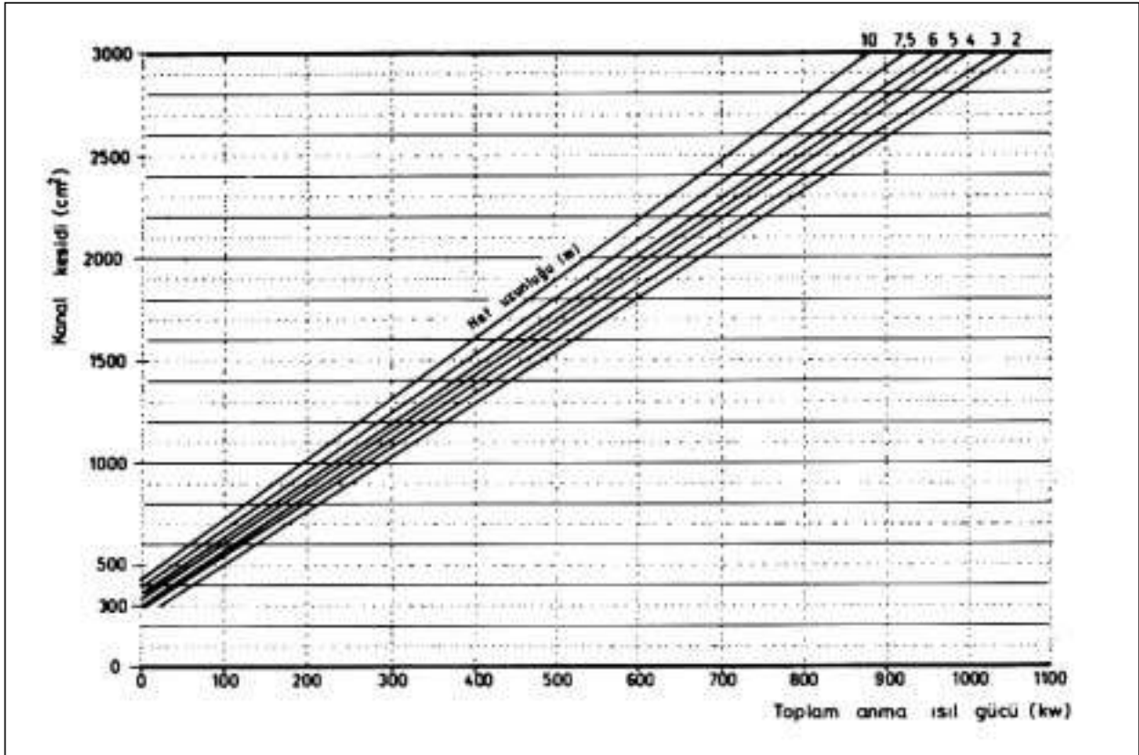
Şekil 9.3 / DAR KESİTLİ VE DÜZ HAVALANDIRMA KANALLARININ ÖLÇÜLERİ
