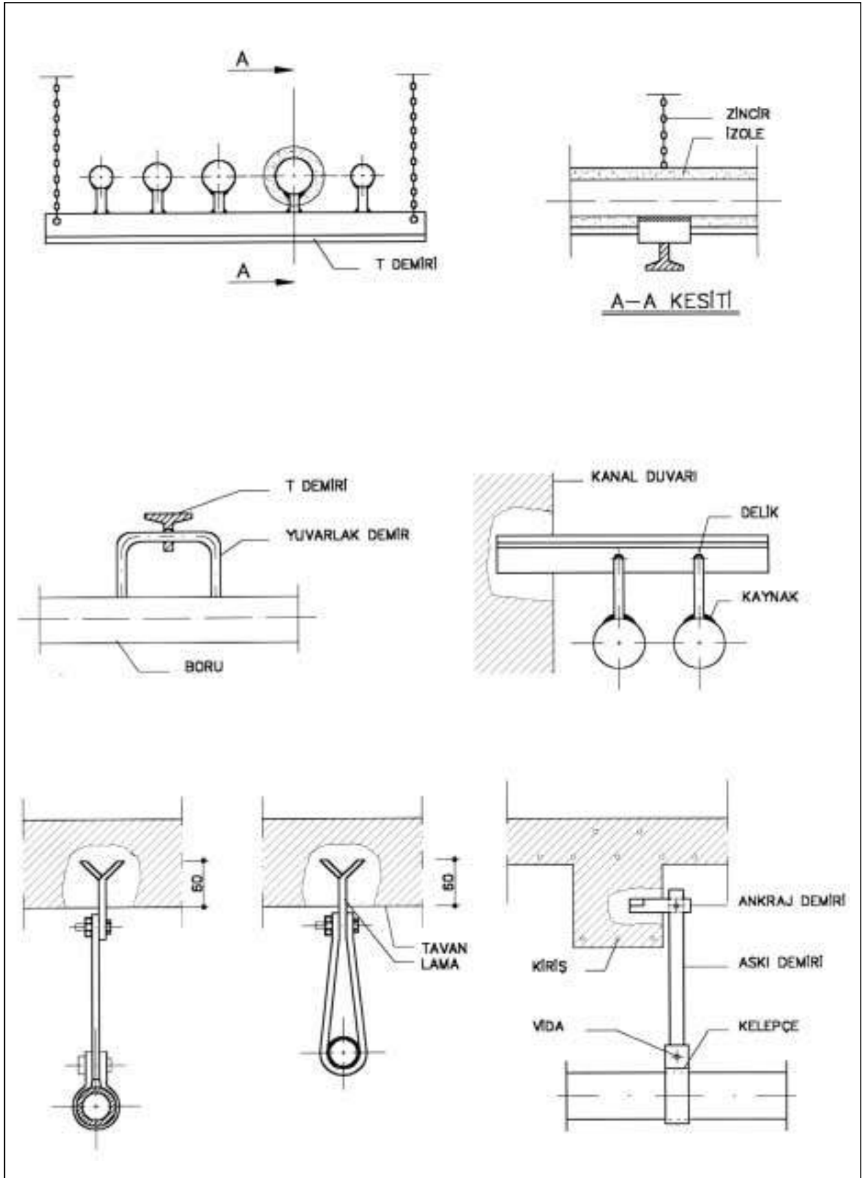
Şekil 7.15 / BORU ASKILARI
