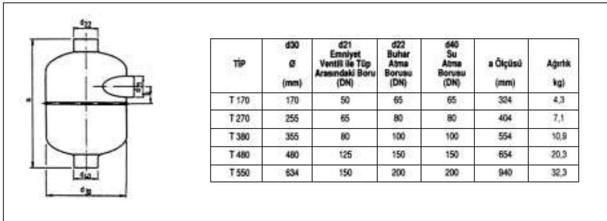
Şekil 6.48/ EMNİYET VENTİLLER ÇIKIŞINA MONTE EDİLECEK BOŞALTMA TÜPLERİNİN BOYUTLARI
