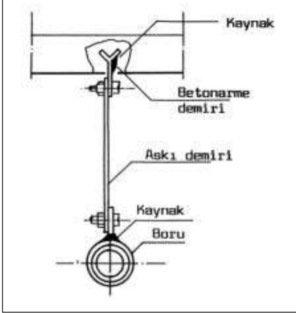
Şekil 7.16 / BETONARME DEMİRİNE KAYNAKLI ASKI
