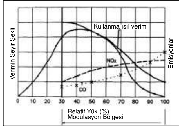
Şekil 5.26/ BÜYÜK BİR MODÜLASYON BÖLGESİ NEDEN ÖNEMLİDİR?
