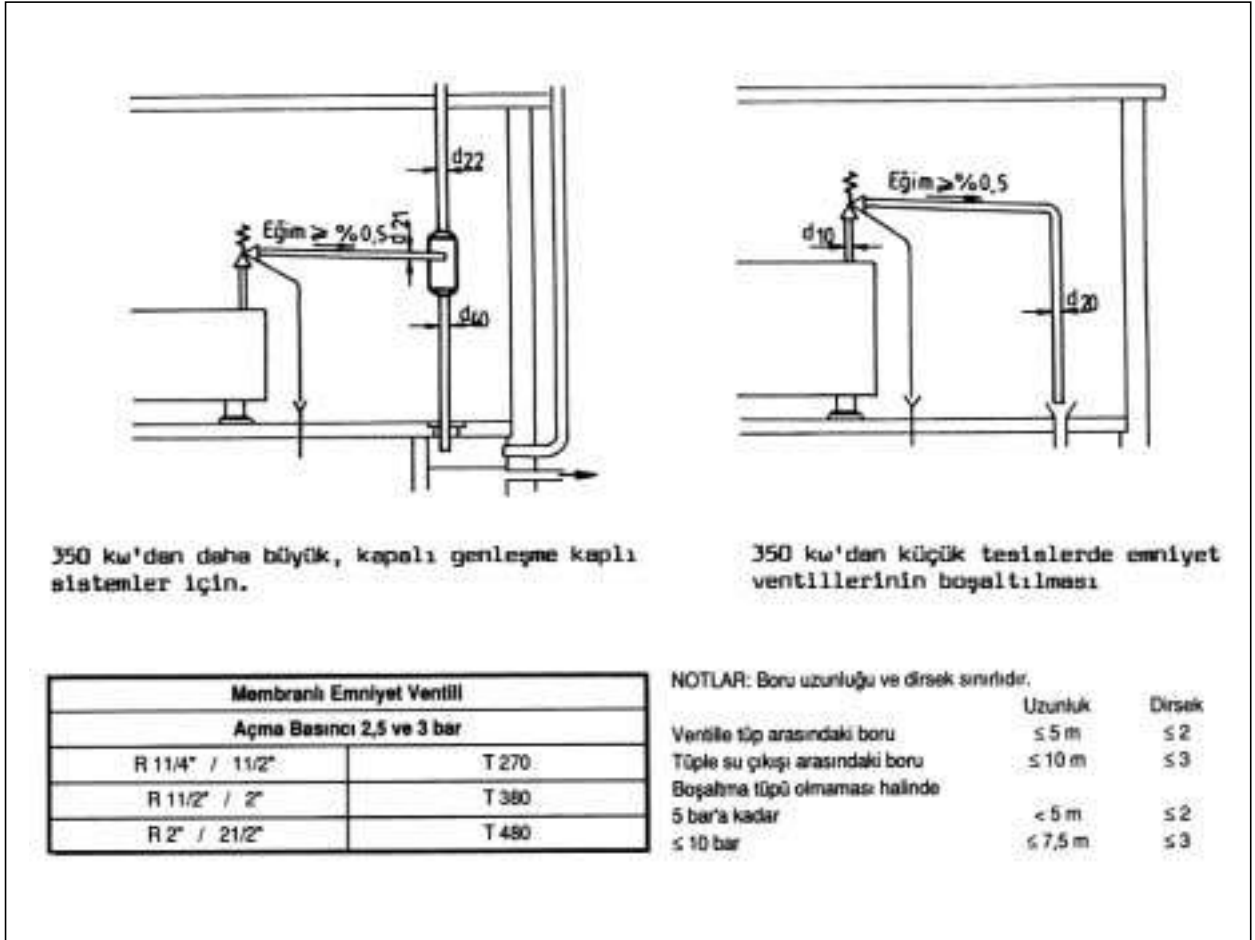
Şekil 6.47/ DIN 4751 KISIM 4'E GÖRE BOŞALTIMA TÜPLÜ TAHLİYE TESİS (Emniyet ventilleri için)
