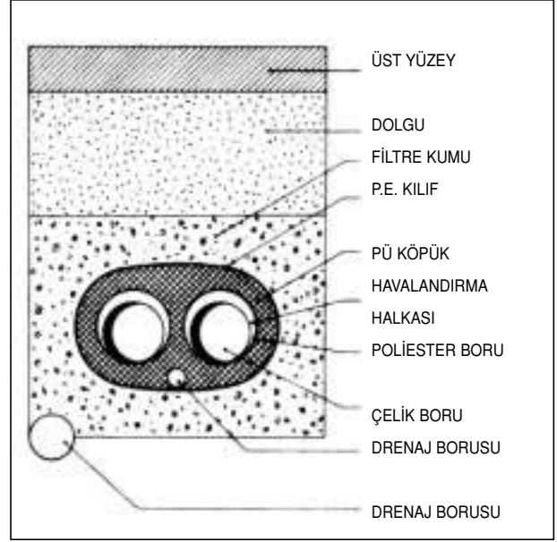
Şekil 4.23 / HAZIR PLASTİK BORU
