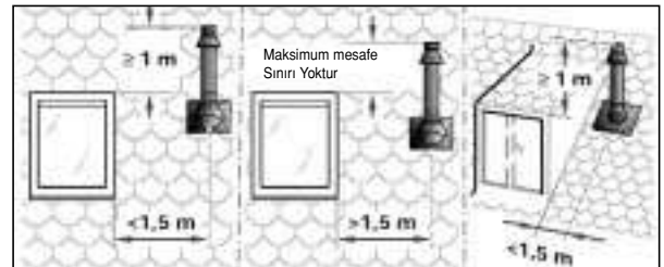
Şekil 10.34 / GB112-60 İÇİN BACA ÇIKIŞ KOŞULLARI
