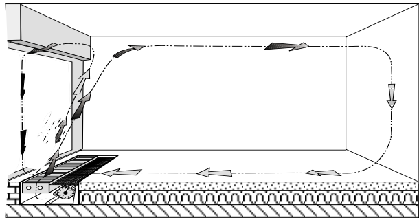
Şekil 6.9/ DOĞAL VE CEBRİ ÇEKİŞLİ DÖŞEME TİPİ KONVEKTÖR ŞEMASI
