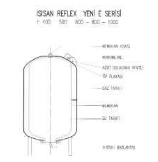
Şekil 6.30b/ ISISAN REFLEX YENİ E SERİSİ
