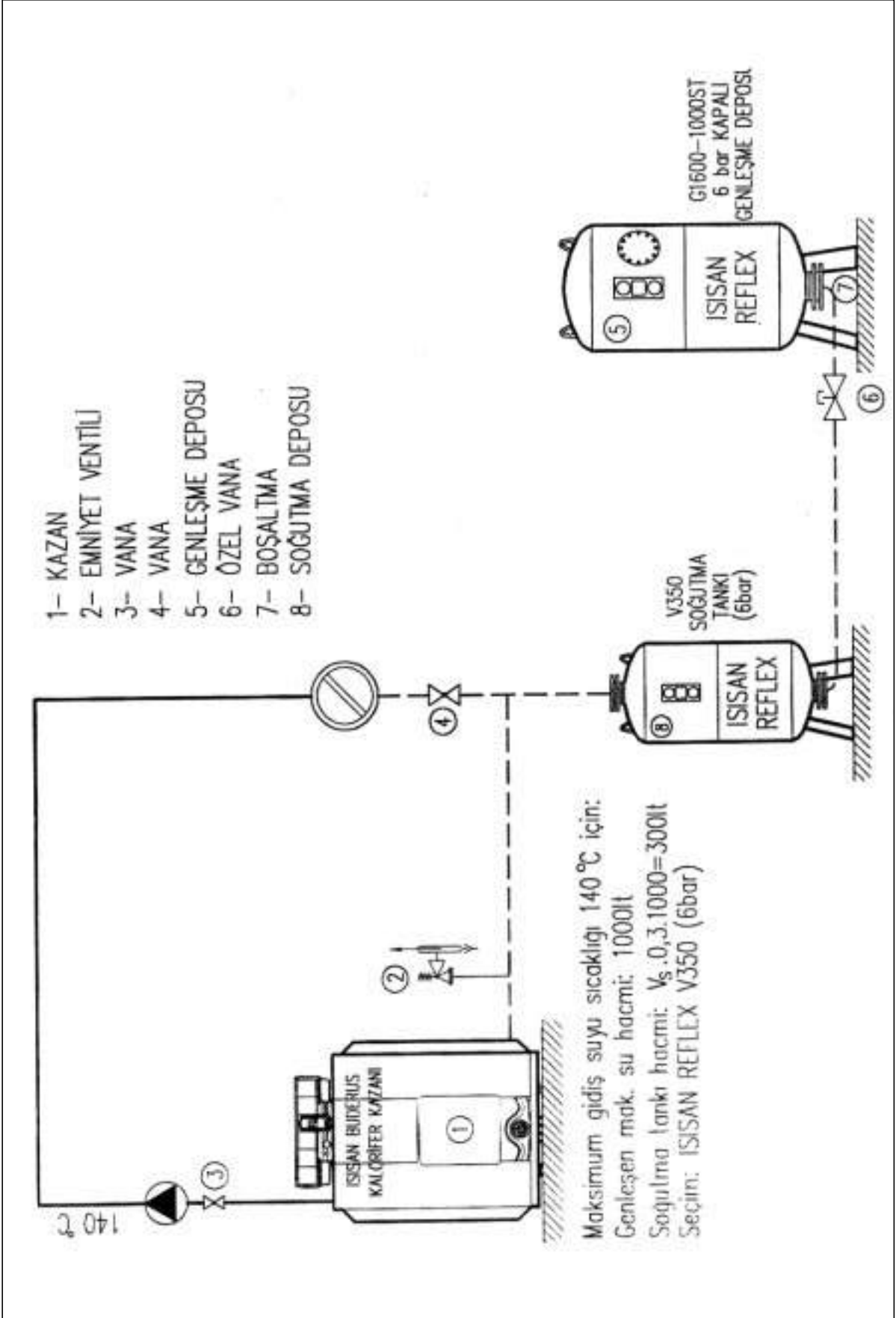
Şekil 4.34/ MEMBRANLI KAPALI GENLEŞME DEPOLU KAYNAR SU SİTEMİ TESİSAT ŞEMASI
