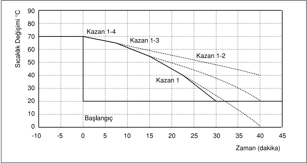
Şekil 5.41/ KASKAD SİSTEMİNİN KAPANMA DAVRANIŞI
