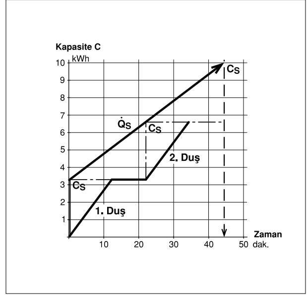
Şekil 3.22 / DUŞ BANYOSUNDAKİ İHTİYAÇ DURUMU, ÖRNEK 1.2'YE GÖRE
