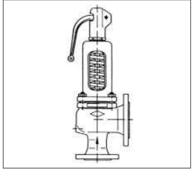
Şekil 7.55 / EMNİYET VENTİLİ
