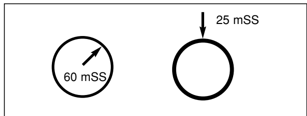
Şekil 5.75/ ÇİFT CİDARLI BOYLERLERDE MAX. KALORİFER BASINCI
