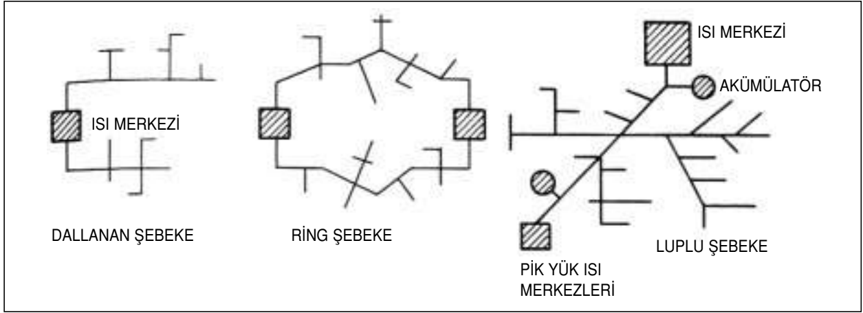
Şekil 4.17 / ÇEŞİTLİ ISITMA ŞEBEKESİ TİPLERİ
