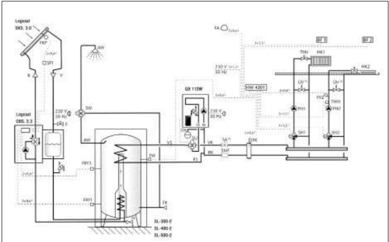
Şekil 4.49 / DUVAR TİPİ KAZANLA TAKVİYELİ GÜNEŞ ENERJİSİYLE KULLANMA SICAK SUYU ISITMA SİSTEMİ
