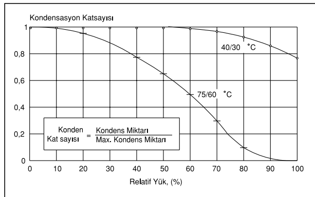
Şekil 5.28/ KONDENSASYON KATSAYISININ YÜKE BAĞLILIĞI
