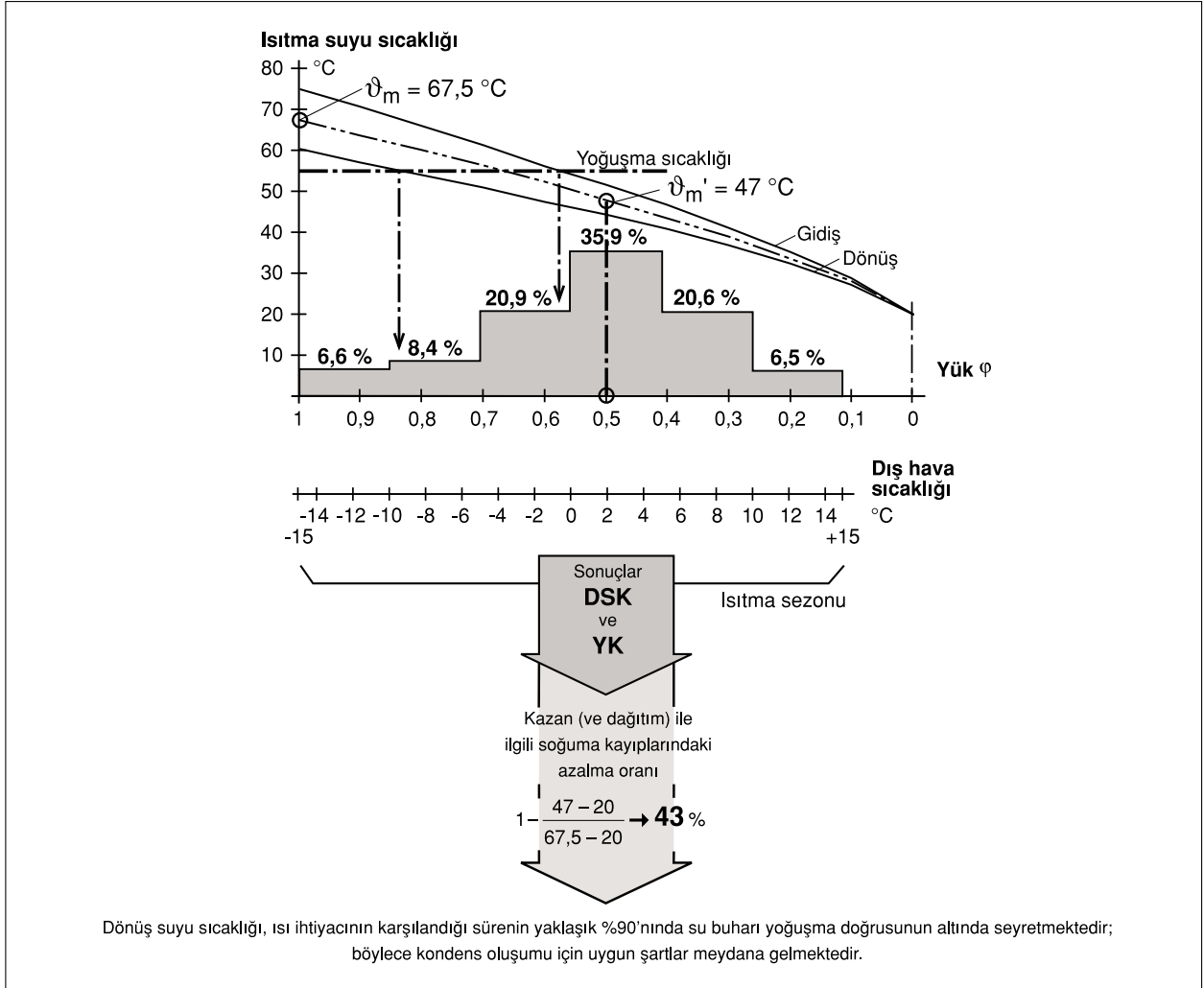
Şekil 3.29 / ISITMA EĞRİSİNİN SEYRİ SİSTEMİN İŞLETME ŞARTLARINI VE EKONOMİKLİĞİNİ ETKİLEMEKTEDİR.
