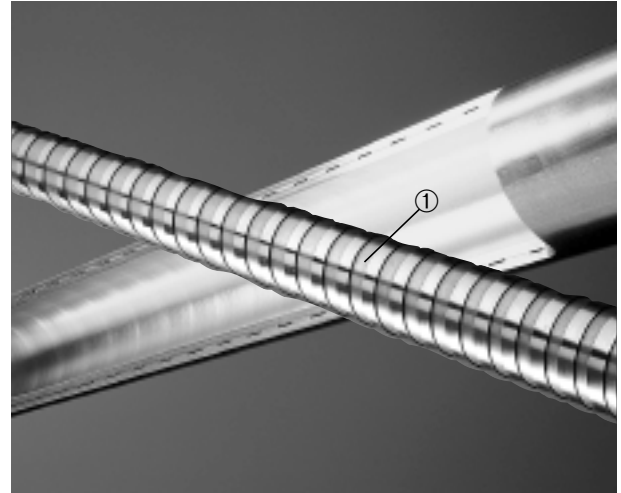
Şekil 3.37 / COMPOSIT - DUMAN GAZI BORUSUNUN YAPISI
