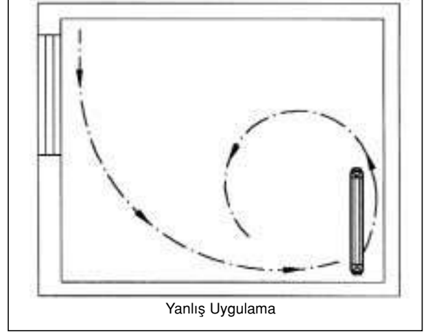
Şekil 2.5 / ODA HAVASI AKIMI RADYATÖRÜN DURDUĞU YERE BELİRLENİR
