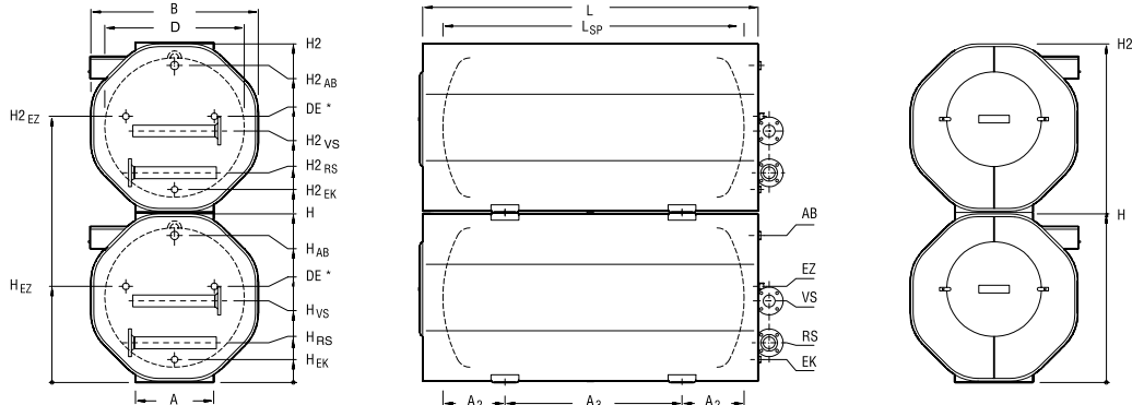
Şekil 5.84/ BUDERUS LOGALUX LT-L2T YATIK TİP duoCLEAN BOYLER
