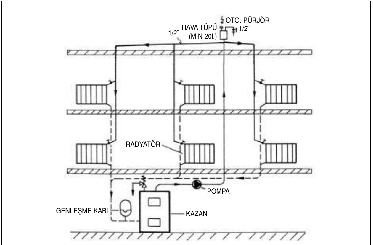
Şekil 4.9 / KAPALI GENLEŞME DEPOSU OLAN ÜSTTEN DAĞITMA, ALTTAN TOPLAMA SİSTEMİ
