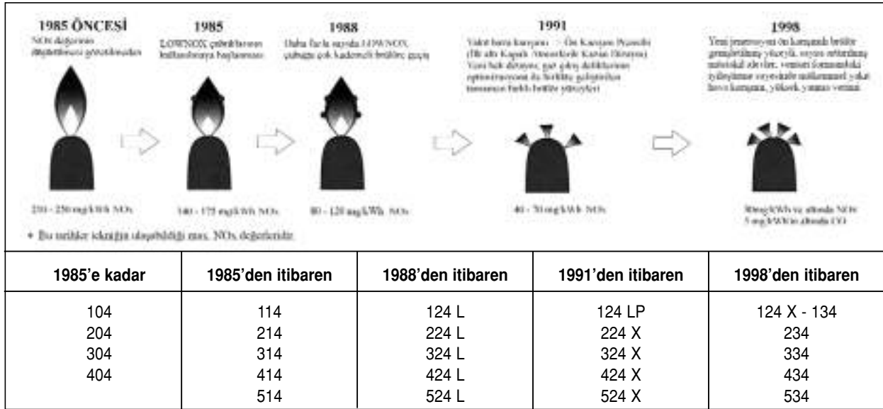
Şekil 5.66/ ISISAN BUDERUS ATMOSFERİK BRÜLÖRLÜ KAZANLAR İLE ÜFLEMELİ BRÜLÖRLÜ KAZANLARIN KARŞILAŞTIRILMASI (GAZ YAKITLI)
