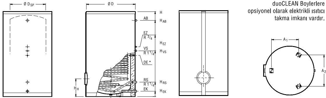
Şekil 5.83/ BUDERUS LOGALUX ST DİK TİP duoCLEAN BOYLER
