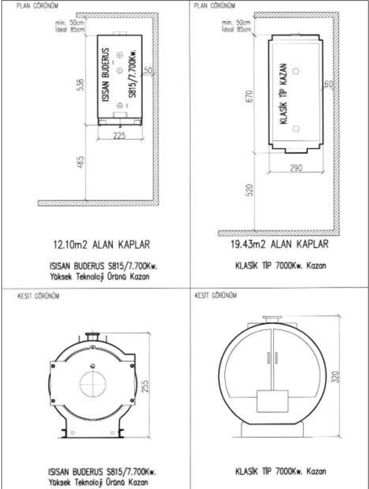
Şekil 9.1 / BUDERUS S815 ÇELİK SICAK SU KAZANLARI İLE EŞDEĞERİ KLASİK TİP ÇELİK KAZANIN, KAPLADIKLARI HACİM AÇISINDAN KARŞILAŞTIRMASI
