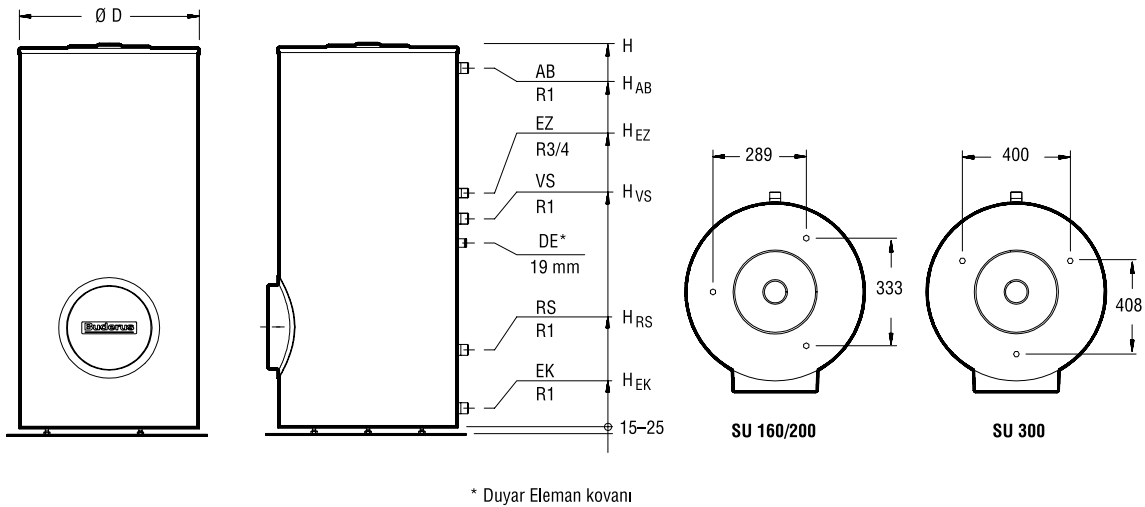
Şekil 5.85/ BUDERUS LOGALUX SU-SB DİK TİP duoCLEAN BOYLER
