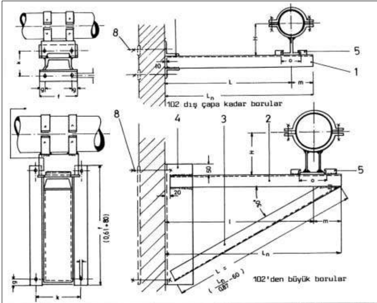
Şekil 7.9 / BORU KELEPÇESİ
