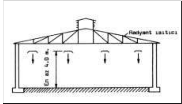
Şekil 6.23/ FABRİKA BİNASININ RADYANT ISITICILARLA ISITILMASI
