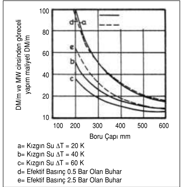
Şekil 4.16 / KIZGIN SU AĞININ GÖRECELİ MALİYETİ
