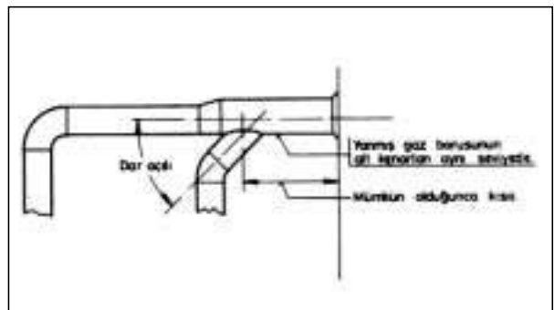
Şekil 10.14 / ORTAK BACA BAĞLANTISI
