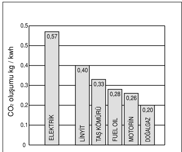
Şekil 11.31 / ÇEŞİTLİ ENERJİ KAYNAKLARININ SPESİFİK CO 2 EMİSYONLARI
