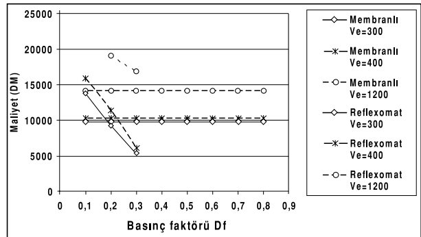
Şekil 6.40/ STATİK BASINÇ Pst=6 bar OLMASI HALİNDE MALİYET KARŞILAŞTIRILMASI
