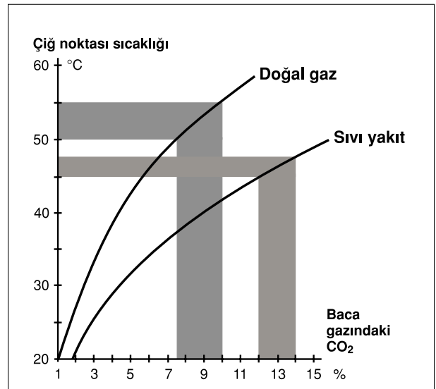
Şekil 3.31 / SU BUHARI ÇİĞ NOKTASI SICAKLIĞININ BACA GAZINDAKİ CO 2 MİKTARINA BAĞLILIĞI
