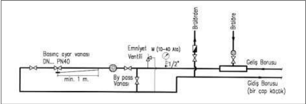
Şekil 5.63/ YAKIT RİNG HATTI SONU 3500 RW/sn FUEL ÖİL KULLANILDIĞINDA RİNG HATTI SONUNDA BASINÇ REGÜLATÖRÜ 25 ATÜ DEĞERE AYARLANIR.
