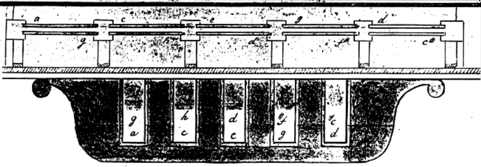
Zeichnung des Instrumentes des Secunden.
