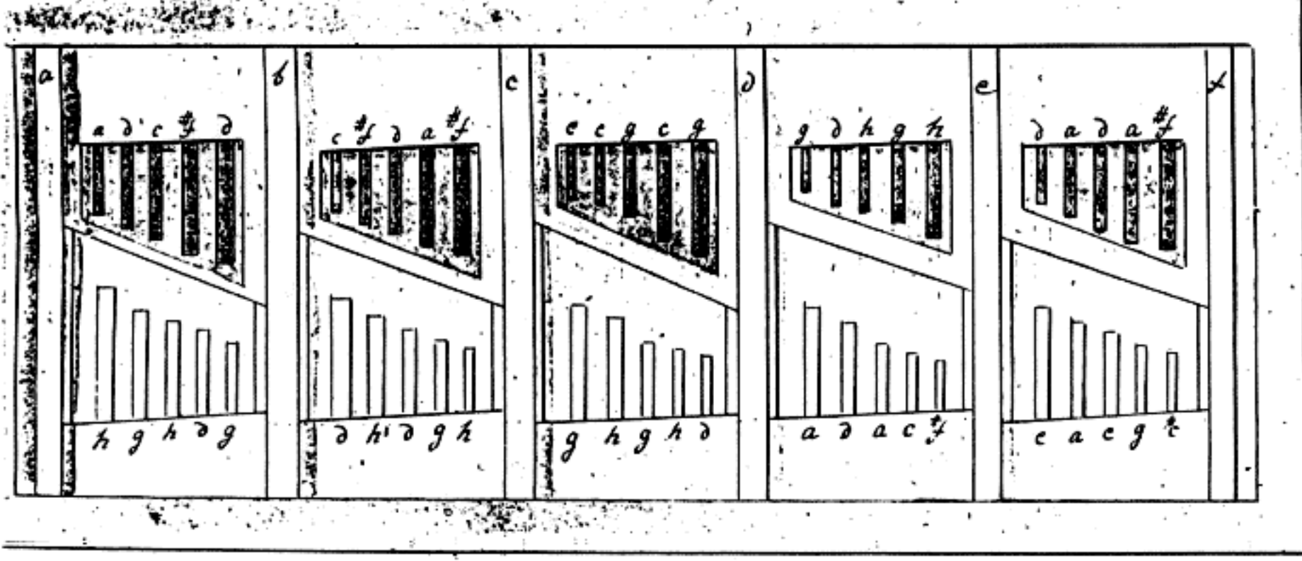
Zeichnung des Instrumentes des Secunden.
