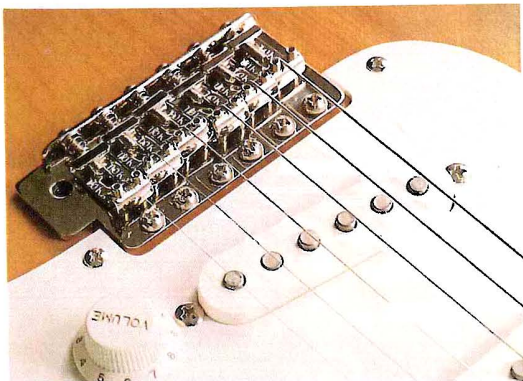
ST80・GSブリッジ&ピックアップ(STヴィンテージ)
