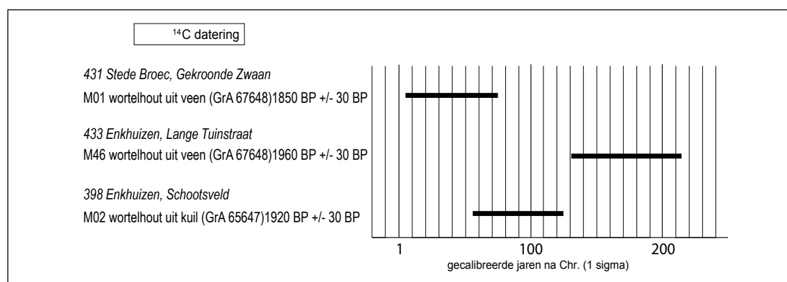
Afb. 4.3. De koolstof datering ( ^{14}\text{C} ) van het wortelhout van grove den ( Pinus sylvestris ) afkomstig van verschillende opgravingen binnen oostelijk West-Friesland. Deze boomsoort groeide in de eerste eeuwen van onze jaartelling binnen de regio.
