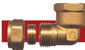
RACOR CODO HEMBRA JOELHO FÊMEA COUDE FEMELLE
