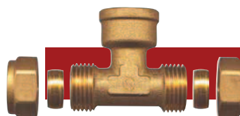
RACOR EN T HEMBRA TÊ FÊMEA RACCORD EN TE FEMELLE
